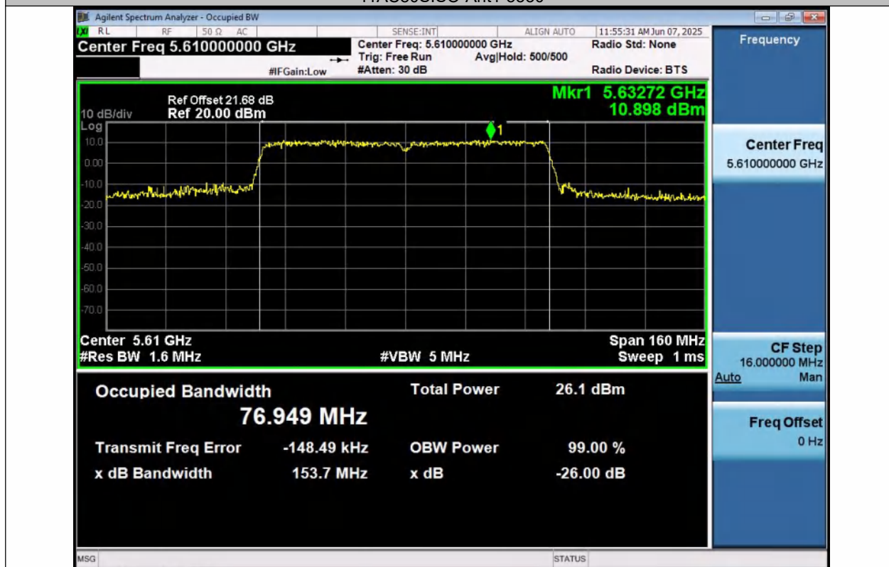
11AC80SISO-Ant1-5610
