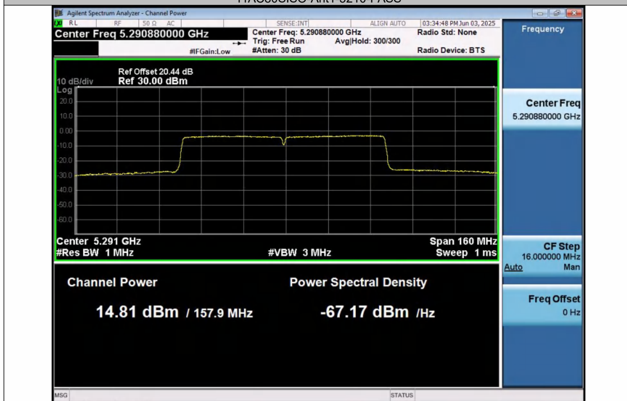
11AC80SISO-Ant1-5290-PASS
