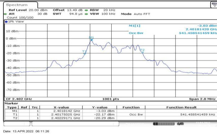
250K_Ant1_2402
