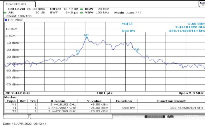
250K_Ant1_2442
