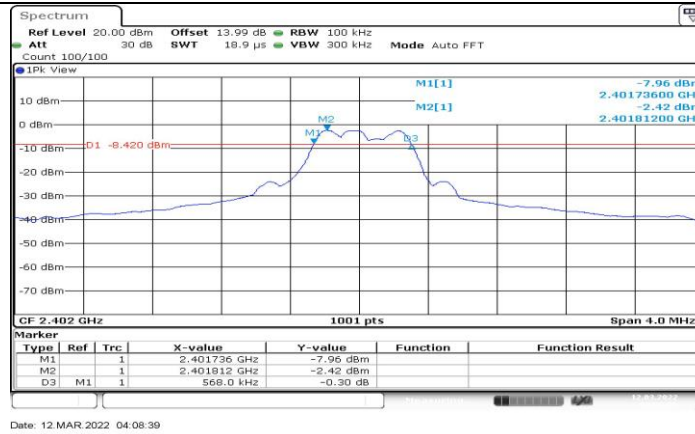
250K_Ant1_2402
