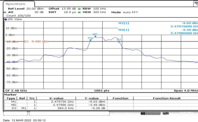
250K_Ant1_2480
