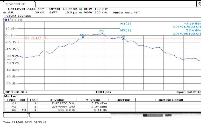
2M_Ant1_2480
