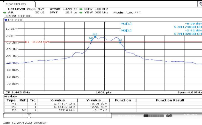
250K_Ant1_2442
