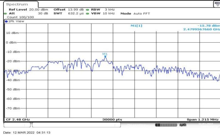
2M_Ant1_2480
