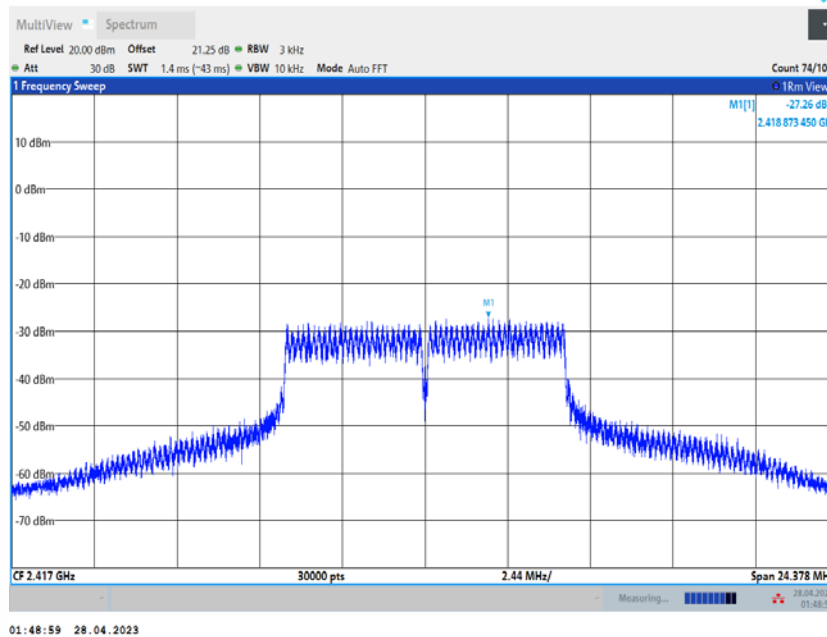
11G_Ant1_2417
