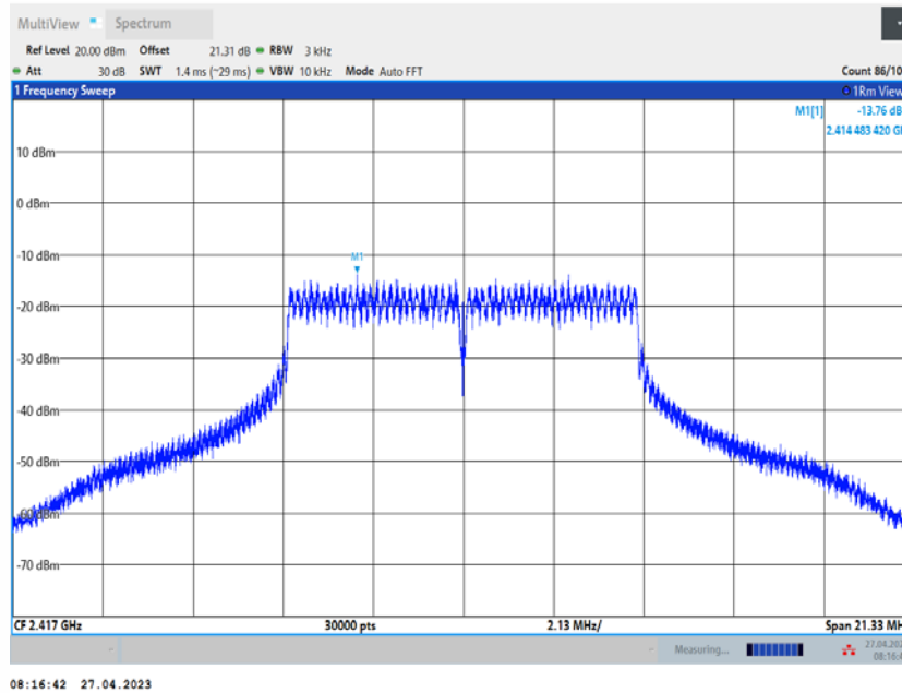
11B_Ant2_2417
