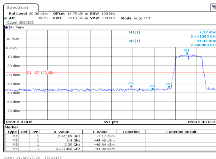
11G_Ant1_Low_2412
