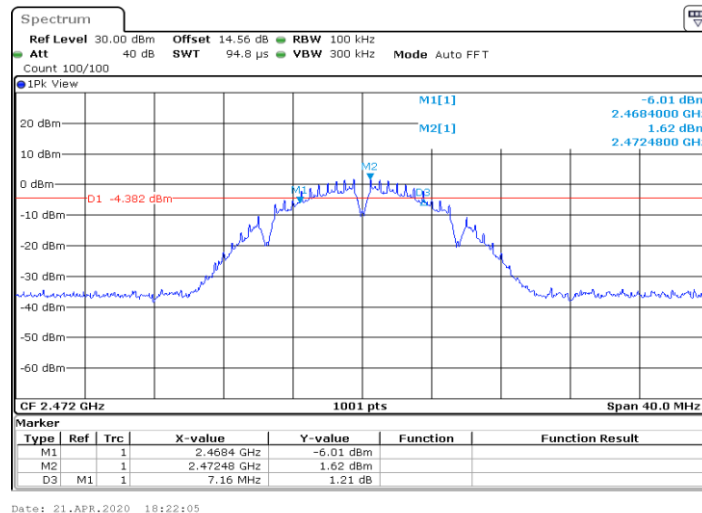
11B_Ant1_2472
