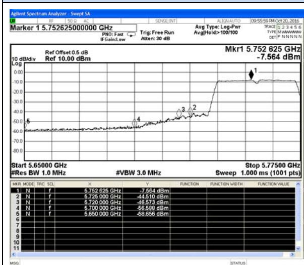
802.11n40-5755MHz-Lower(Peak)
