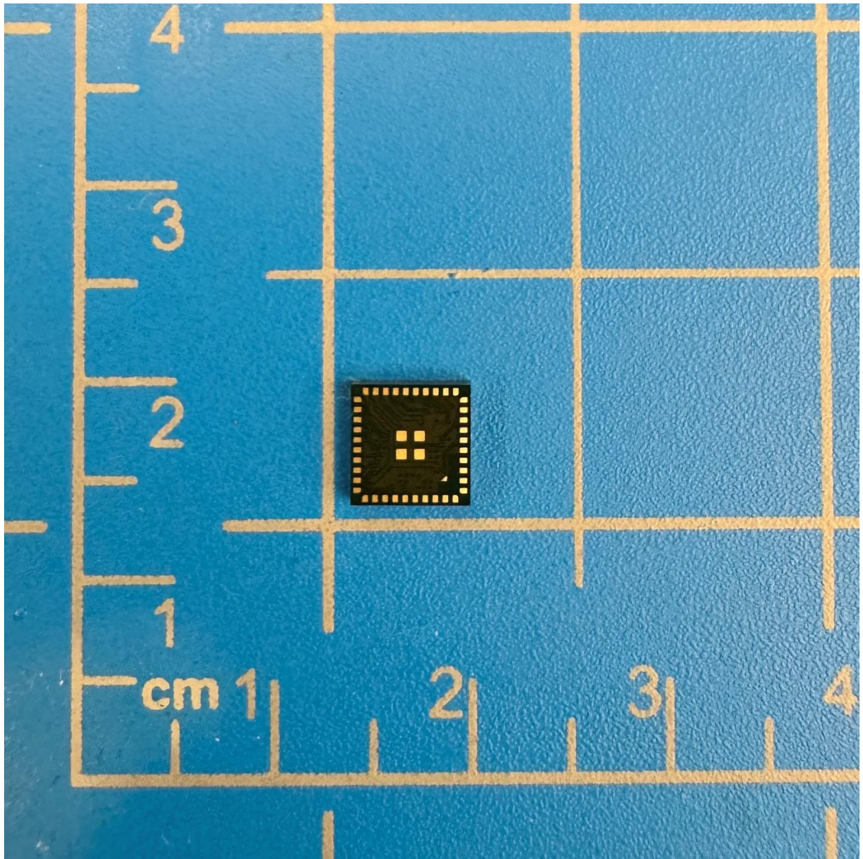
Figure 2. Lyra-S BLE module (bottom)
