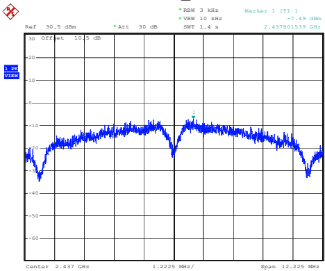
802.11b_2437MHz
