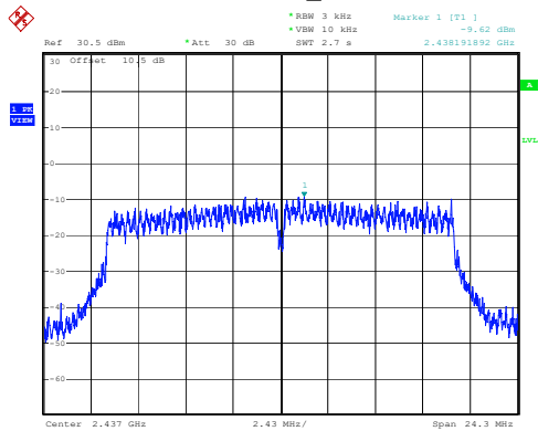
802.11n20_2437MHz
