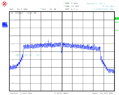
802.11n20_2462MHz
