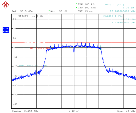
802.11n20_2437MHz
