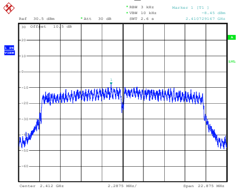
802.11n20_2412MHz
