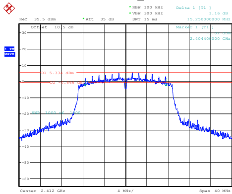
802.11n20_2412MHz
