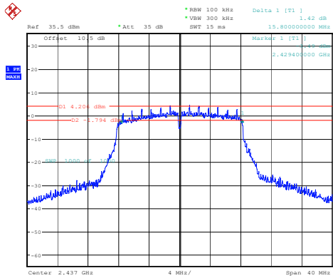
802.11g_2437MHz
