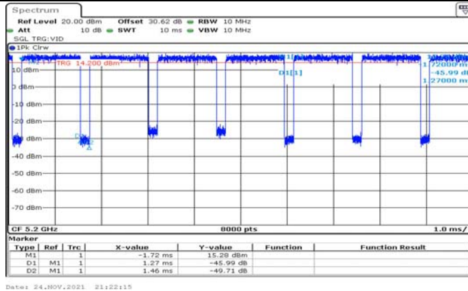
11N20SISO Ant1 5200
