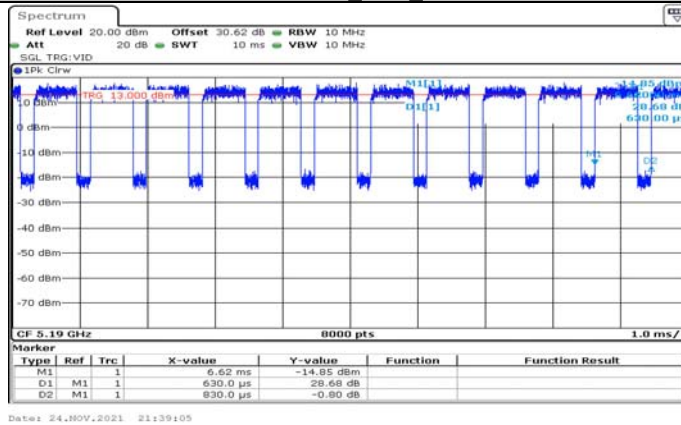
11N40SISO Ant1 5190
