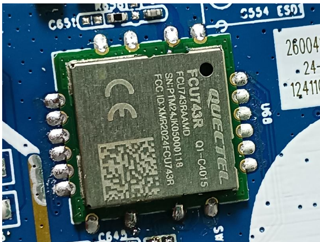
Wi-Fi Module
