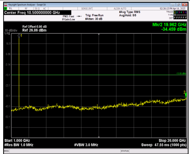
Band25-1.4MHz-QPSK-26365-1RB#0-Range2:1000~20000MHz
