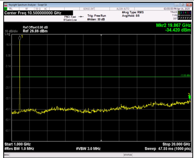
Band25-20MHz-QPSK-26590-1RB#0-Range2:1000~20000MHz
