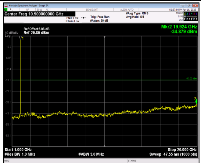
Band25-1.4MHz-QPSK-26683-1RB#0-Range2:1000~20000MHz
