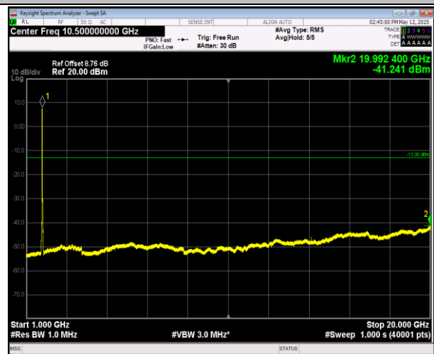
66-66-20MHz-20MHz-QPSK-QPSK-132374-132572-1RB#0 -ORB#0-1000~20000MHz-PASS
