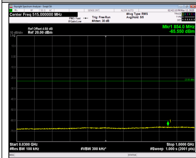
66-66-20MHz-20MHz-16QAM-16QAM-132323-132521-1 00RB#0-100RB#0-30~1000MHz-PASS
