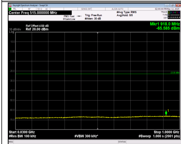
66-66-20MHz-20MHz-QPSK-QPSK-132374-132572-1RB #0-ORB#0-30~1000MHz-PASS
