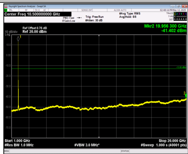
66-66-20MHz-20MHz-QPSK-QPSK-132374-132572-1RB#9 9-0RB#0-1000~20000MHz-PASS
