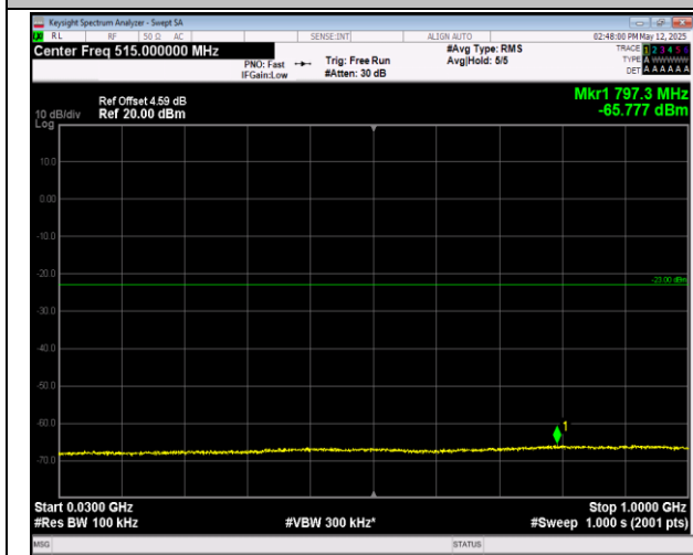
66-66-20MHz-20MHz-QPSK-QPSK-132374-132572-1RB #99-0RB#0-30~1000MHz-PASS
