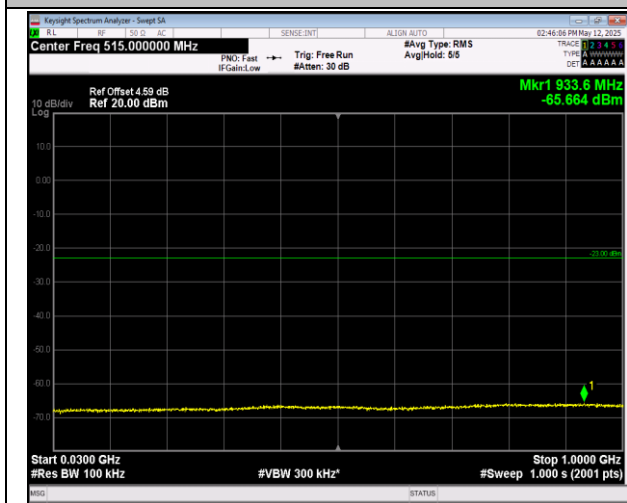
66-66-20MHz-20MHz-16QAM-16QAM-132374-132572-1 RB#0-1RB#99-30~1000MHz-PASS
