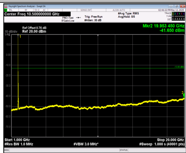
66-66-20MHz-20MHz-16QAM-16QAM-132374-132572-1RB #0-1RB#99-1000~20000MHz-PASS
