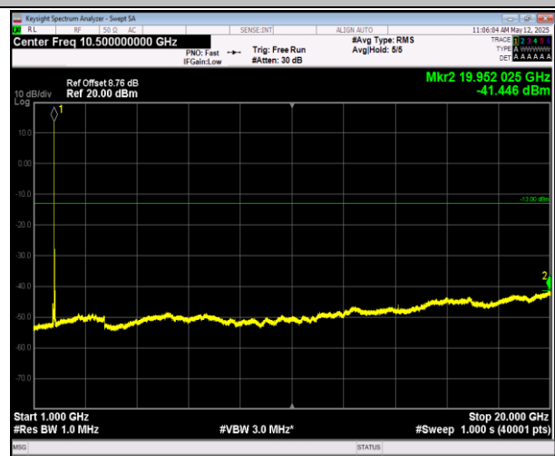
66-66-20MHz-5MHz-QPSK-QPSK-132522-132639-1RB#99 -0RB#0-1000~20000MHz-PASS
