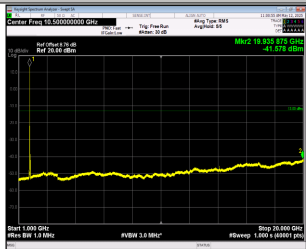
66-66-20MHz-5MHz-QPSK-QPSK-132397-132514-1RB#99 -ORB#0-1000~20000MHz-PASS
