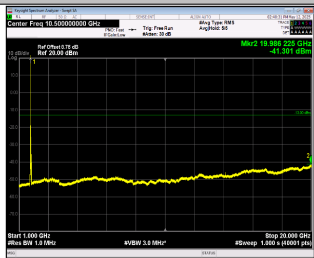
66-66-20MHz-20MHz-QPSK-QPSK-132323-132521-1RB#0 -1RB#99-1000~20000MHz-PASS
