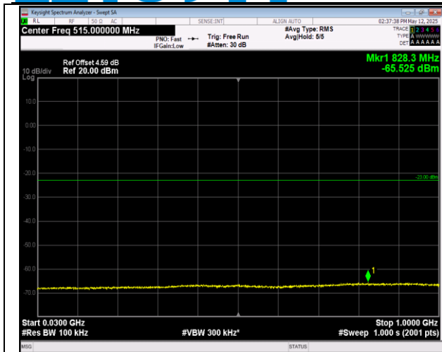
66-66-20MHz-20MHz-QPSK-QPSK-132072-132270-1RB #99-ORB#0-30~1000MHz-PASS
