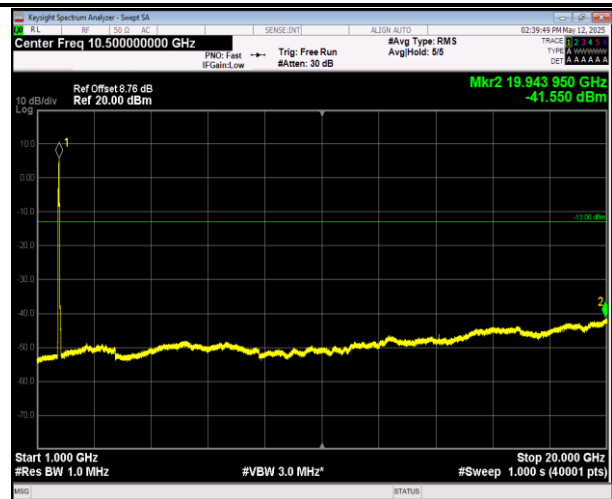
66-66-20MHz-20MHz-QPSK-QPSK-132323-132521-1RB#0 -ORB#0-1000~20000MHz-PASS
