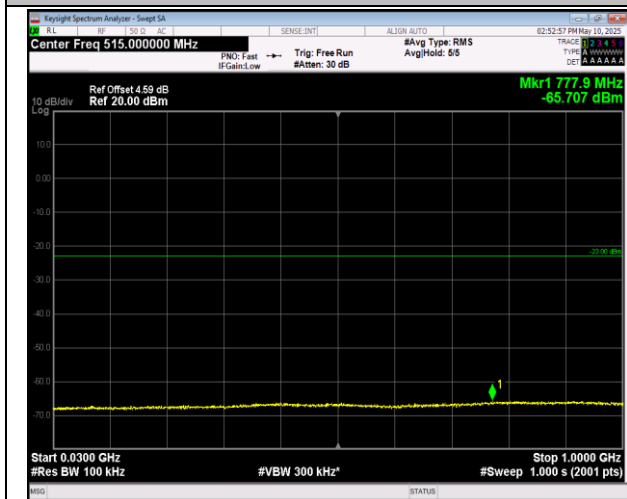
66-66-5MHz-20MHz-QPSK-QPSK-132455-132572-25RB #0-100RB#0-30-1000MHz-PASS
