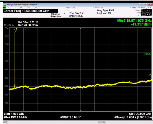
66-66-20MHz-20MHz-QPSK-QPSK-132323-132521-1RB#9 9-ORB#0-1000~20000MHz-PASS
