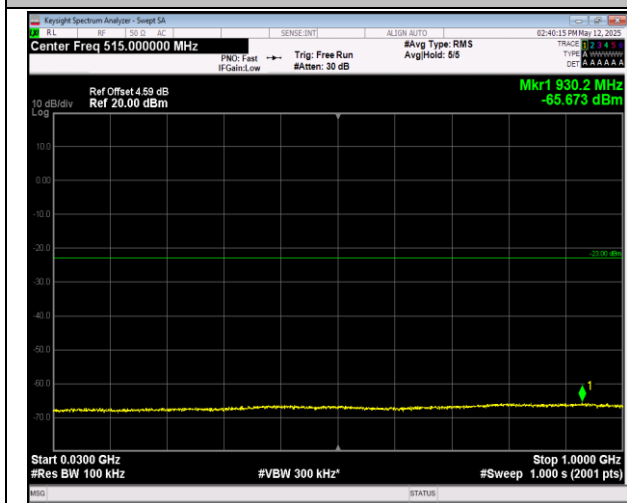
66-66-20MHz-20MHz-QPSK-QPSK-132323-132521-1RB #0-1RB#99-30~1000MHz-PASS
