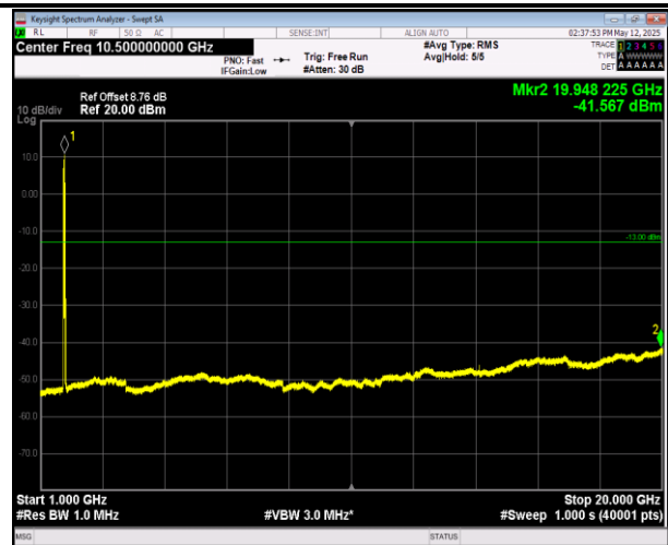
66-66-20MHz-20MHz-QPSK-QPSK-132072-132270-1RB#9 9-ORB#0-1000~20000MHz-PASS
