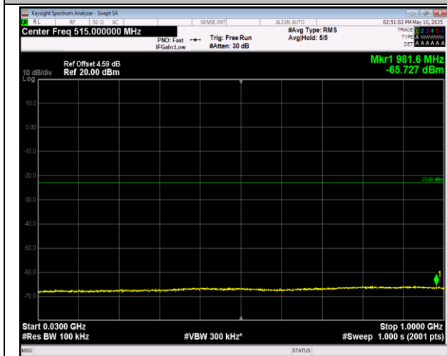
66-66-5MHz-20MHz-QPSK-QPSK-132455-132572-1RB# 0-ORB#0-30~1000MHz-PASS
