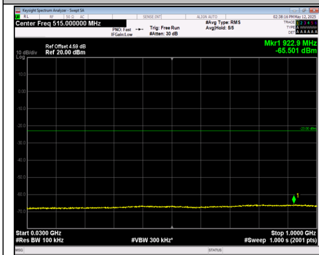
66-66-20MHz-20MHz-16QAM-16QAM-132072-132270-1 RB#99-0RB#0-30~1000MHz-PASS
