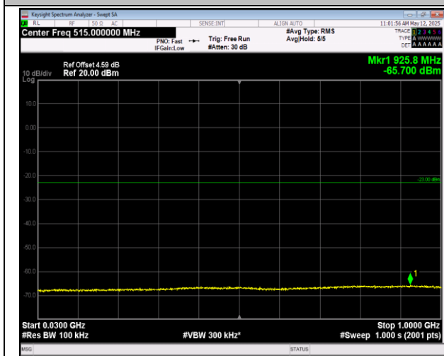
66-66-20MHz-5MHz-16QAM-16QAM-132397-132514-1R B#0-0RB#0-30~1000MHz-PASS
