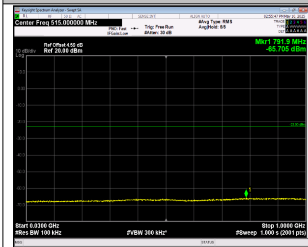
66-66-20MHz-5MHz-QPSK-QPSK-132072-132189-1RB# 0-0RB#0-30~1000MHz-PASS
