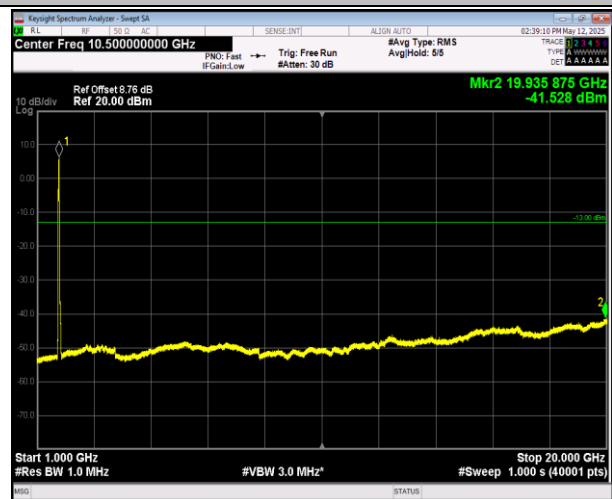
66-66-20MHz-20MHz-16QAM-16QAM-132072-132270-1RB #0-ORB#0-1000~20000MHz-PASS
