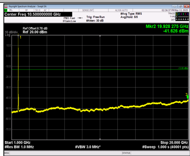
66-66-20MHz-20MHz-QPSK-QPSK-132072-132270-100RB #0-100RB#0-1000~20000MHz-PASS
