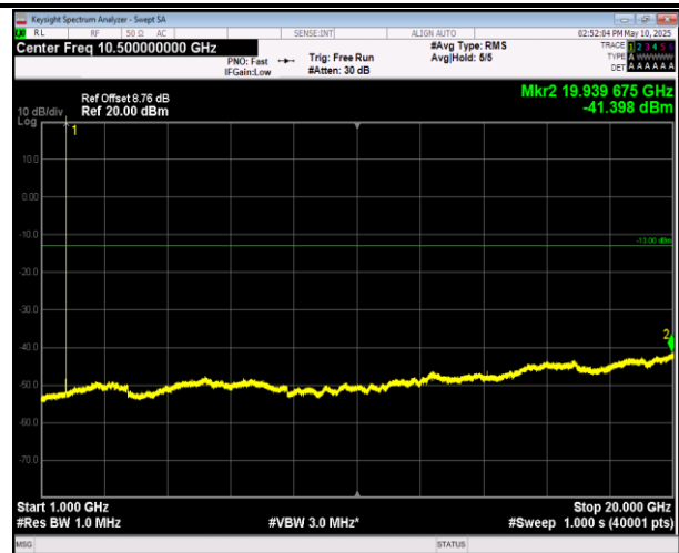
66-66-5MHz-20MHz-QPSK-QPSK-132455-132572-1RB#0- 1RB#99-1000-20000MHz-PASS
