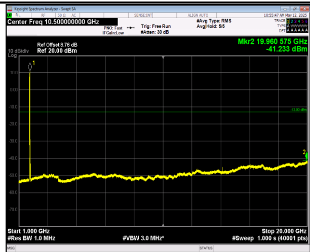
66-66-20MHz-5MHz-QPSK-QPSK-132072-132189-1RB#99 -ORB#0-1000~20000MHz-PASS
