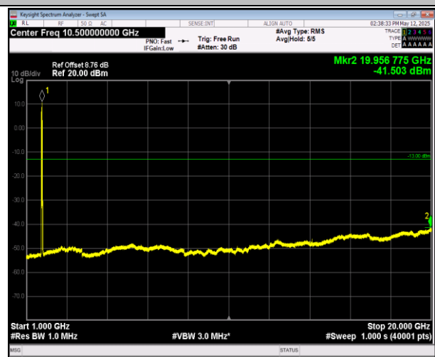
66-66-20MHz-20MHz-16QAM-16QAM-132072-132270-1RB #99-0RB#0-1000~20000MHz-PASS
