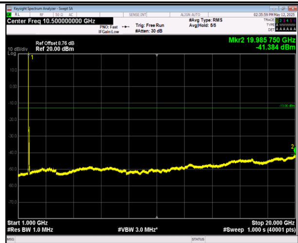
66-66-20MHz-20MHz-16QAM-16QAM-132072-132270-1RB #0-1RB#99-1000~20000MHz-PASS
