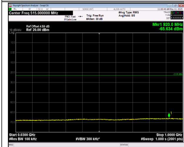
66-66-20MHz-5MHz-QPSK-QPSK-132397-132514-1RB# 99-ORB#0-30~1000MHz-PASS
