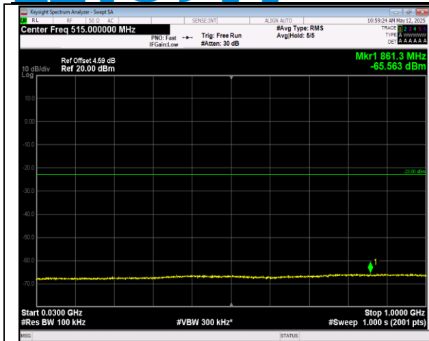
66-66-20MHz-5MHz-QPSK-QPSK-132397-132514-100R B#0-25RB#0-30~1000MHz-PASS
