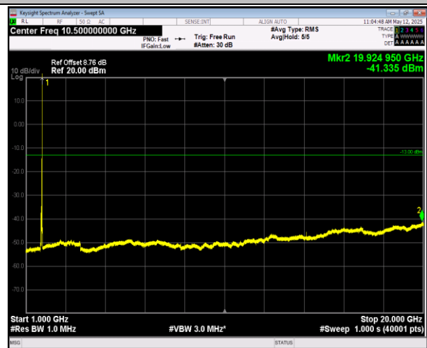
66-66-20MHz-5MHz-QPSK-QPSK-132522-132639-100RB# 0-25RB#0-1000~20000MHz-PASS
