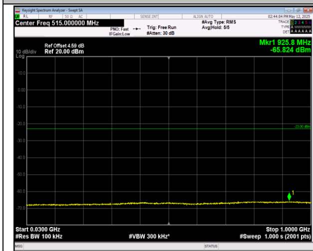
66-66-20MHz-20MHz-16QAM-16QAM-132323-132521-1 RB#0-0RB#0-30~1000MHz-PASS
