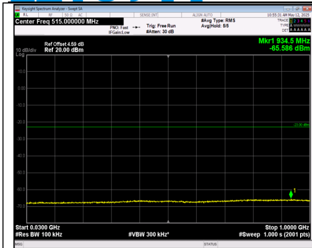
66-66-20MHz-5MHz-QPSK-QPSK-132072-132189-1RB# 99-ORB#0-30~1000MHz-PASS
