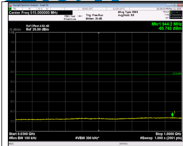
66-66-20MHz-20MHz-QPSK-QPSK-132323-132521-1RB #0-ORB#0-30~1000MHz-PASS
