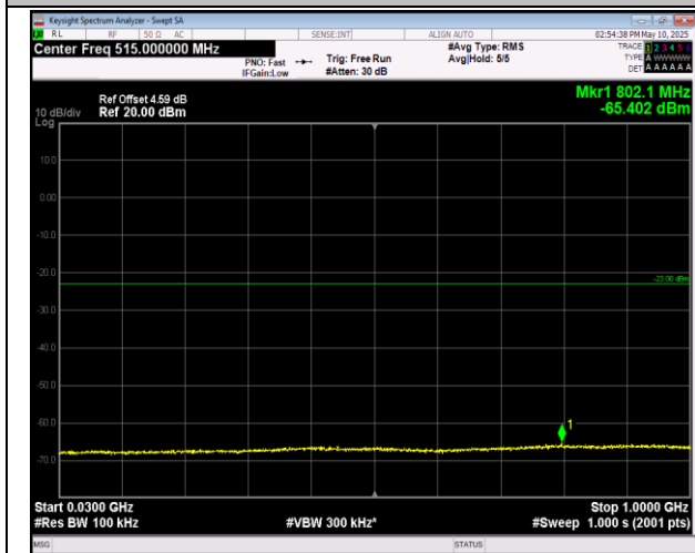
66-66-5MHz-20MHz-16QAM-16QAM-132455-132572-1R B#24-0RB#0-30~1000MHz-PASS
