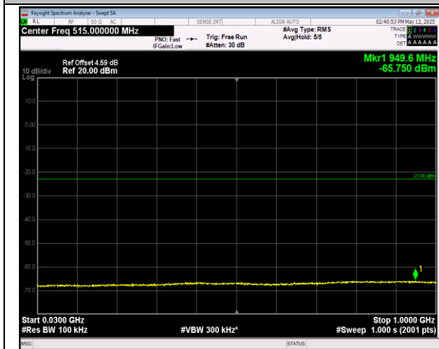
66-66-20MHz-20MHz-16QAM-16QAM-132323-132521-1 RB#0-1RB#99-30~1000MHz-PASS
