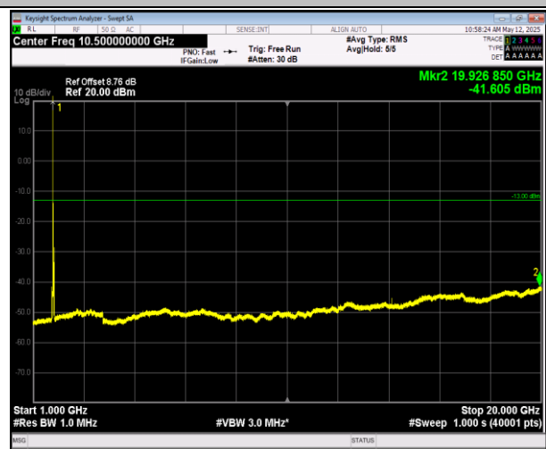
66-66-20MHz-5MHz-QPSK-QPSK-132397-132514-1RB#0- 1RB#24-1000~20000MHz-PASS
