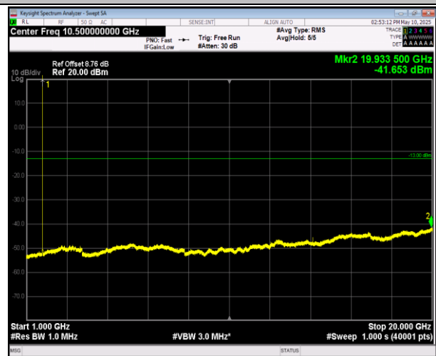
66-66-5MHz-20MHz-QPSK-QPSK-132455-132572-25RB#0 -100RB#0-1000-20000MHz-PASS
