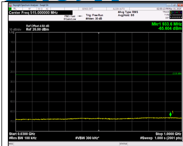
66-66-5MHz-20MHz-16QAM-16QAM-132455-132572-1R B#0-0RB#0-30~1000MHz-PASS
