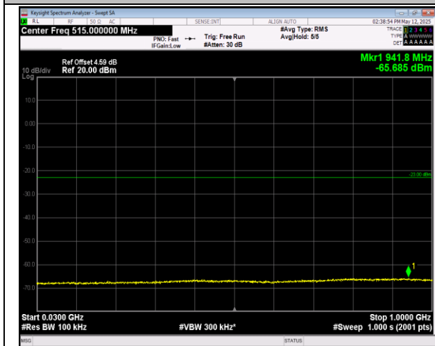
66-66-20MHz-20MHz-16QAM-16QAM-132072-132270-1RB RB#0-ORB#0-30~1000MHz-PASS
