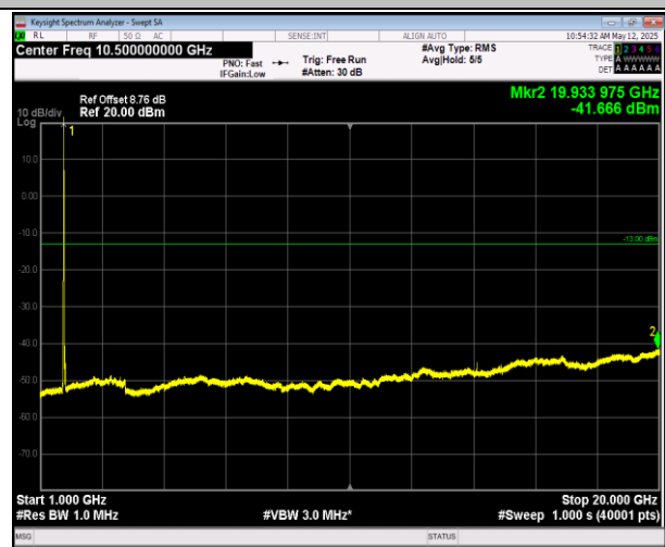
66-66-20MHz-5MHz-QPSK-QPSK-132072-132189-100RB# 0-25RB#0-1000~20000MHz-PASS
