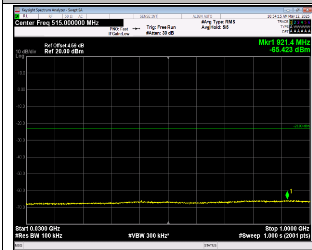
66-66-20MHz-5MHz-QPSK-QPSK-132072-132189-100RB# B#0-25RB#0-30~1000MHz-PASS
