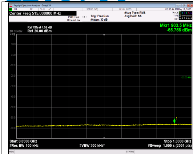
66-66-20MHz-20MHz-16QAM-16QAM-132072-132270-1 RB#0-1RB#99-30~1000MHz-PASS
