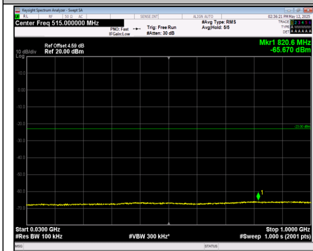
66-66-20MHz-20MHz-QPSK-QPSK-132072-132270-100RB RB#0-100RB#0-30~1000MHz-PASS
