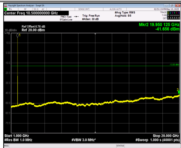
66-66-5MHz-20MHz-QPSK-QPSK-132455-132572-1RB#0- ORB#0-1000~20000MHz-PASS
