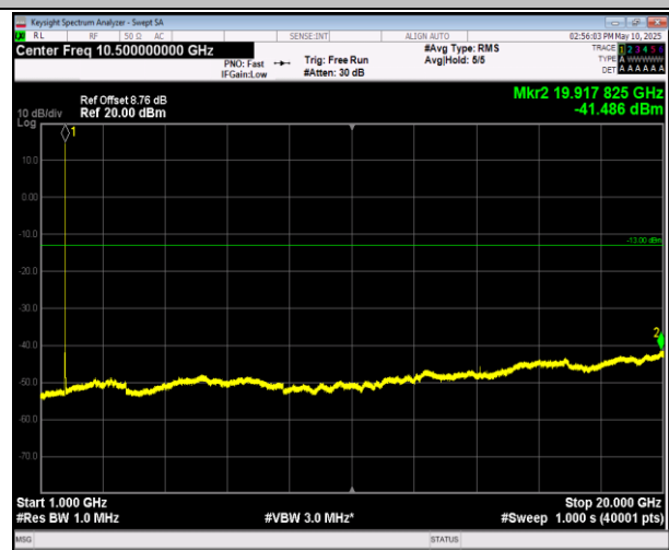
66-66-20MHz-5MHz-QPSK-QPSK-132072-132189-1RB#0- 0RB#0-1000~20000MHz-PASS
