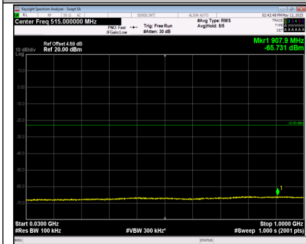
66-66-20MHz-20MHz-QPSK-QPSK-132323-132521-1RB #99-ORB#0-30~1000MHz-PASS
