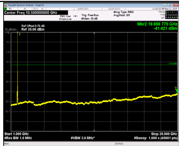
66-66-20MHz-5MHz-QPSK-QPSK-132522-132639-1RB#0- 1RB#24-1000~20000MHz-PASS
