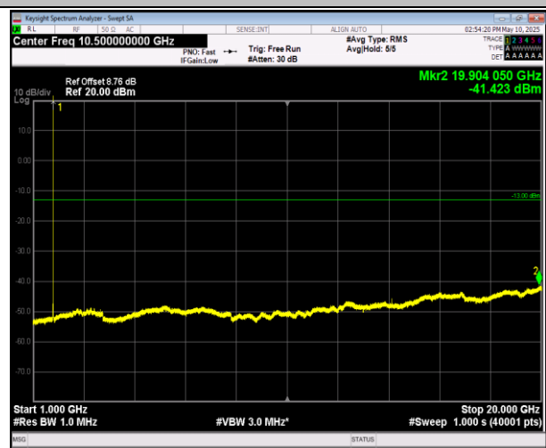
66-66-5MHz-20MHz-QPSK-QPSK-132455-132572-1RB#24 -0RB#0-1000-20000MHz-PASS
