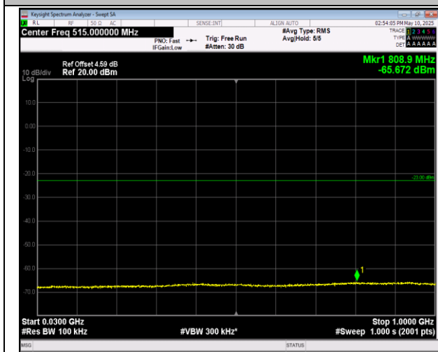
66-66-5MHz-20MHz-QPSK-QPSK-132455-132572-1RB# 24-0RB#0-30-1000MHz-PASS
