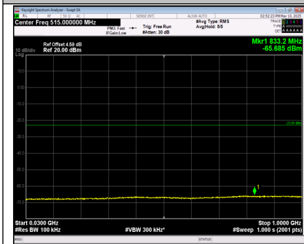
66-66-5MHz-20MHz-16QAM-16QAM-132455-132572-1R B#0-1RB#99-30~1000MHz-PASS
