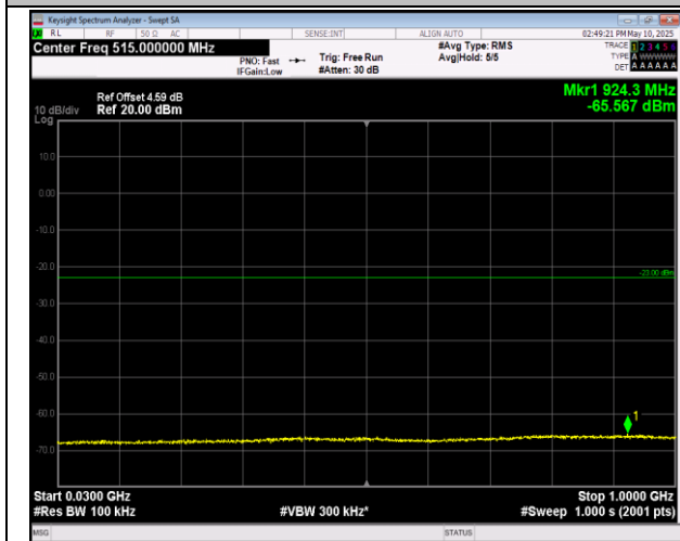
66-66-5MHz-20MHz-QPSK-QPSK-132330-132447-1RB# 24-ORB#0-30~1000MHz-PASS
