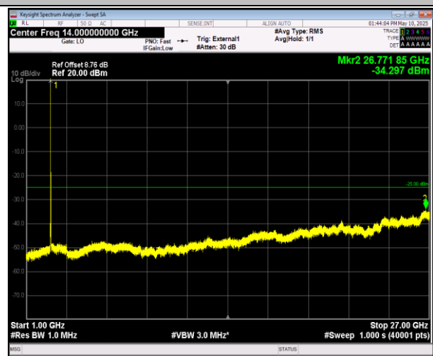
41-41-20MHz-20MHz-QPSK-QPSK-40521-40719-1RB#0-1 RB#99-1000~27000MHz-PASS
