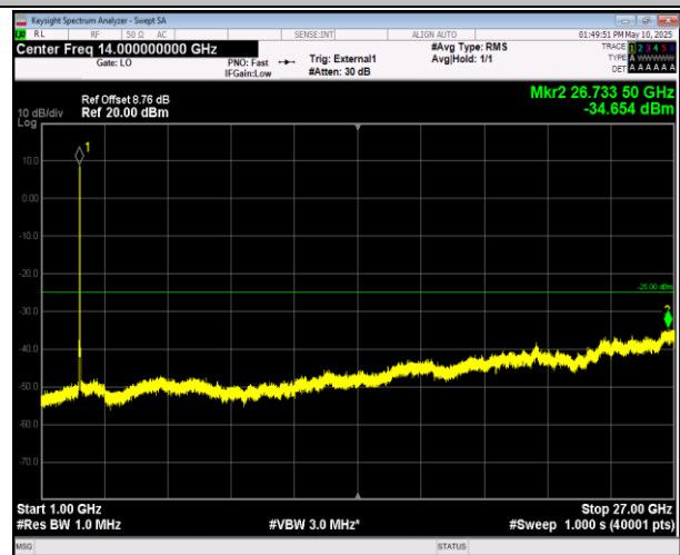
41-41-20MHz-20MHz-QPSK-QPSK-41292-41490-1RB#0-0 RB#0-1000~27000MHz-PASS
