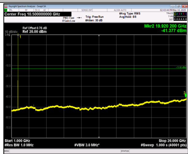
66-66-5MHz-20MHz-QPSK-QPSK-132005-132122-25RB#0 -100RB#0-1000~20000MHz-PASS
