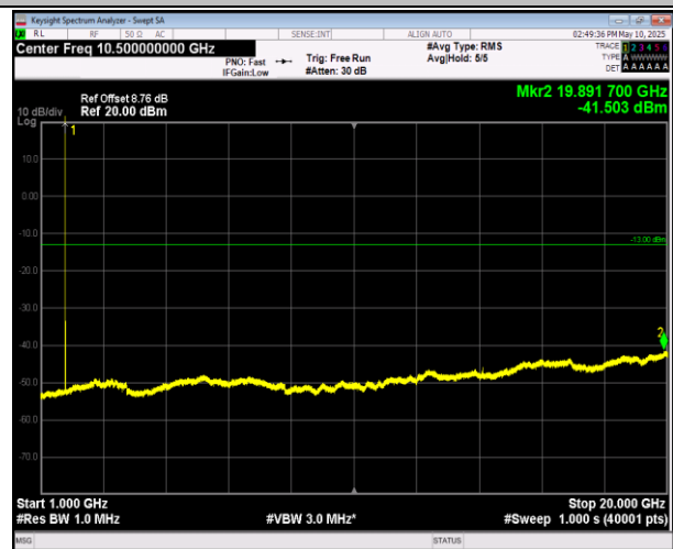
66-66-5MHz-20MHz-QPSK-QPSK-132330-132447-1RB#24 -ORB#0-1000~20000MHz-PASS
