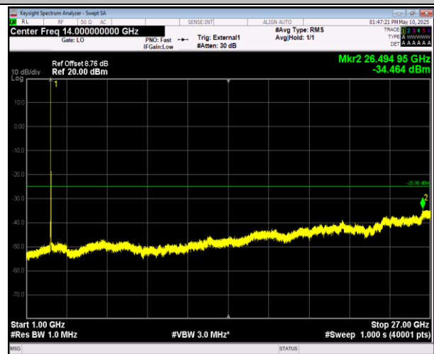
41-41-20MHz-20MHz-QPSK-QPSK-40521-40719-1RB#99- ORB#0-1000~27000MHz-PASS
