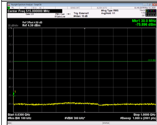
41-41-20MHz-20MHz-QPSK-QPSK-41292-41490-1RB#0 -0RB#0-30~1000MHz-PASS
