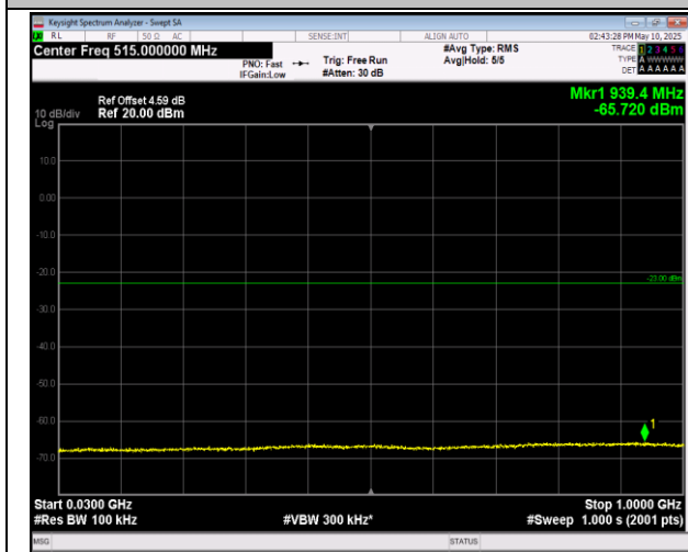
66-66-5MHz-20MHz-QPSK-QPSK-132005-132122-25RB #0-100RB#0-30~1000MHz-PASS
