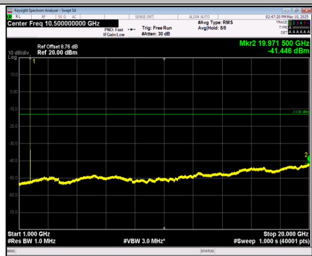
66-66-5MHz-20MHz-QPSK-QPSK-132330-132447-1RB#0- 1RB#99-1000~20000MHz-PASS
