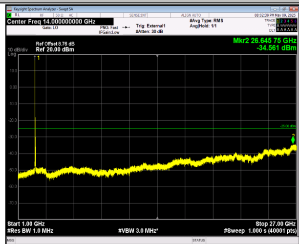
38-38-20MHz-20MHz-16QAM-16QAM-37901-38099-1RB#0 -1RB#99-1000~27000MHz-PASS
