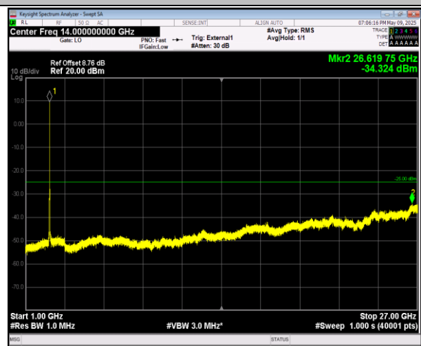
38-38-20MHz-20MHz-QPSK-QPSK-37850-38048-1RB#0-0 RB#0-1000~27000MHz-PASS
