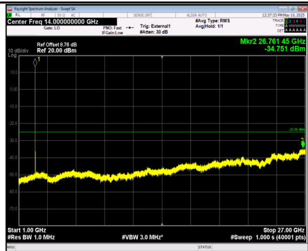
41-41-5MHz-20MHz-QPSK-QPSK-40528-40645-1RB#0-0RB#0-1000~27000MHz-PASS
