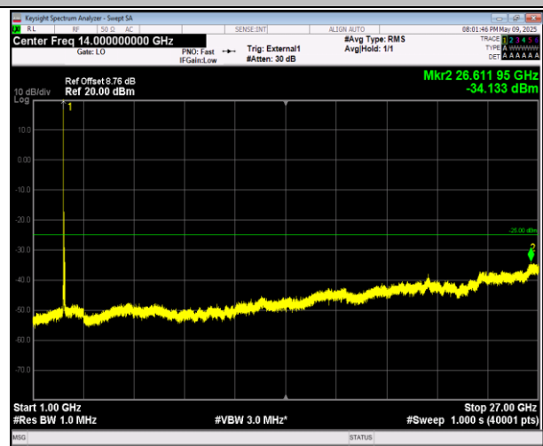
38-38-20MHz-20MHz-QPSK-QPSK-37901-38099-1RB#0-1 RB#99-1000~27000MHz-PASS
