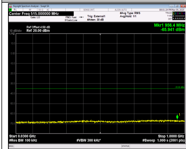
38-38-20MHz-20MHz-QPSK-QPSK-37901-38099-1RB#0 -1RB#99-30~1000MHz-PASS
