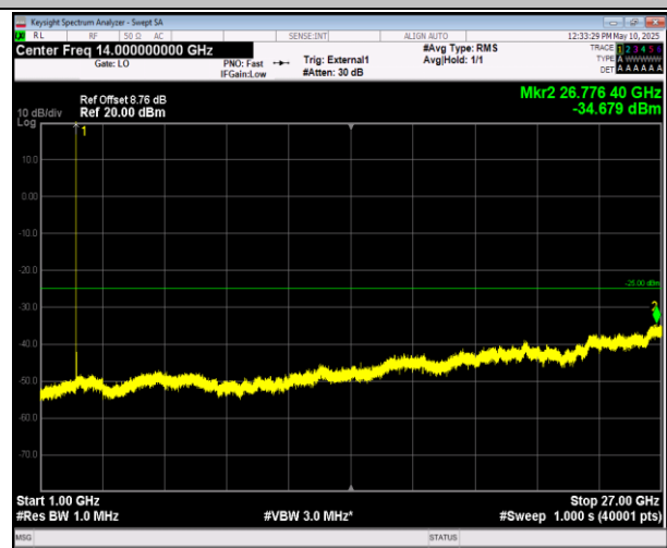
41-41-5MHz-20MHz-QPSK-QPSK-39683-39800-25RB#0-1 00RB#0-1000~27000MHz-PASS
