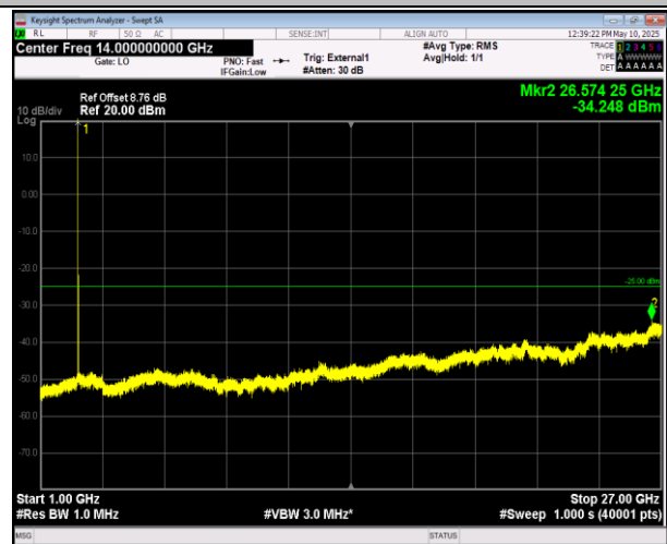
41-41-5MHz-20MHz-16QAM-16QAM-40528-40645-1RB#0- 1RB#99-1000~27000MHz-PASS
