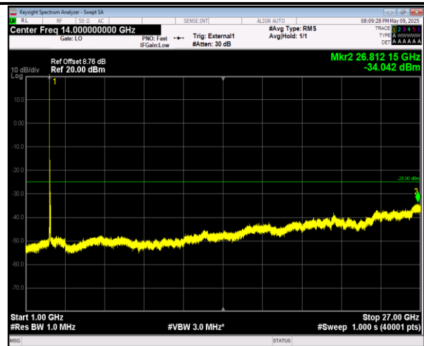
38-38-20MHz-20MHz-QPSK-QPSK-37952-38150-1RB#0-1 RB#99-1000~27000MHz-PASS
