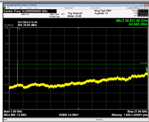
41-41-5MHz-20MHz-QPSK-QPSK-40528-40645-1RB#0-01RB#99-1000~27000MHz-PASS
