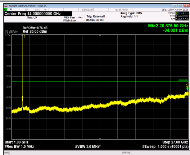
38-38-20MHz-20MHz-QPSK-QPSK-37952-38150-100RB#0 -100RB#0-1000~27000MHz-PASS
