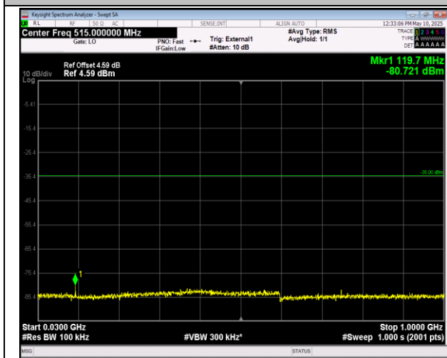
41-41-5MHz-20MHz-QPSK-QPSK-39683-39800-25RB#0 -100RB#0-30~1000MHz-PASS
