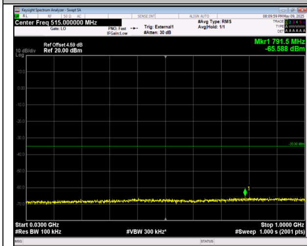
38-38-20MHz-20MHz-16QAM-16QAM-37952-38150-1RB #0-1RB#99-30~1000MHz-PASS
