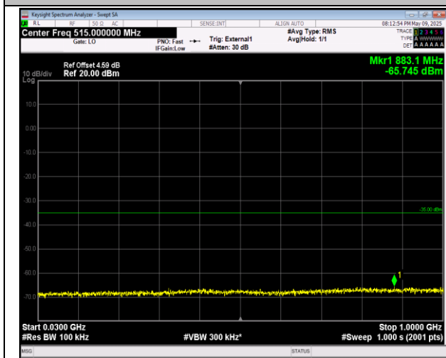
38-38-20MHz-20MHz-QPSK-QPSK-37952-38150-1RB#9 9-0RB#0-30~1000MHz-PASS
