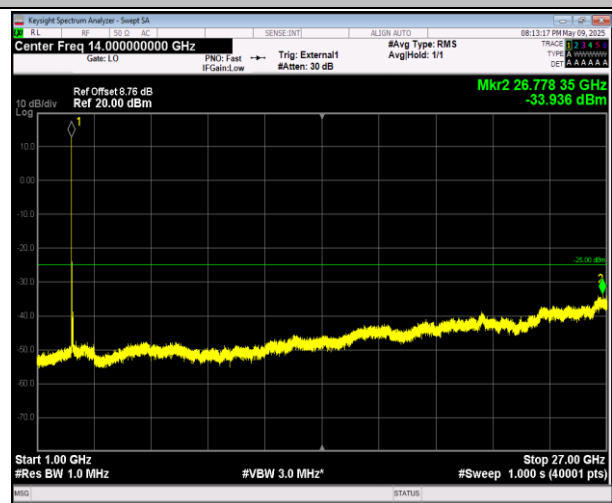
38-38-20MHz-20MHz-QPSK-QPSK-37952-38150-1RB#99- 0RB#0-1000~27000MHz-PASS
