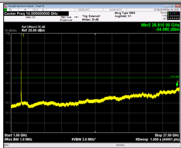
38-38-20MHz-20MHz-QPSK-QPSK-37850-38048-100RB#0 -100RB#0-1000~27000MHz-PASS
