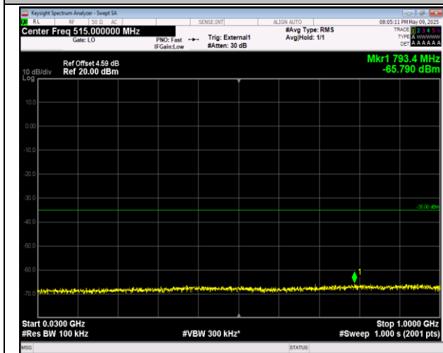
38-38-20MHz-20MHz-QPSK-QPSK-37901-38099-1RB#9 9-ORB#0-30~1000MHz-PASS
