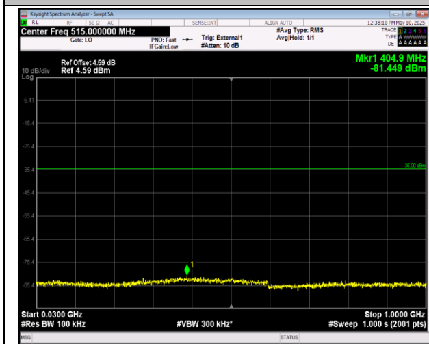
41-41-5MHz-20MHz-QPSK-QPSK-40528-40645-1RB#0-01RB#99-30~1000MHz-PASS
