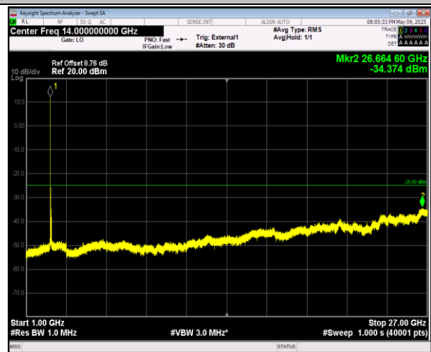
38-38-20MHz-20MHz-QPSK-QPSK-37901-38099-1RB#99- ORB#0-1000~27000MHz-PASS
