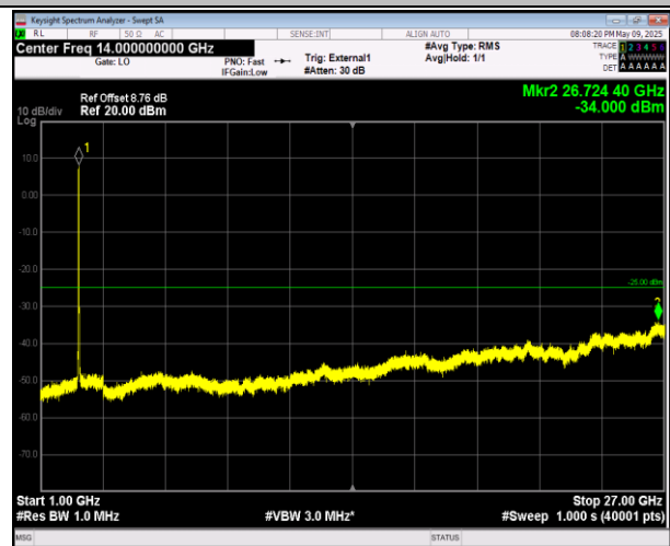
38-38-20MHz-20MHz-QPSK-QPSK-37952-38150-1RB#0-0 RB#0-1000~27000MHz-PASS
