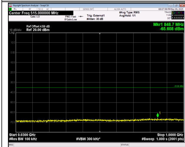
38-38-20MHz-20MHz-QPSK-QPSK-37952-38150-1RB#0 -0RB#0-30~1000MHz-PASS
