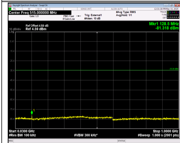
41-41-5MHz-20MHz-QPSK-QPSK-39683-39800-1RB#0-01RB#99-30~1000MHz-PASS
