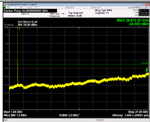
41-41-5MHz-20MHz-QPSK-QPSK-40528-40645-1RB#24-0RB#0-1000~27000MHz-PASS
