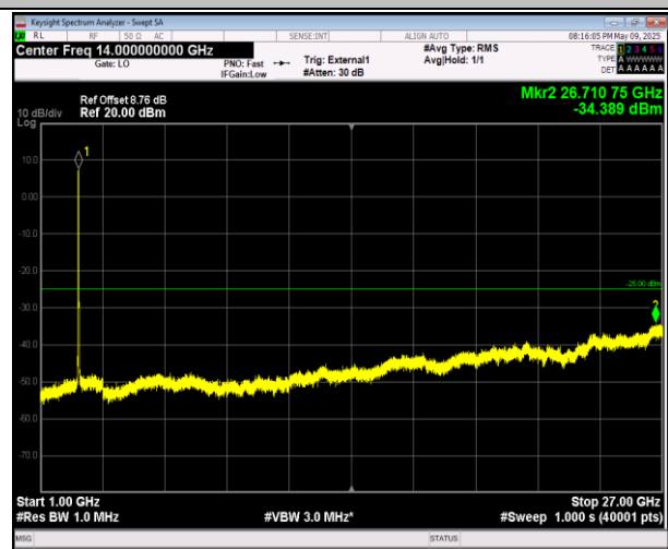
41-41-5MHz-20MHz-QPSK-QPSK-39683-39800-1RB#0-0RB#0-1000~27000MHz-PASS
