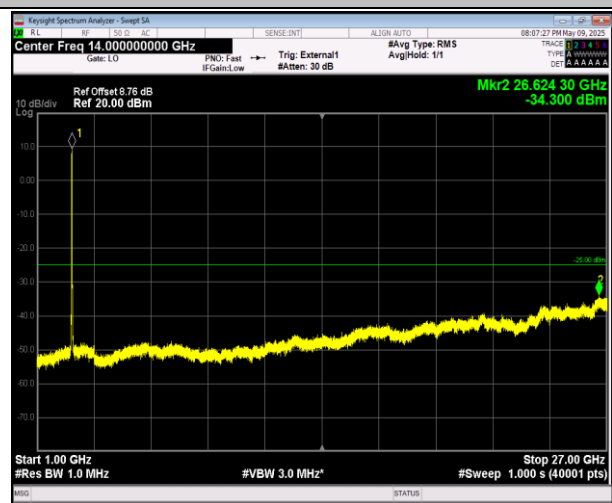
38-38-20MHz-20MHz-16QAM-16QAM-37901-38099-1RB#0 -0RB#0-1000~27000MHz-PASS
