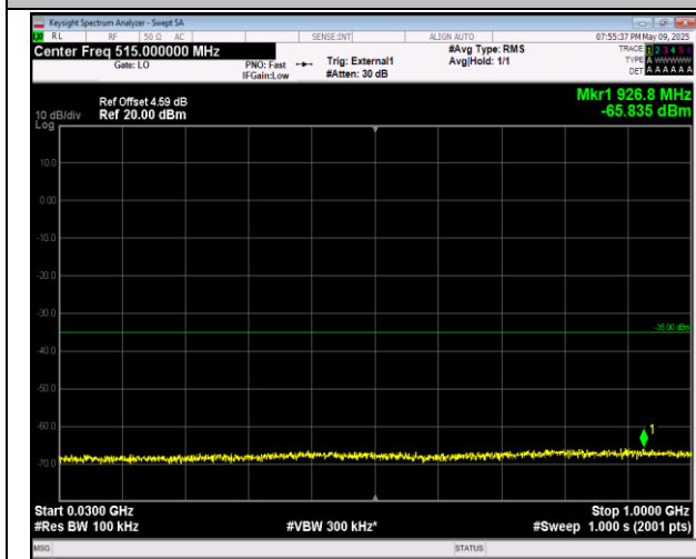
38-38-20MHz-20MHz-QPSK-QPSK-37850-38048-100RB #0-100RB#0-30~1000MHz-PASS
