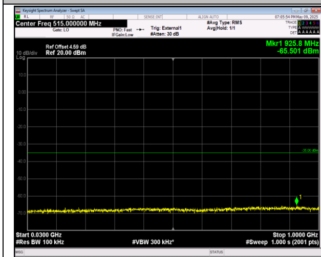
38-38-20MHz-20MHz-QPSK-QPSK-37850-38048-1RB#0 -0RB#0-30~1000MHz-PASS
