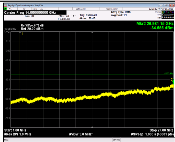
41-41-5MHz-20MHz-QPSK-QPSK-39683-39800-1RB#0-01RB#99-1000~27000MHz-PASS
