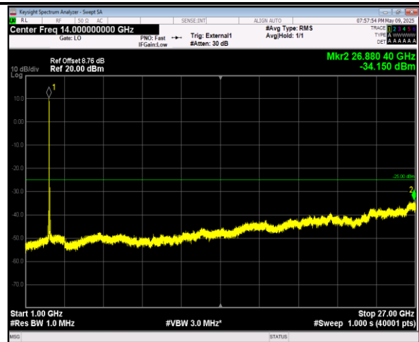
38-38-20MHz-20MHz-QPSK-QPSK-37850-38048-1RB#99- ORB#0-1000~27000MHz-PASS
