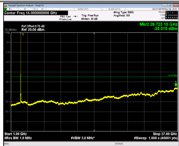
7-7-20MHz-20MHz-QPSK-QPSK-21152-21350-100RB#0-1 00RB#0-1000~27000MHz-PASS
