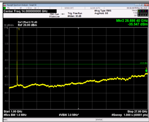
7-7-20MHz-20MHz-QPSK-QPSK-20850-21048-100RB#0-1 00RB#0-1000~27000MHz-PASS
