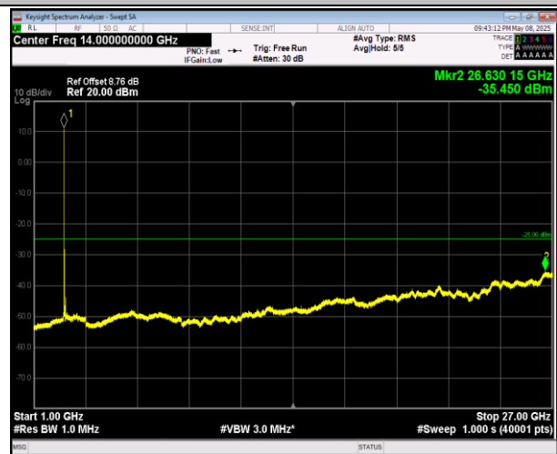
7-7-20MHz-20MHz-QPSK-QPSK-21001-21199-1RB#99-0RB B#0-1000~27000MHz-PASS
