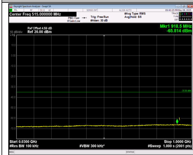
7-7-20MHz-20MHz-QPSK-QPSK-21001-21199-1RB#0-1 RB#99-30~1000MHz-PASS
