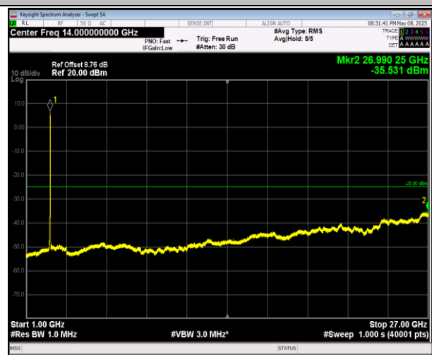
7-7-20MHz-20MHz-QPSK-QPSK-20850-21048-1RB#0-0RB #0-1000~27000MHz-PASS
