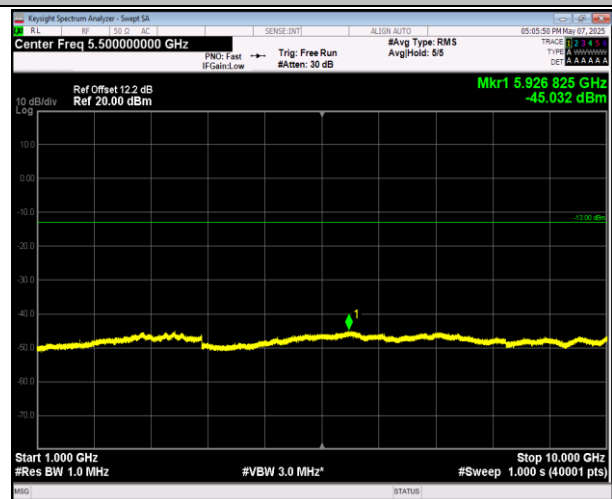
5-5-10MHz-10MHz-QPSK-QPSK-20501-20600-50RB#0-50RB#0-1000~10000MHz-PASS
