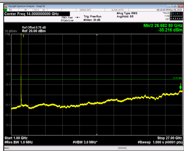
7-7-20MHz-10MHz-QPSK-QPSK-20850-20994-100RB#0-50RB#0-1000~27000MHz-PASS
