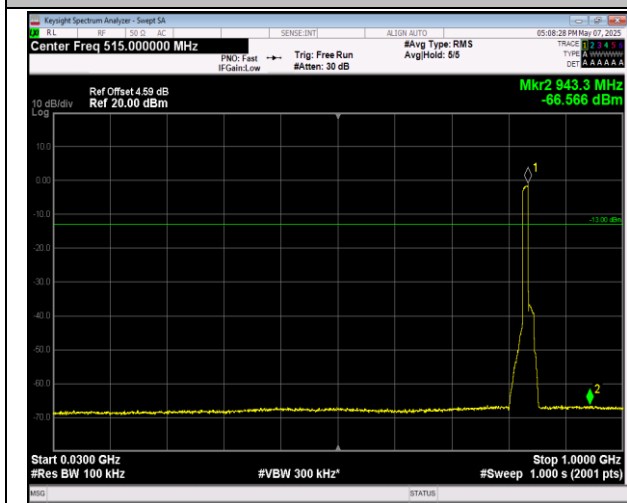
7-7-10MHz-20MHz-QPSK-QPSK-20805-20949-1RB#0-0 RB#0-30~1000MHz-PASS
