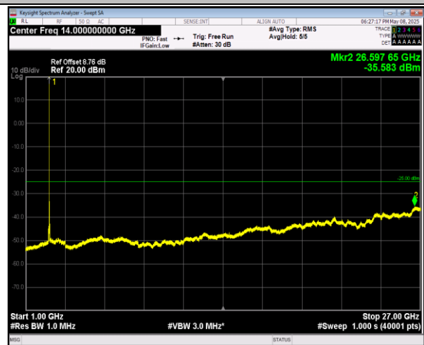
7-7-10MHz-20MHz-QPSK-QPSK-21206-21350-50RB#0-10 ORB#0-1000~27000MHz-PASS
