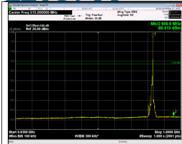
5-5-10MHz-10MHz-QPSK-QPSK-20476-20575-50RB#0-50RB#0-30~1000MHz-PASS
