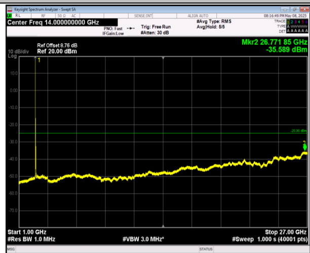
7-7-20MHz-10MHz-QPSK-QPSK-20850-20994-1RB#0-0-1RB#49-1000~27000MHz-PASS
