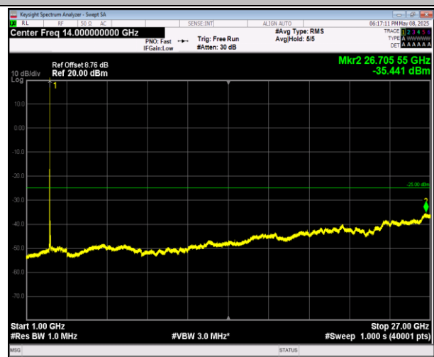
7-7-10MHz-20MHz-QPSK-QPSK-20805-20949-50RB#0-100RB#0-1000~27000MHz-PASS
