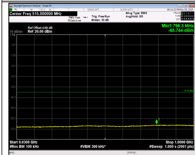
7-7-20MHz-10MHz-QPSK-QPSK-20850-20994-1RB#0-0-1RB#49-30~1000MHz-PASS
