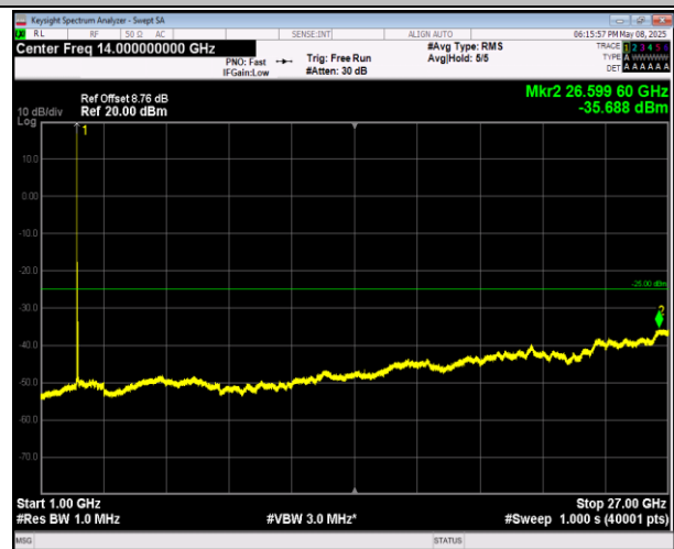
7-7-10MHz-20MHz-QPSK-QPSK-20805-20949-1RB#0-1RB #99-1000~27000MHz-PASS
