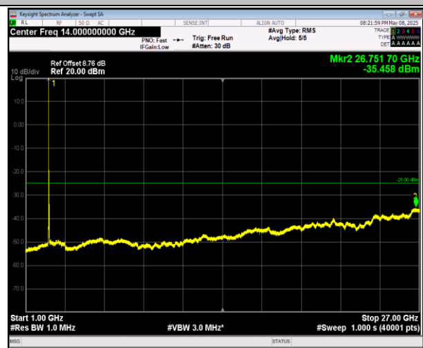
7-7-20MHz-10MHz-QPSK-QPSK-21051-21195-1RB#0-1RB #49-1000~27000MHz-PASS
