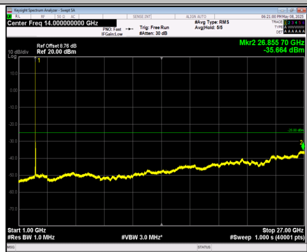
7-7-10MHz-20MHz-QPSK-QPSK-21006-21150-1RB#0-1RB #99-1000~27000MHz-PASS
