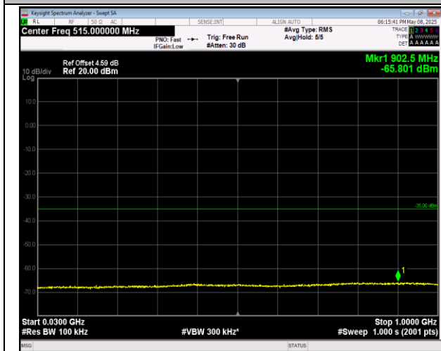
7-7-10MHz-20MHz-QPSK-QPSK-20805-20949-1RB#0-1 RB#99-30~1000MHz-PASS
