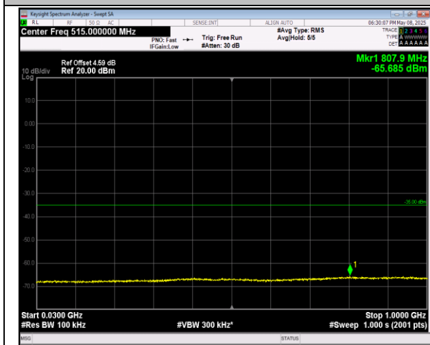
7-7-20MHz-10MHz-QPSK-QPSK-20850-20994-1RB#0-0-RB#0-30~1000MHz-PASS
