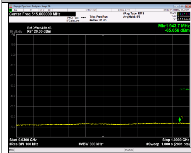
7-7-20MHz-10MHz-QPSK-QPSK-20850-20994-100RB#0-50RB#0-30~1000MHz-PASS
