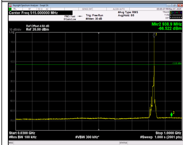
5-5-10MHz-10MHz-QPSK-QPSK-20501-20600-50RB#0-050RB#0-30~1000MHz-PASS
