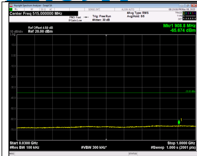
7-7-20MHz-10MHz-QPSK-QPSK-20850-20994-1RB#99-0RB#0-30~1000MHz-PASS
