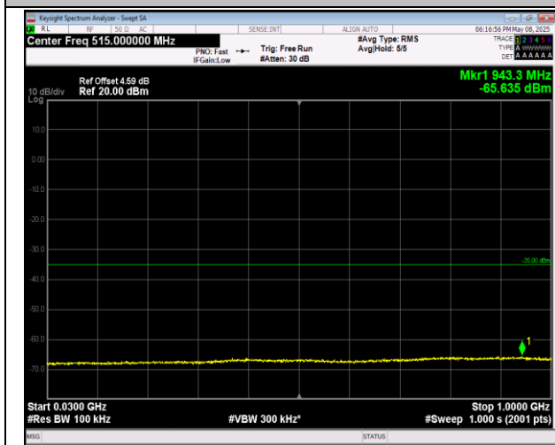
7-7-10MHz-20MHz-QPSK-QPSK-20805-20949-50RB#0-100RB#0-30~1000MHz-PASS
