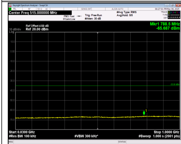
7-7-10MHz-20MHz-QPSK-QPSK-21206-21350-50RB#0-0- 100RB#0-30~1000MHz-PASS
