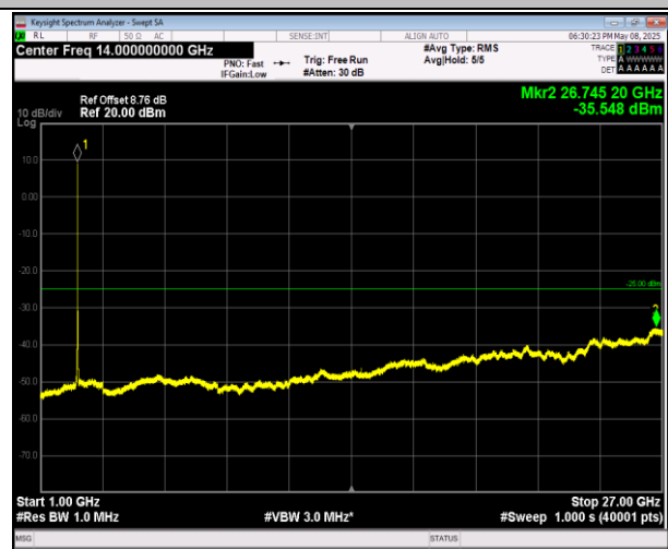
7-7-20MHz-10MHz-QPSK-QPSK-20850-20994-1RB#0-0RB#0-1000~27000MHz-PASS
