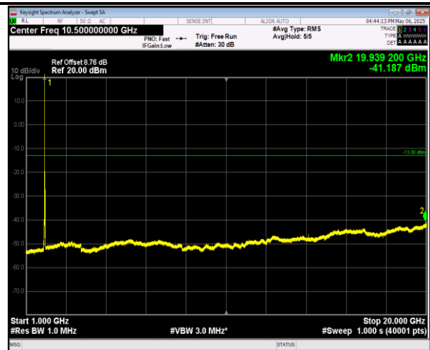
2-2-20MHz-20MHz-QPSK-QPSK-18902-19100-1RB#0-1RB #99-1000~20000MHz-PASS
