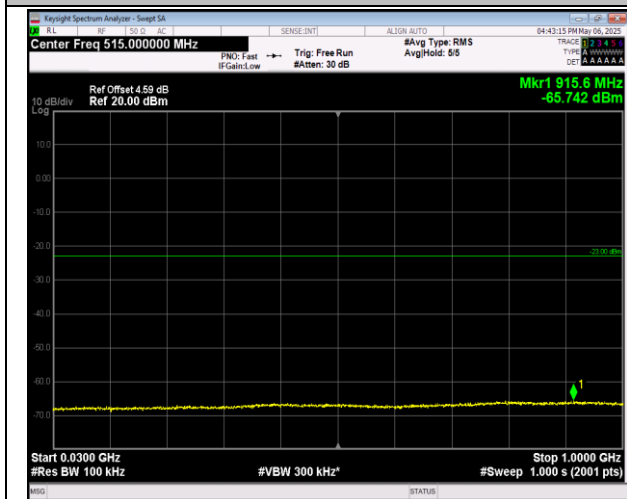
2-2-20MHz-20MHz-QPSK-QPSK-18902-19100-1RB#0-0 RB#0-30~1000MHz-PASS
