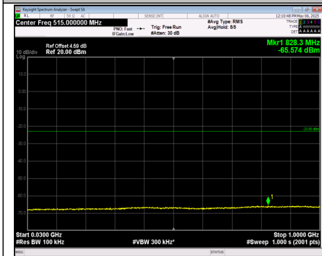
2-2-5MHz-20MHz-QPSK-QPSK-18983-19100-25RB#0-1 00RB#0-30~1000MHz-PASS
