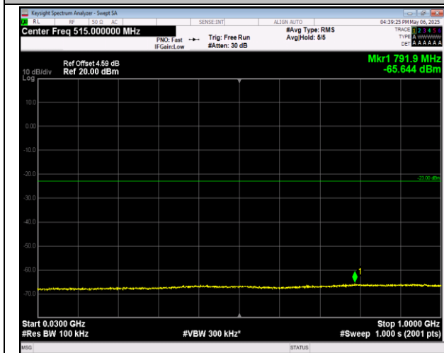
2-2-20MHz-20MHz-16QAM-16QAM-18801-18999-1RB#0 -1RB#99-30~1000MHz-PASS
