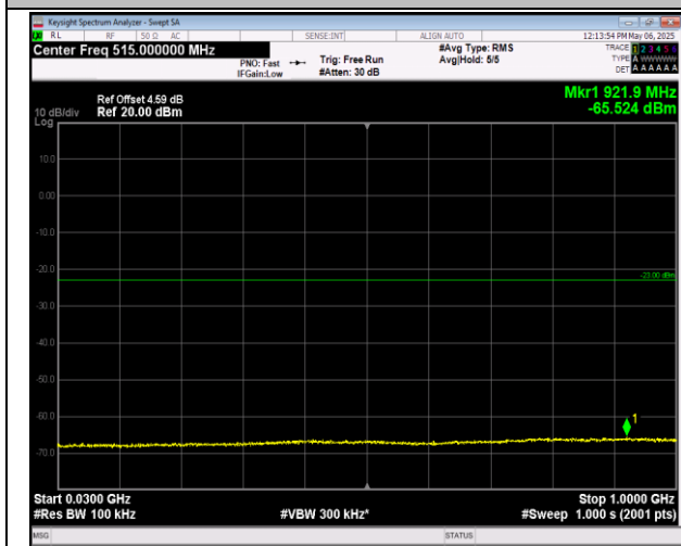
2-2-20MHz-20MHz-QPSK-QPSK-18700-18898-1RB#0-0 RB#0-30~1000MHz-PASS
