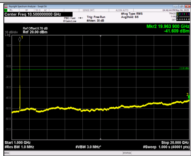
2-2-20MHz-20MHz-QPSK-QPSK-18902-19100-1RB#99-0R B#0-1000~20000MHz-PASS
