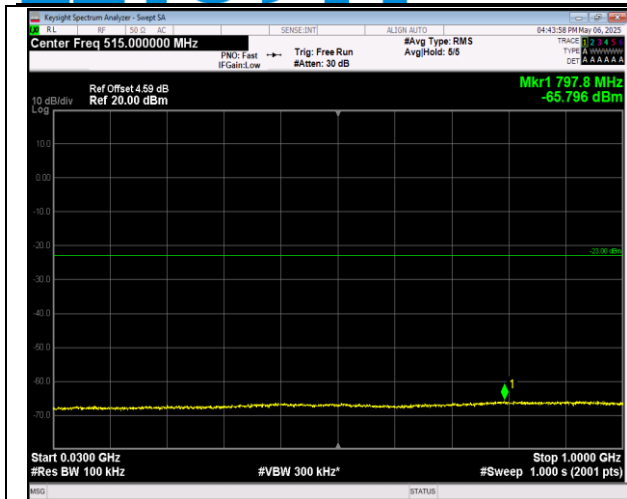
2-2-20MHz-20MHz-QPSK-QPSK-18902-19100-1RB#0-1 RB#99-30~1000MHz-PASS
