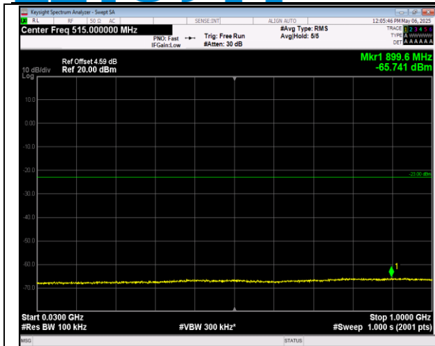
2-2-5MHz-20MHz-QPSK-QPSK-18808-18925-25RB#0-1 00RB#0-30~1000MHz-PASS
