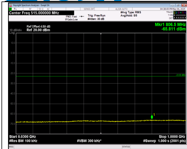
2-2-20MHz-20MHz-QPSK-QPSK-18801-18999-1RB#0-0 RB#0-30~1000MHz-PASS
