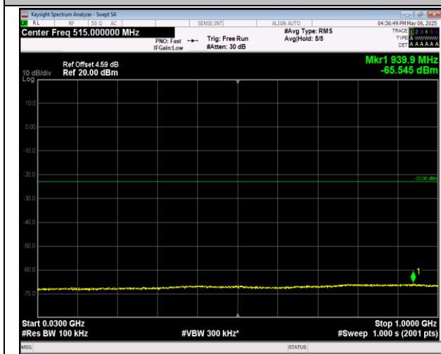
2-2-20MHz-20MHz-16QAM-16QAM-18700-18898-1RB#9 9-0RB#0-30~1000MHz-PASS
