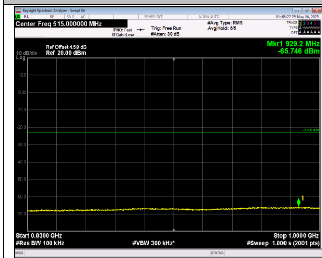
5-5-3MHz-5MHz-QPSK-QPSK-20416-20455-1RB#0-0RB #0-30~1000MHz-PASS
