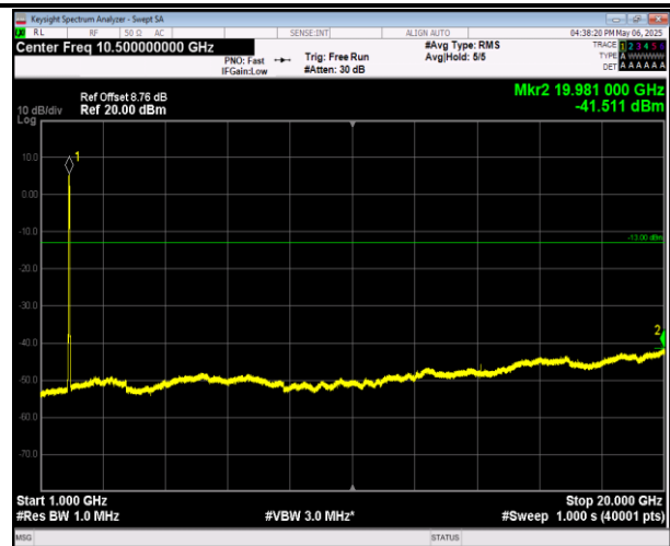
2-2-20MHz-20MHz-QPSK-QPSK-18801-18999-1RB#0-0RB #0-1000~20000MHz-PASS
