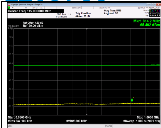
2-2-5MHz-20MHz-QPSK-QPSK-18983-19100-1RB#0-1R B#99-30~1000MHz-PASS
