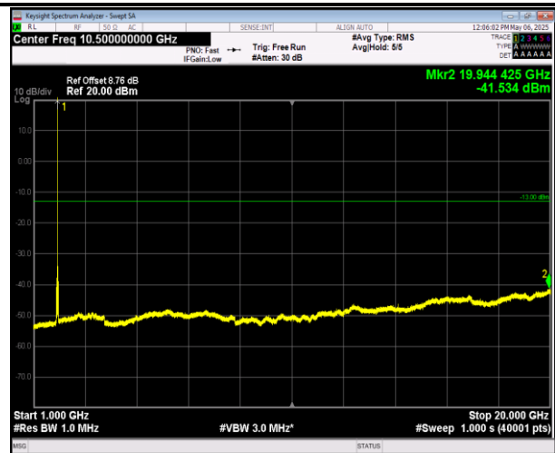
2-2-5MHz-20MHz-QPSK-QPSK-18808-18925-25RB#0-100 RB#0-1000~20000MHz-PASS
