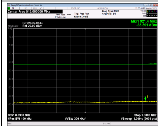
2-2-5MHz-20MHz-QPSK-QPSK-18633-18750-25RB#0-1 00RB#0-30~1000MHz-PASS
