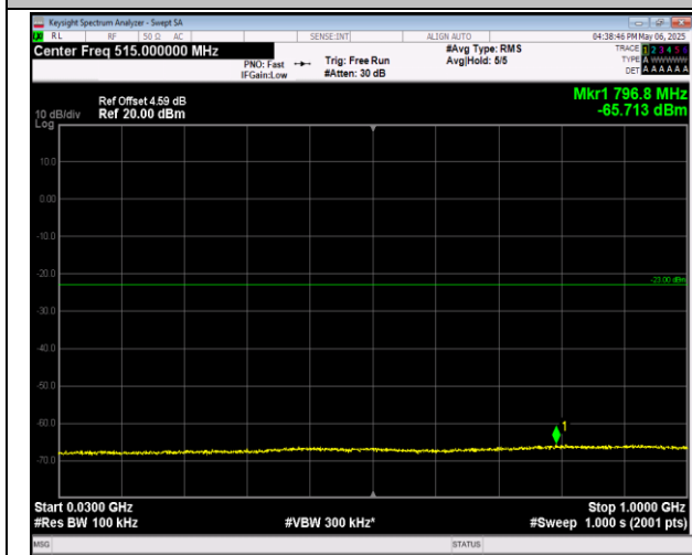
2-2-20MHz-20MHz-QPSK-QPSK-18801-18999-1RB#0-1 RB#99-30~1000MHz-PASS
