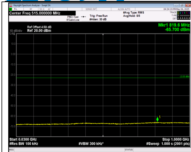
2-2-20MHz-20MHz-16QAM-16QAM-18700-18898-1RB#0 -1RB#99-30~1000MHz-PASS
