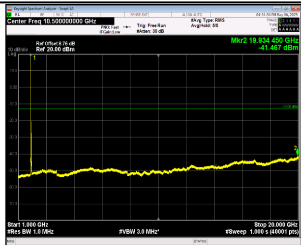
2-2-20MHz-20MHz-16QAM-16QAM-18700-18898-1RB#0-1 RB#99-1000~20000MHz-PASS
