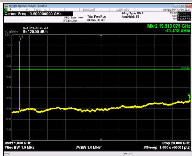
2-2-20MHz-20MHz-QPSK-QPSK-18801-18999-1RB#99-0R B#0-1000~20000MHz-PASS
