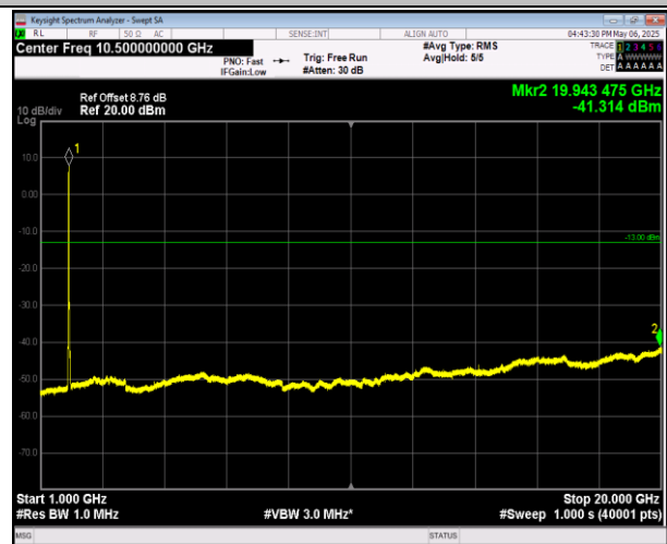
2-2-20MHz-20MHz-QPSK-QPSK-18902-19100-1RB#0-ORB #0-1000~20000MHz-PASS
