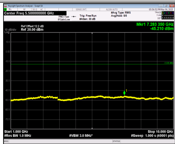
5-5-3MHz-5MHz-QPSK-QPSK-20416-20455-15RB#0-25RB #0-1000~10000MHz-PASS
