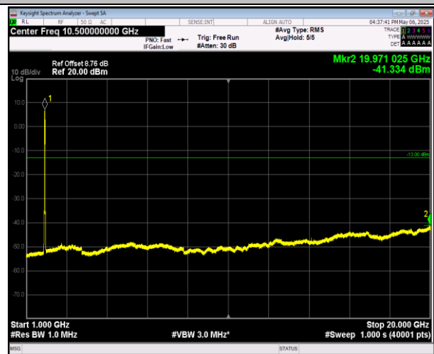
2-2-20MHz-20MHz-16QAM-16QAM-18700-18898-1RB#0-0 RB#0-1000~20000MHz-PASS
