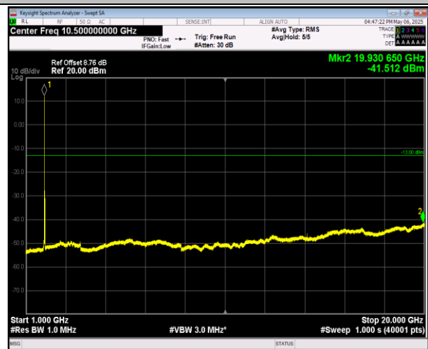
2-2-20MHz-20MHz-16QAM-16QAM-18902-19100-1RB#99- ORB#0-1000~20000MHz-PASS
