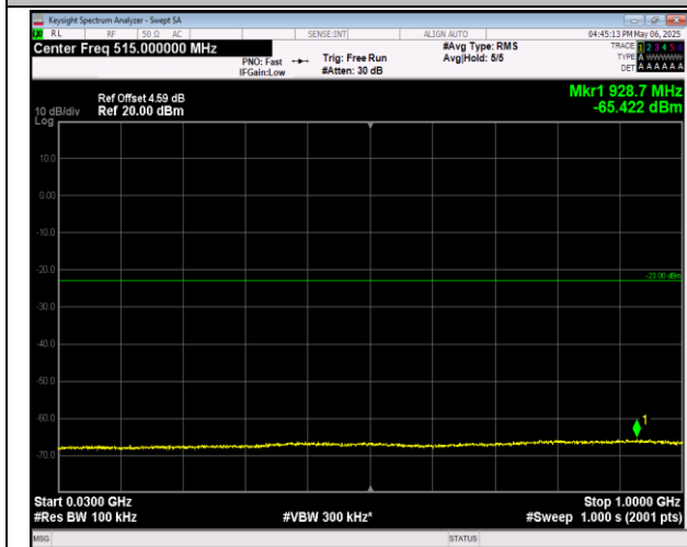
2-2-20MHz-20MHz-QPSK-QPSK-18902-19100-100RB#0- -100RB#0-30~1000MHz-PASS
