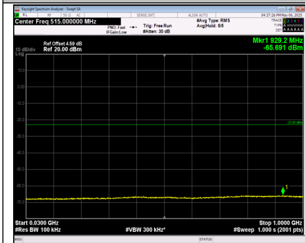
2-2-20MHz-20MHz-16QAM-16QAM-18700-18898-1RB#0-0RB#0-30~1000MHz-PASS
