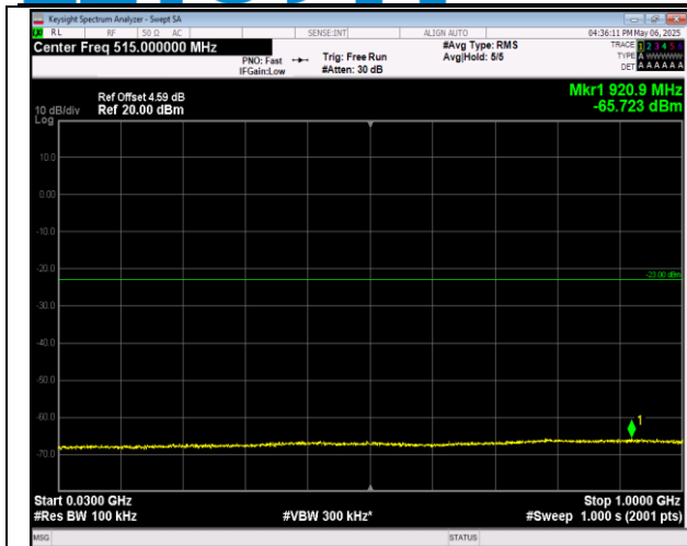
2-2-20MHz-20MHz-QPSK-QPSK-18700-18898-1RB#99-0RB#0-30~1000MHz-PASS
