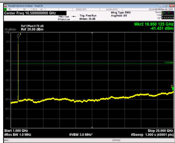
2-2-20MHz-20MHz-QPSK-QPSK-18700-18898-1RB#0-0RB #0-1000~20000MHz-PASS
