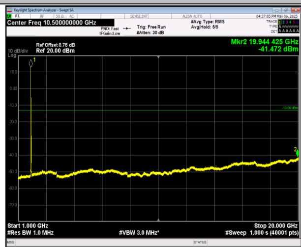
2-2-20MHz-20MHz-16QAM-16QAM-18700-18898-1RB#99- 0RB#0-1000~20000MHz-PASS
