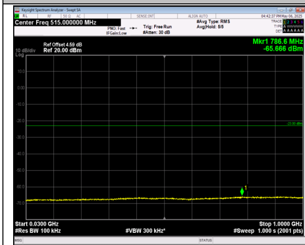
2-2-20MHz-20MHz-16QAM-16QAM-18801-18999-1RB#0 -0RB#0-30~1000MHz-PASS
