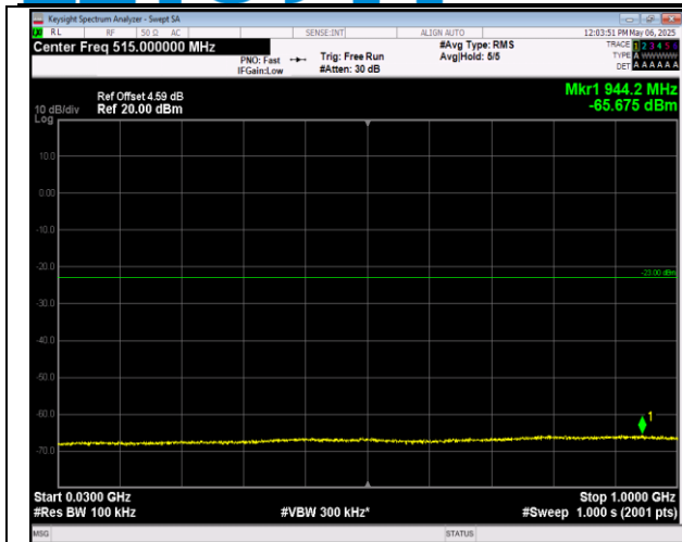
2-2-5MHz-20MHz-QPSK-QPSK-18808-18925-1RB#0-0R B#0-30~1000MHz-PASS
