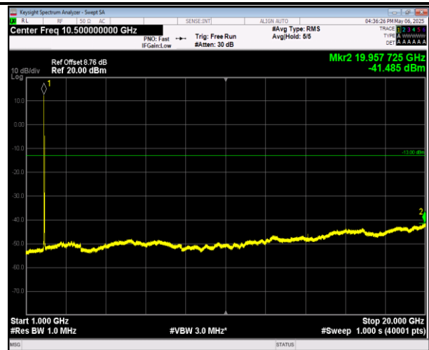
2-2-20MHz-20MHz-QPSK-QPSK-18700-18898-1RB#99-0R B#0-1000~20000MHz-PASS
