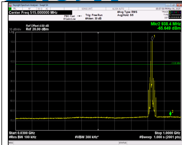
5-5-3MHz-5MHz-QPSK-QPSK-20416-20455-1RB#14-0R B#0-30~1000MHz-PASS
