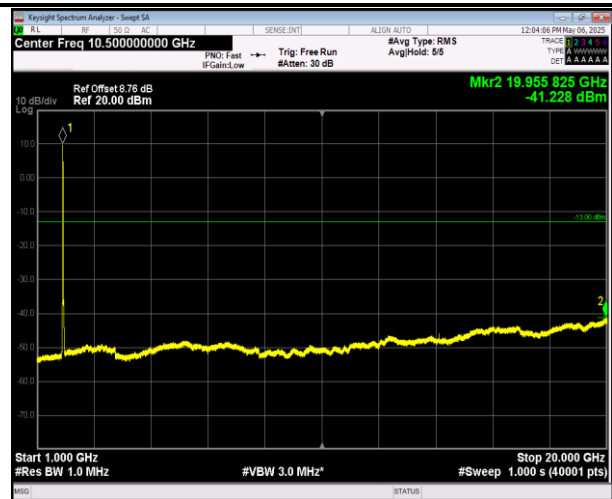
2-2-5MHz-20MHz-QPSK-QPSK-18808-18925-1RB#0-0RB# 0-1000~20000MHz-PASS
