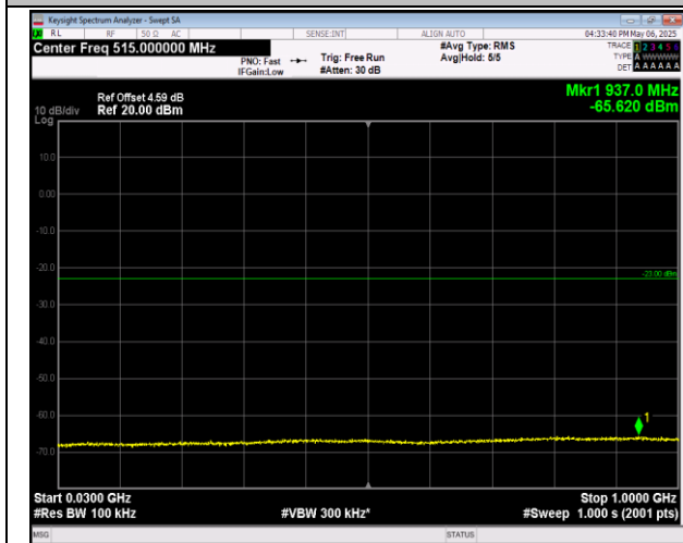
2-2-20MHz-20MHz-QPSK-QPSK-18700-18898-1RB#0-1 RB#99-30~1000MHz-PASS
