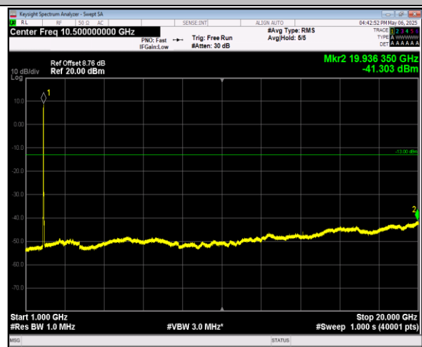
2-2-20MHz-20MHz-16QAM-16QAM-18801-18999-1RB#0-0 RB#0-1000~20000MHz-PASS
