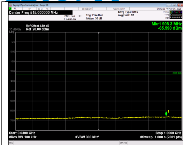
2-2-20MHz-20MHz-QPSK-QPSK-18801-18999-100RB#0 -100RB#0-30~1000MHz-PASS
