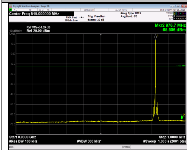
5-5-3MHz-5MHz-QPSK-QPSK-20416-20455-15RB#0-25 RB#0-30~1000MHz-PASS
