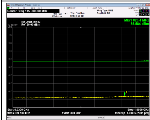
2-2-5MHz-20MHz-QPSK-QPSK-18808-18925-1RB#0-1R B#99-30~1000MHz-PASS
