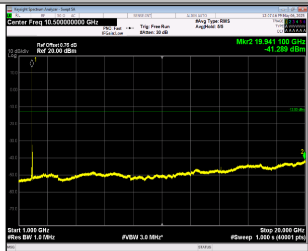
2-2-5MHz-20MHz-QPSK-QPSK-18808-18925-1RB#24-0RB #0-1000~20000MHz-PASS
