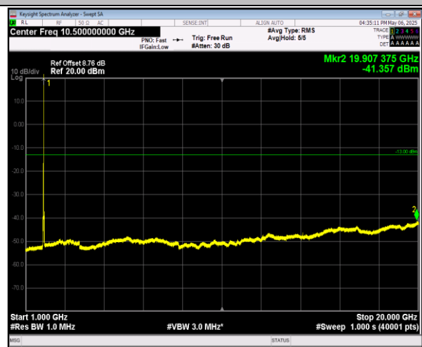
2-2-20MHz-20MHz-QPSK-QPSK-18700-18898-100RB#0-1 00RB#0-1000~20000MHz-PASS
