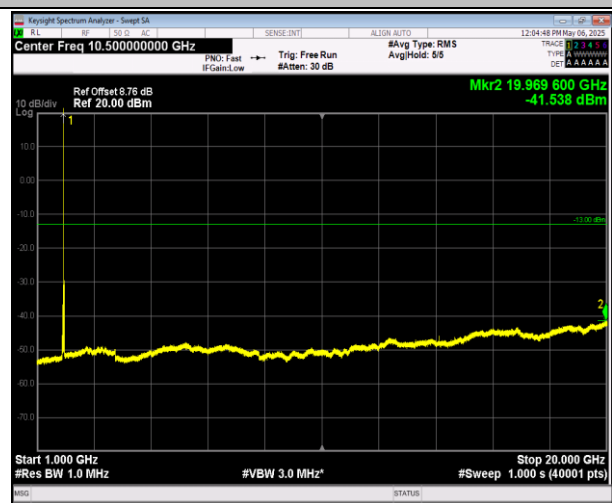
2-2-5MHz-20MHz-QPSK-QPSK-18808-18925-1RB#0-1RB# 99-1000~20000MHz-PASS
