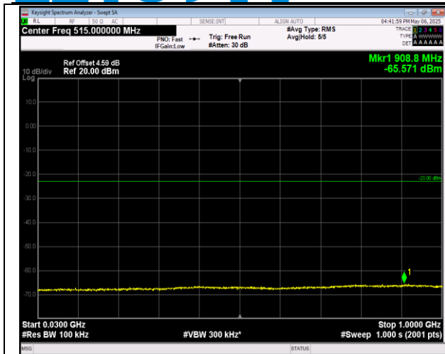
2-2-20MHz-20MHz-16QAM-16QAM-18801-18999-1RB#9 9-ORB#0-30~1000MHz-PASS
