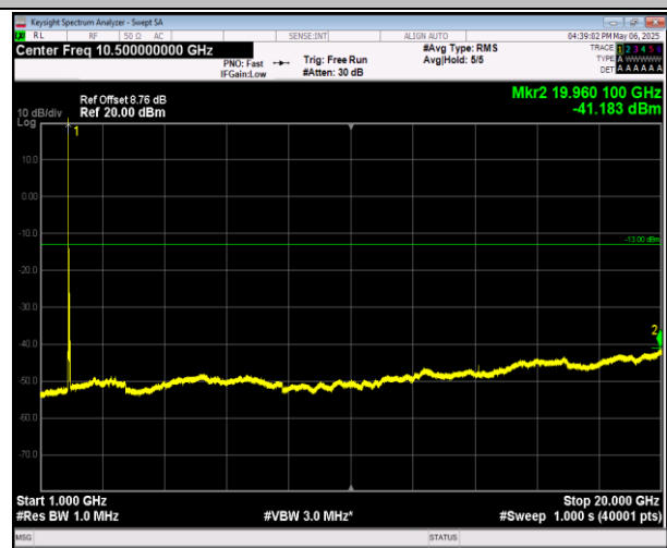
2-2-20MHz-20MHz-QPSK-QPSK-18801-18999-1RB#0-1RB #99-1000~20000MHz-PASS
