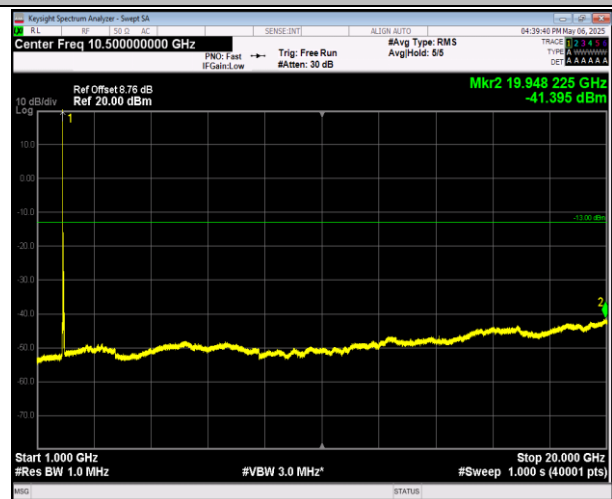
2-2-20MHz-20MHz-16QAM-16QAM-18801-18999-1RB#0-1 RB#99-1000~20000MHz-PASS
