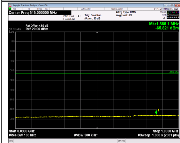
2-2-20MHz-20MHz-QPSK-QPSK-18801-18999-1RB#99-9 ORB#0-30~1000MHz-PASS
