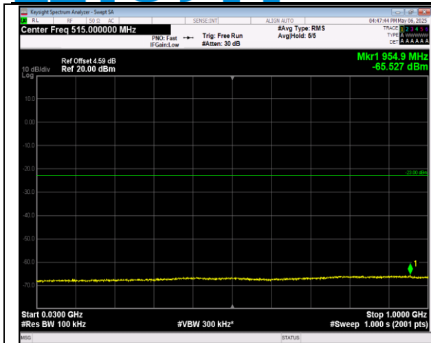
2-2-20MHz-20MHz-16QAM-16QAM-18902-19100-1RB#0 -ORB#0-30~1000MHz-PASS
