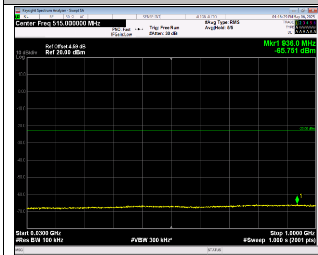
2-2-20MHz-20MHz-QPSK-QPSK-18902-19100-1RB#99-99- ORB#0-30~1000MHz-PASS
