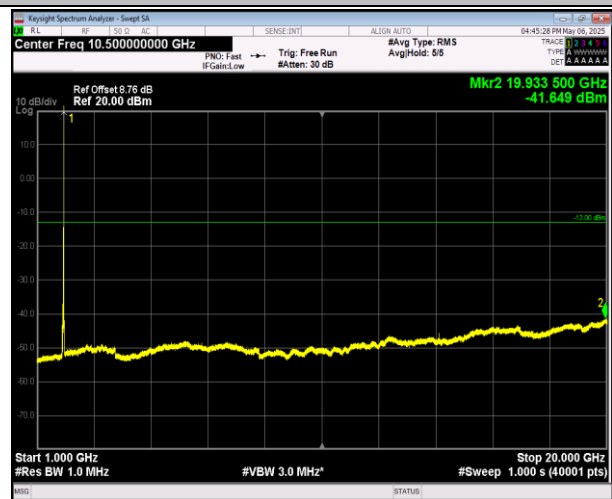
2-2-20MHz-20MHz-QPSK-QPSK-18902-19100-100RB#0-1 00RB#0-1000~20000MHz-PASS
