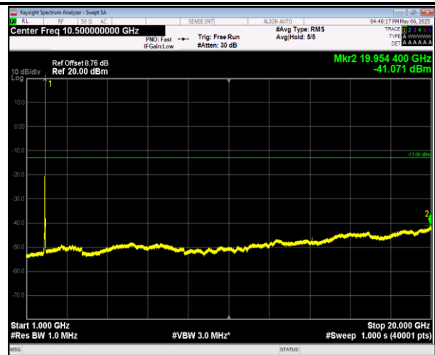
2-2-20MHz-20MHz-QPSK-QPSK-18801-18999-100RB#0-1 00RB#0-1000~20000MHz-PASS
