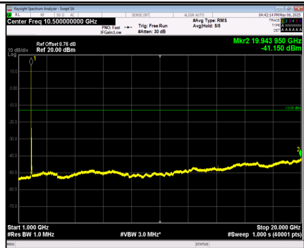
2-2-20MHz-20MHz-16QAM-16QAM-18801-18999-1RB#99- ORB#0-1000~20000MHz-PASS
