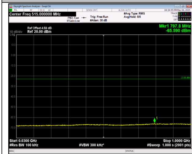
2-2-20MHz-20MHz-QPSK-QPSK-18700-18898-100RB#0-100RB#0-30~1000MHz-PASS
