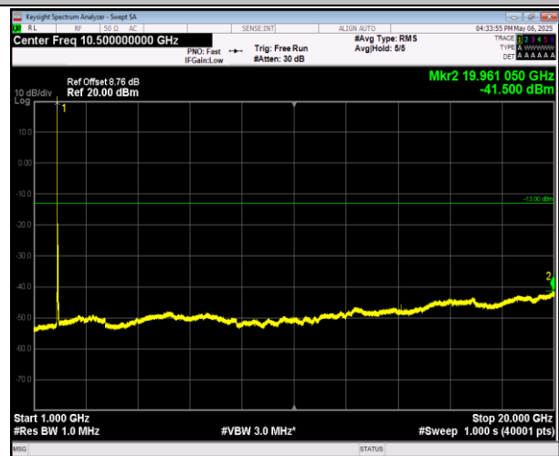
2-2-20MHz-20MHz-QPSK-QPSK-18700-18898-1RB#0-1RB #99-1000~20000MHz-PASS
