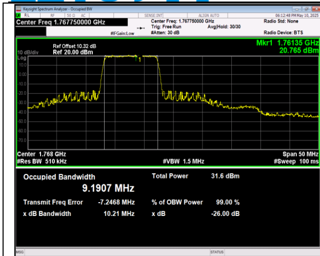
66-66-10MHz-20MHz-QPSK-QPSK-132027-132171-50R B#0-100RB#0-PASS
