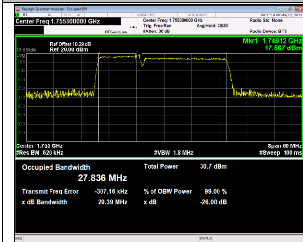
66-66-10MHz-20MHz-QPSK-QPSK-132428-132572-50R B#0-100RB#0-PASS
