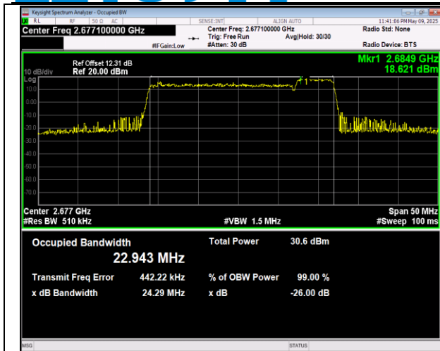
41-41-20MHz-10MHz-QPSK-QPSK-39750-39894-100RB #0-50RB#0-PASS
