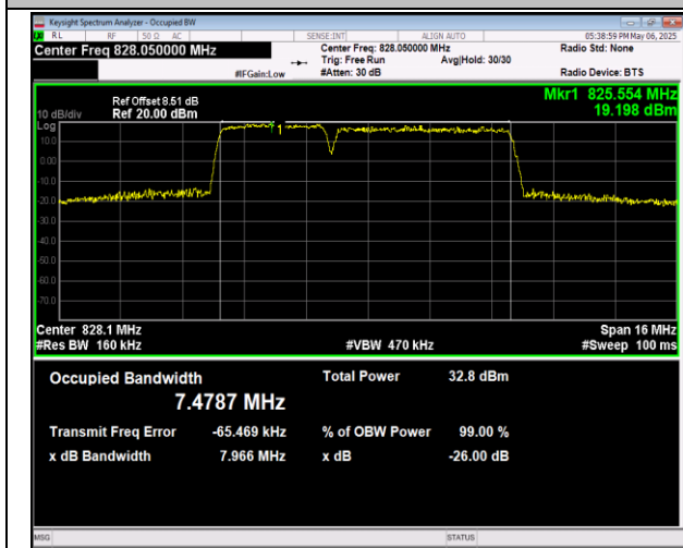
5-5-3MHz-5MHz-QPSK-QPSK-20501-20540-15RB#0-25 RB#0-PASS
