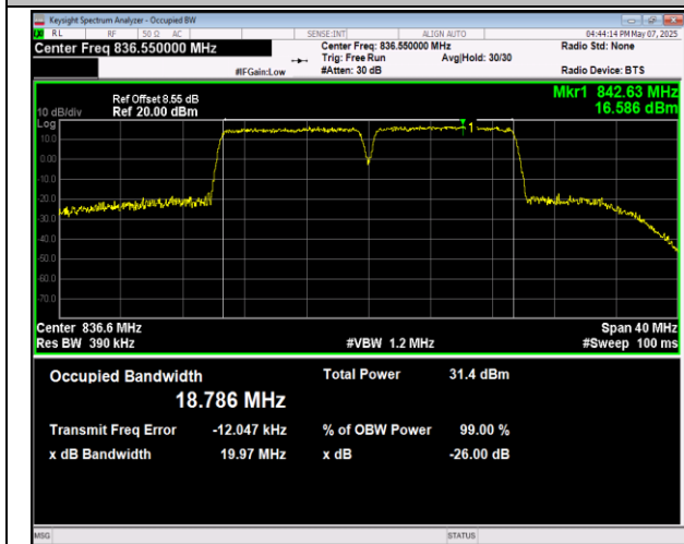
5-5-10MHz-10MHz-QPSK-QPSK-20501-20600-50RB#0-50RB#0-PASS
