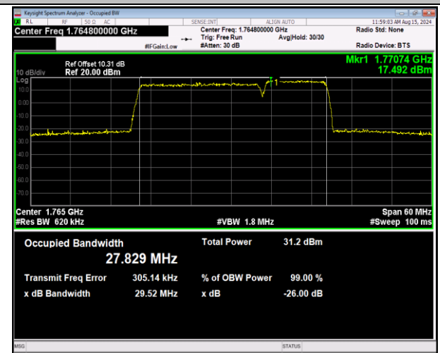
66-66-20MHz-10MHz-QPSK-QPSK-132473-132617-100R B#0-50RB#0-PASS
