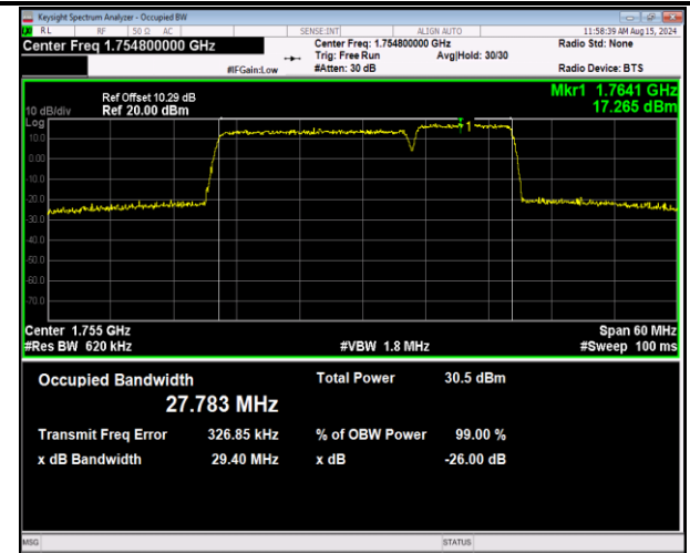
66-66-20MHz-10MHz-16QAM-16QAM-132373-132517-10 ORB#0-50RB#0-PASS
