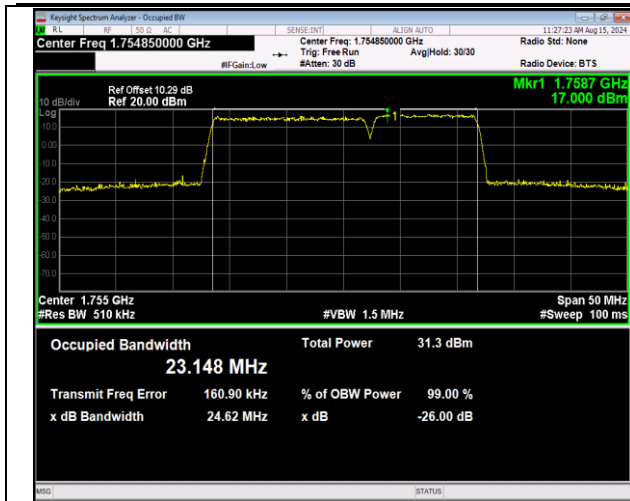
66-66-15MHz-10MHz-QPSK-QPSK-132373-132493-75RB #0-50RB#0-PASS
