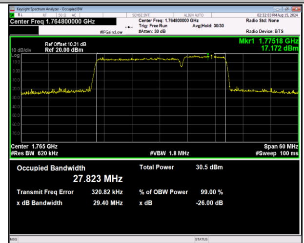
66-66-20MHz-10MHz-64QAM-64QAM-132473-132617-10 ORB#0-50RB#0-PASS
