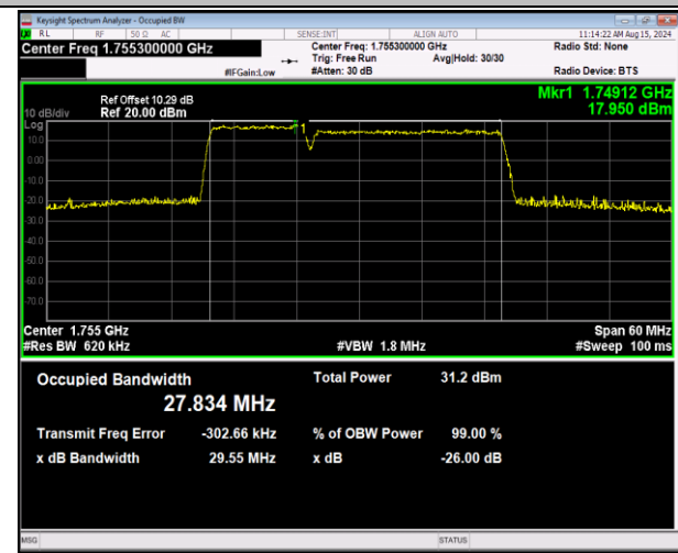
66-66-10MHz-20MHz-QPSK-QPSK-132328-132472-50RB #0-100RB#0-PASS
