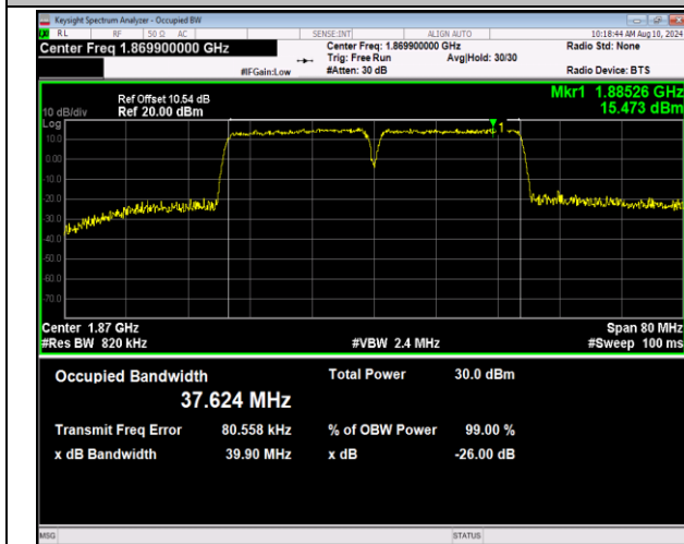
2-2-20MHz-20MHz-16QAM-16QAM-18700-18898-100RB#0-100RB#0-PASS
