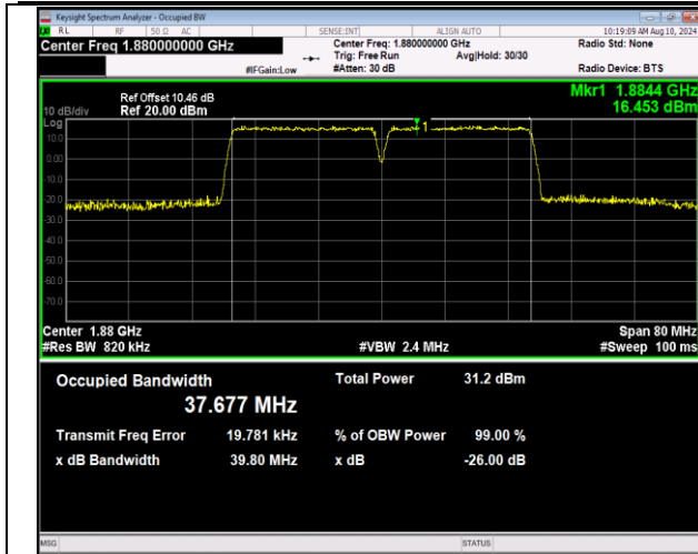
2-2-20MHz-20MHz-QPSK-QPSK-18801-18999-100RB#0-100RB#0-PASS
