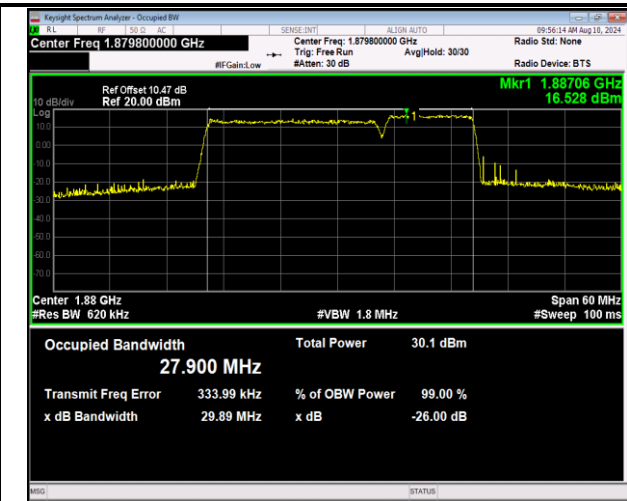
2-2-20MHz-10MHz-16QAM-16QAM-18851-18995-100RB#0-50RB#0-PASS
