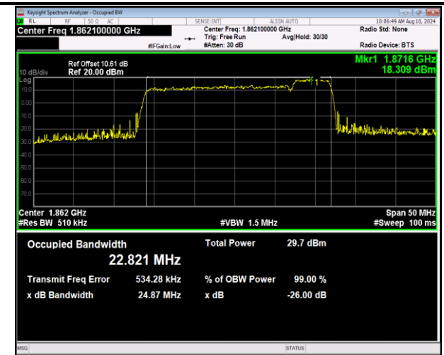
2-2-20MHz-5MHz-16QAM-16QAM-18700-18817-100RB#0-2 -25RB#0-PASS
