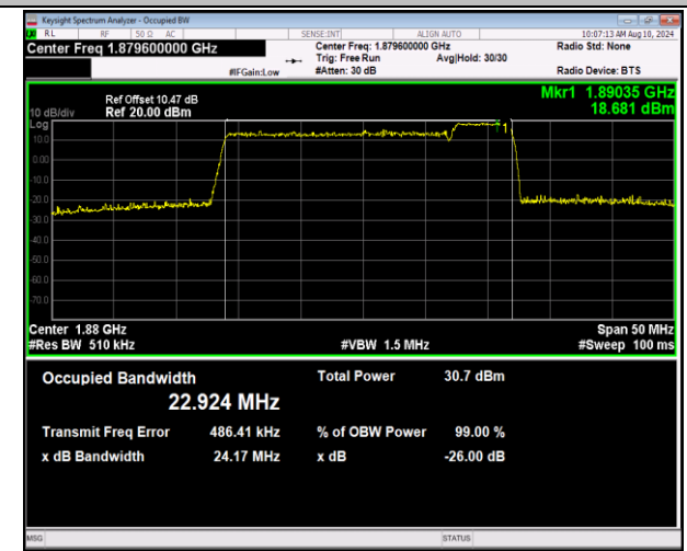
2-2-20MHz-5MHz-QPSK-QPSK-18875-18992-100RB#0-2 5RB#0-PASS
