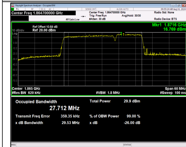
2-2-20MHz-10MHz-16QAM-16QAM-18700-18844-100RB# 0-50RB#0-PASS
