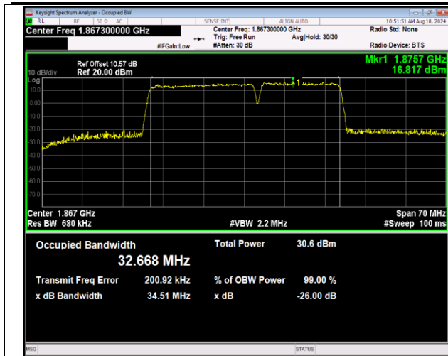
2-2-20MHz-15MHz-QPSK-QPSK-18700-18871-100RB#0-75RB#0-PASS
