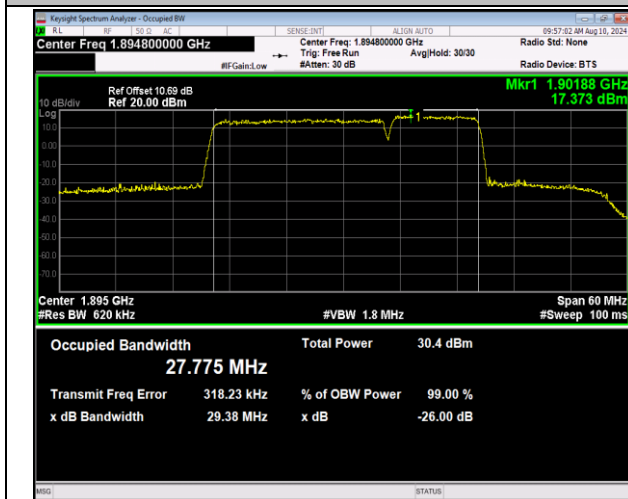
2-2-20MHz-10MHz-16QAM-16QAM-19001-19145-100RB#0-50RB#0-PASS
