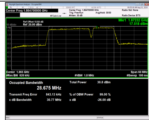
2-2-20MHz-10MHz-QPSK-QPSK-18700-18844-100RB#0- 50RB#0-PASS
