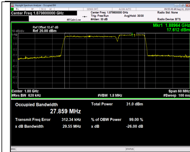
2-2-20MHz-10MHz-QPSK-QPSK-18851-18995-100RB#0-50RB#0-PASS
