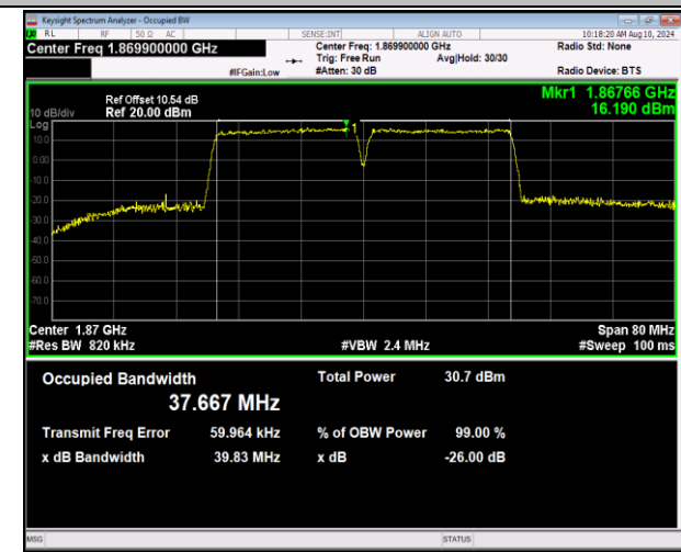
2-2-20MHz-20MHz-QPSK-QPSK-18700-18898-100RB#0-100RB#0-PASS
