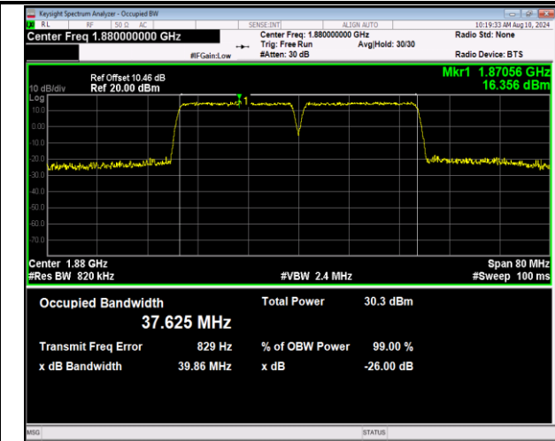
2-2-20MHz-20MHz-16QAM-16QAM-18801-18999-100RB#0-100RB#0-PASS
