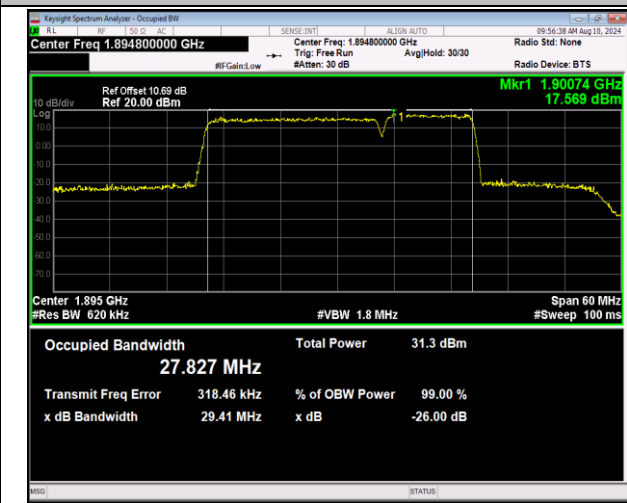
2-2-20MHz-10MHz-QPSK-QPSK-19001-19145-100RB#0-50RB#0-PASS
