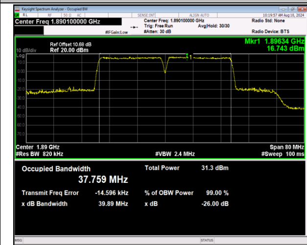
2-2-20MHz-20MHz-QPSK-QPSK-18902-19100-100RB#0-100RB#0-PASS
