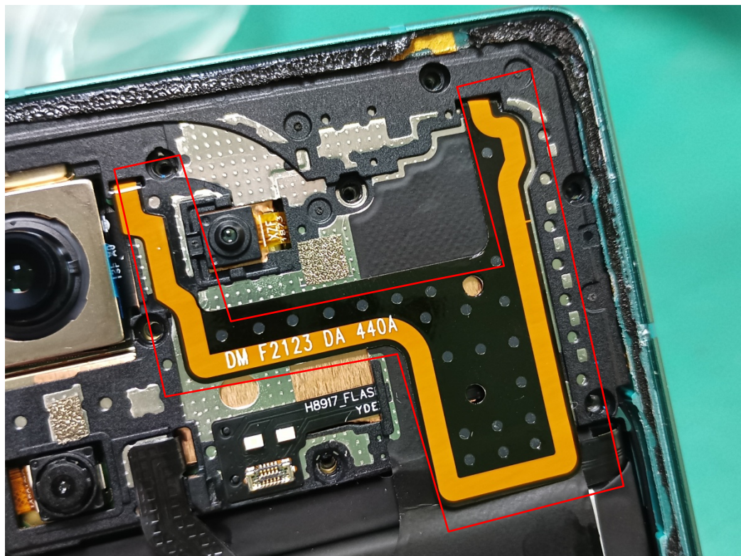
NFC ANT
