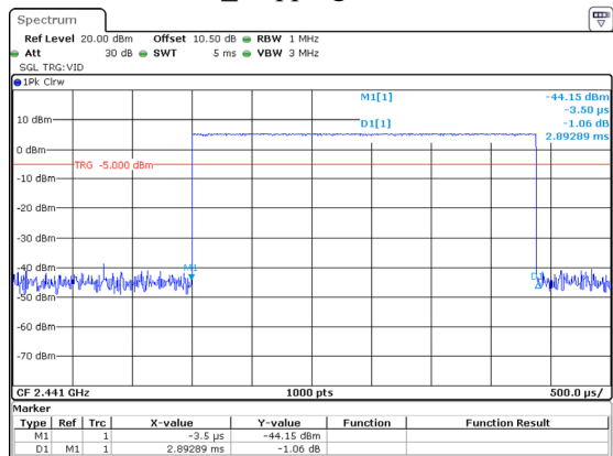
DH5_Hopping 2.893ms
