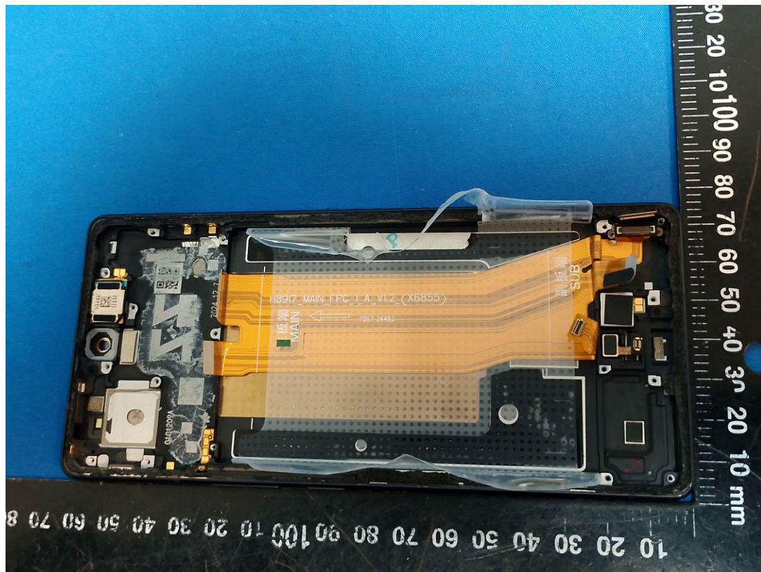
WWAN Antenna(ANT 0)
