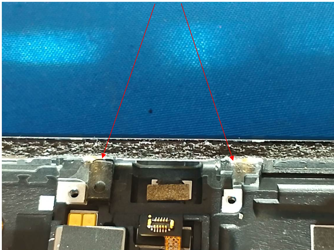
WWAN Antenna(ANT 0)
