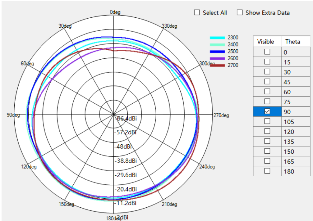
LTE B7/40Theta=90deg
