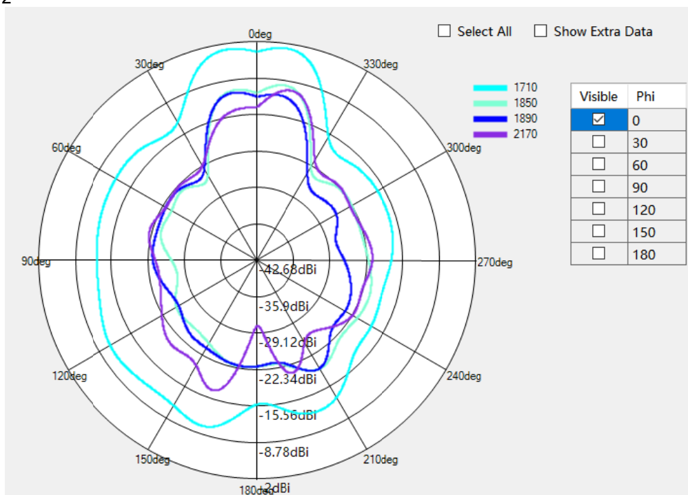
LTE B2/3 Phi=0deg
