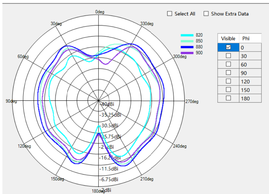
GSM850/WCDMA B5/LTE B5/B26 Phi=0deg
