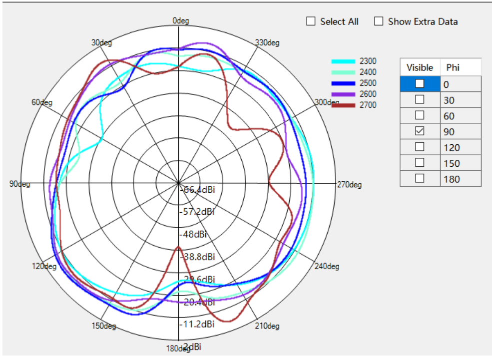
LTE B7/40Phi=90deg
