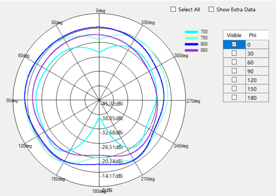
LTE B12/B13/B17/B28 Phi=0deg
