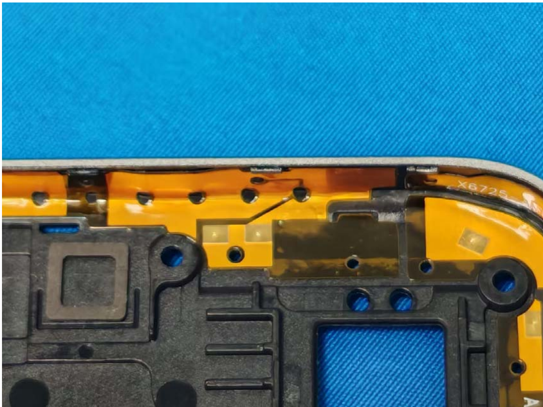
GPS Antenna(ANT 13)
