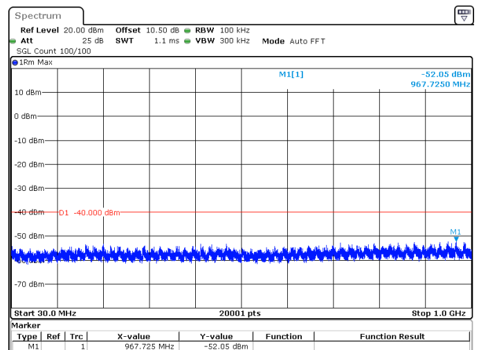
80MHz_30kHz_3660MHz_DFT-s-OFDM QPSK_RB216@0 -52.05 dBm
