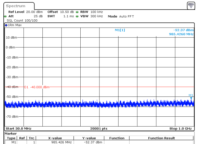
80MHz_30kHz_3660MHz_DFT-s-OFDM QPSK_RB1@216 -52.37 dBm
