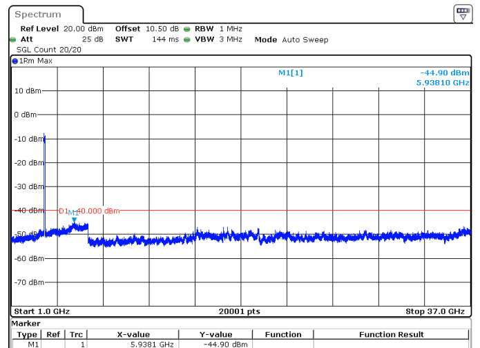
80MHz_30kHz_3590MHz_DFT-s-OFDM QPSK_RB216@0 -44.90 dBm
