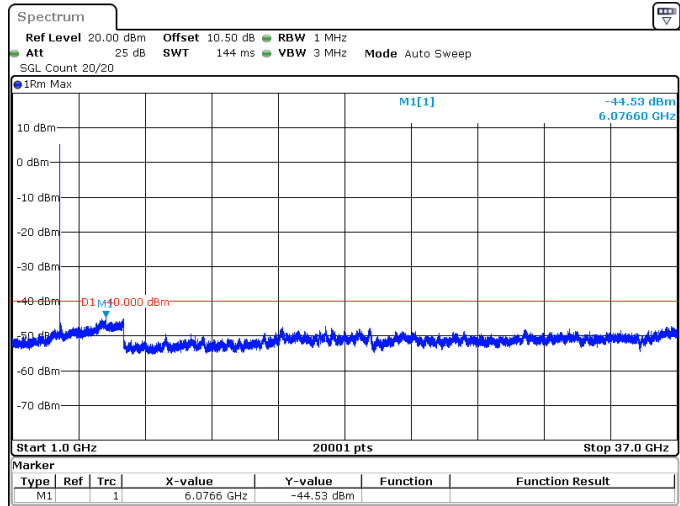
90MHz_30kHz_3595MHz_DFT-s-OFDM QPSK_RB1@0 -44.53 dBm
