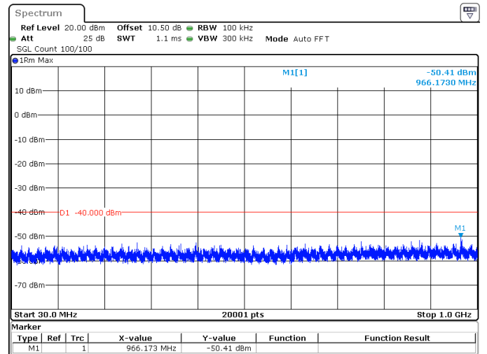
80MHz_30kHz_3660MHz_DFT-s-OFDM QPSK_RB1@0 -50.41 dBm
