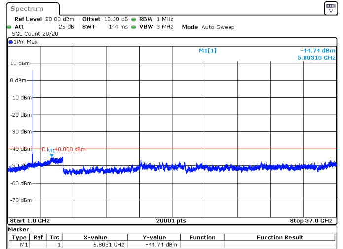
100MHz_30kHz_3650MHz_DFT-s-OFDM QPSK_RB1@272 -44.74 dBm
