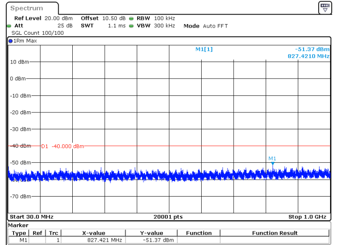
100MHz_30kHz_3650MHz_DFT-s-OFDM QPSK_RB1@0 -51.37 dBm
