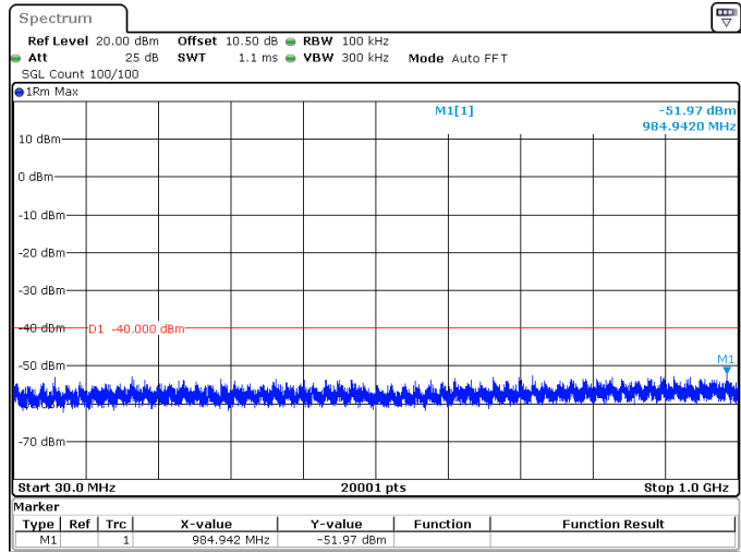
90MHz_30kHz_3595MHz_DFT-s-OFDM QPSK_RB243@0 -51.97 dBm
