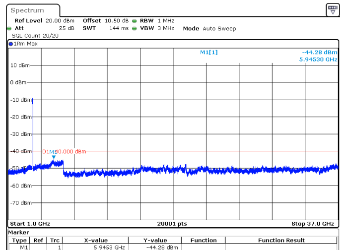
100MHz_30kHz_3650MHz_DFT-s-OFDM QPSK_RB270@0 -44.28 dBm
