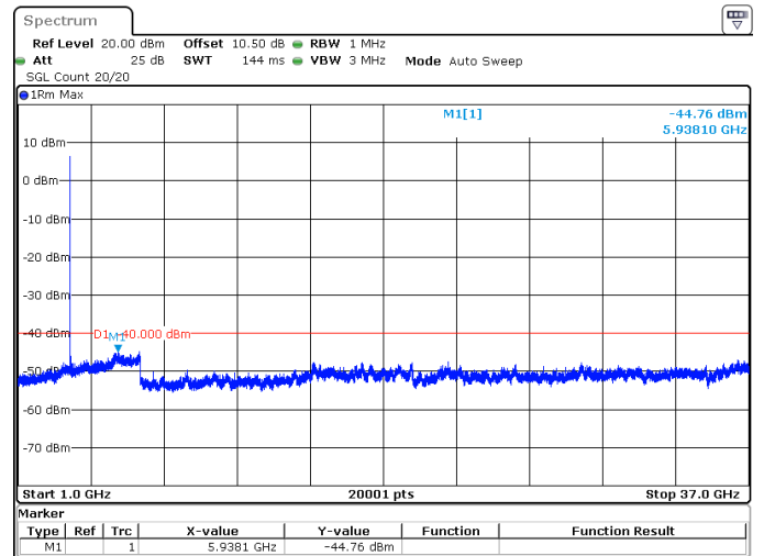
60MHz_30kHz_3580MHz_DFT-s-OFDM QPSK_RB1@0 -44.76 dBm
