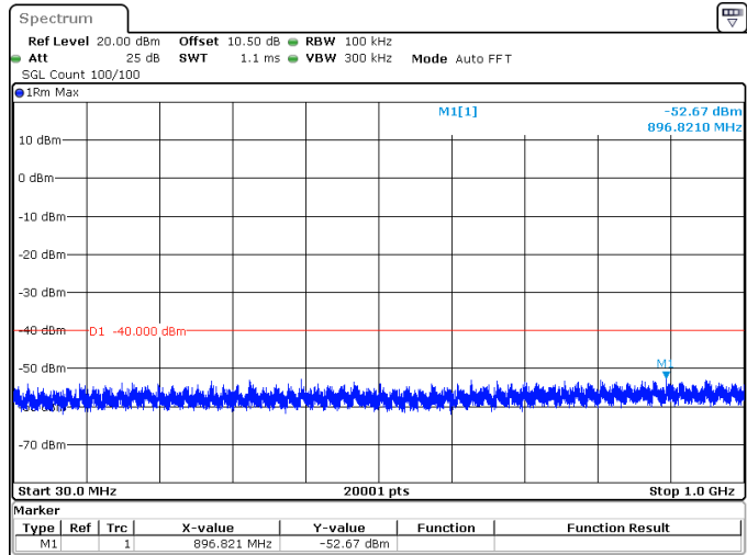
90MHz_30kHz_3595MHz_DFT-s-OFDM QPSK_RB1@0 -52.67 dBm
