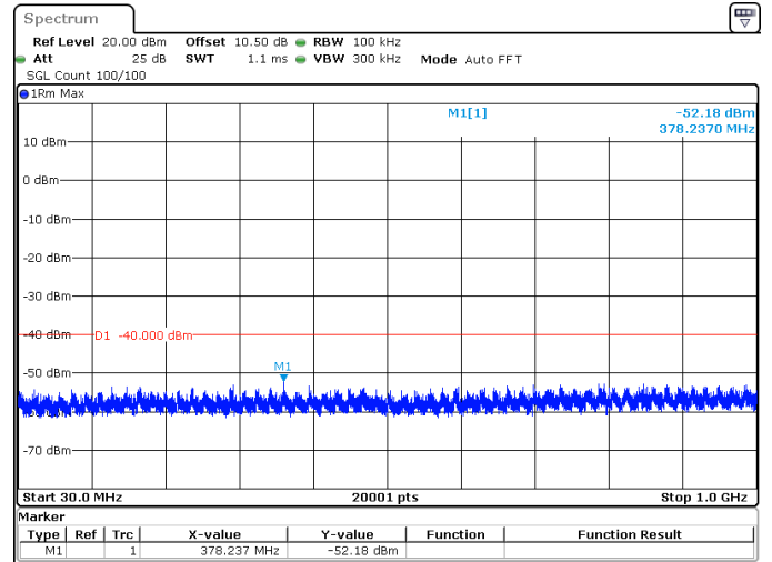
15MHz_30kHz_3625MHz_DFT-s-OFDM QPSK_RB1@0 -52.18 dBm
