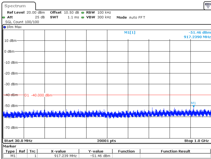
100MHz_30kHz_3600MHz_DFT-s-OFDM QPSK_RB270@0 -51.46 dBm
