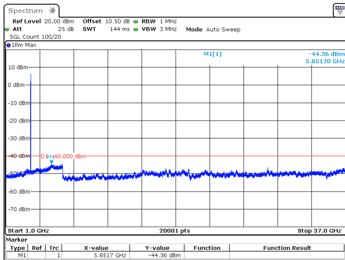
10MHz_30kHz_3625MHz_DFT-s-OFDM QPSK_RB1@0 -44.36 dBm
