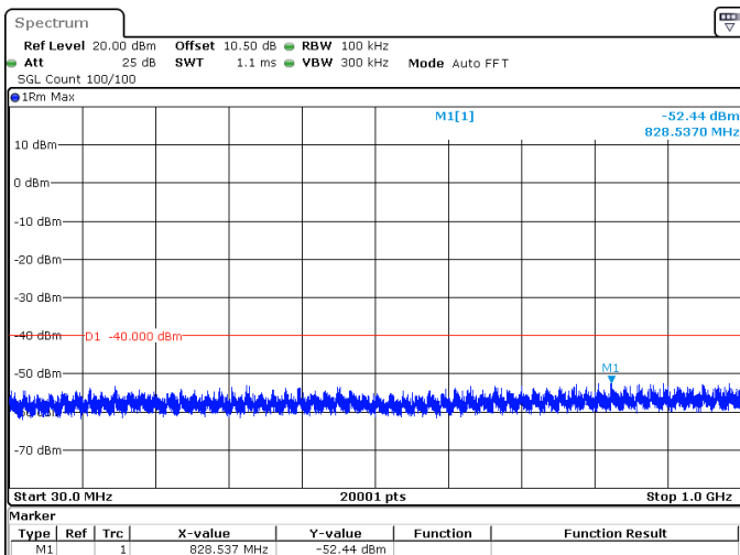
90MHz_30kHz_3625MHz_DFT-s-OFDM QPSK_RB1@244 -52.44 dBm
