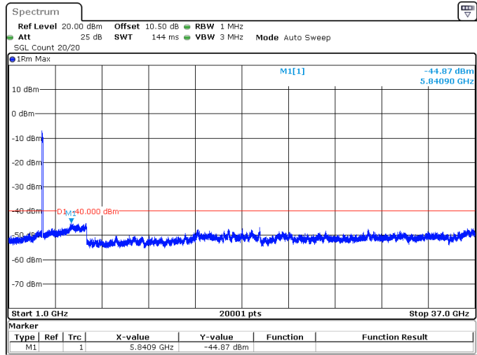
90MHz_30kHz_3595MHz_DFT-s-OFDM QPSK_RB243@0 -44.87 dBm
