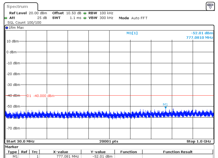
10MHz_30kHz_3555MHz_DFT-s-OFDM QPSK_RB24@0 -52.01 dBm
