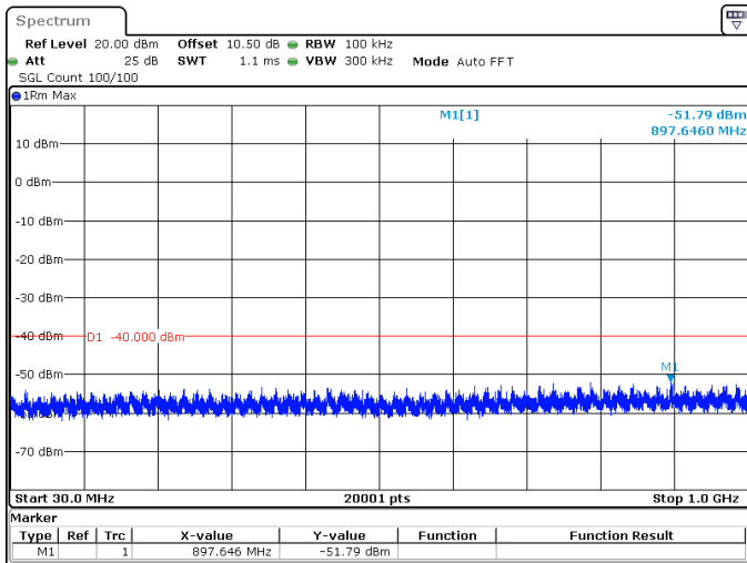
100MHz_30kHz_3625MHz_DFT-s-OFDM QPSK_RB270@0 -51.79 dBm
