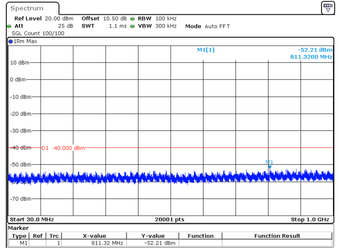
25MHz_30kHz_3625MHz_DFT-s-OFDM QPSK_RB1@0 -52.21 dBm
