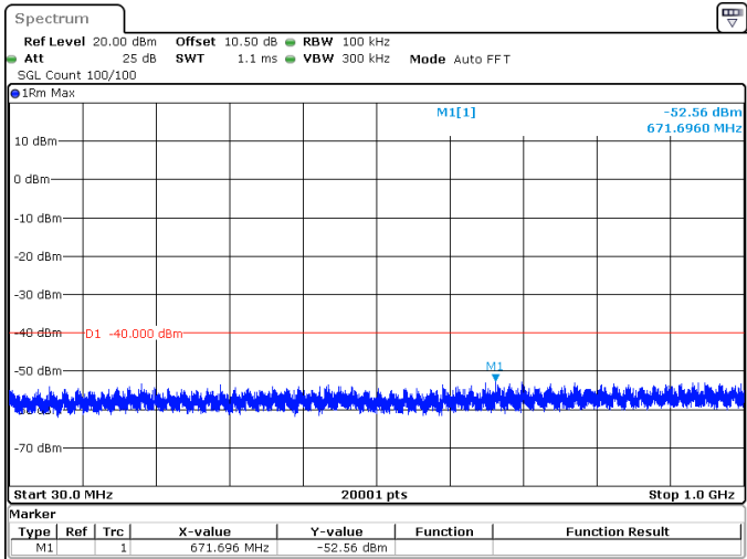
80MHz_30kHz_3660MHz_DFT-s-OFDM QPSK_RB216@0 -52.56 dBm
