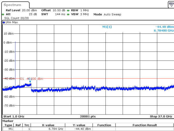
10MHz_30kHz_3695MHz_DFT-s-OFDM QPSK_RB24@0 -44.40 dBm
