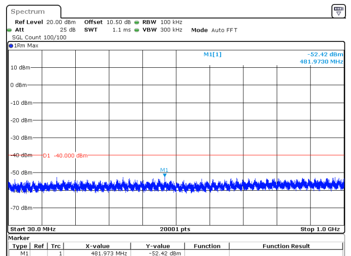
15MHz_15kHz_3692.5MHz_DFT-s-OFDM QPSK_RB75@0 -52.42 dBm
