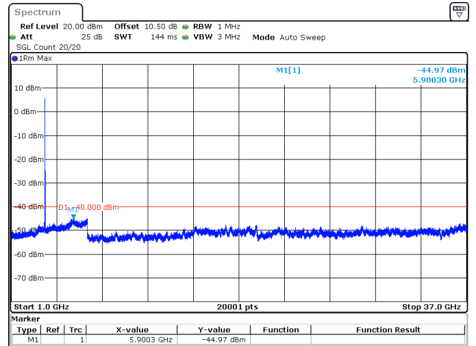
80MHz_30kHz_3625MHz_DFT-s-OFDM QPSK_RB1@216 -44.97 dBm
