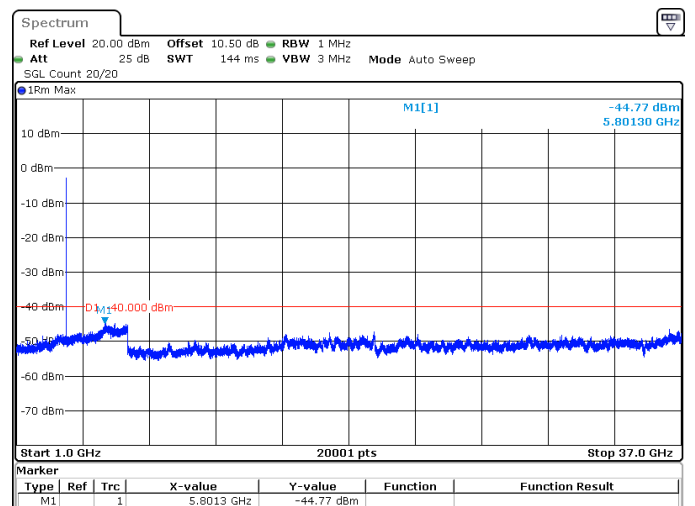
25MHz_30kHz_3687.5MHz_DFT-s-OFDM QPSK_RB64@0 -44.77 dBm
