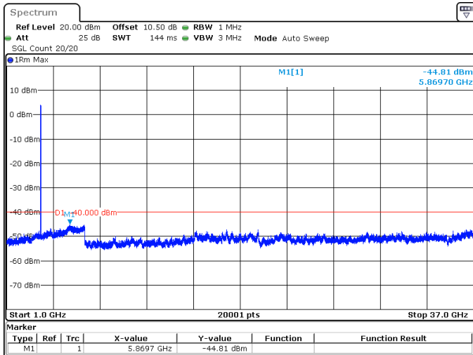
10MHz_15kHz_3625MHz_DFT-s-OFDM QPSK_RB1@0 -44.81 dBm
