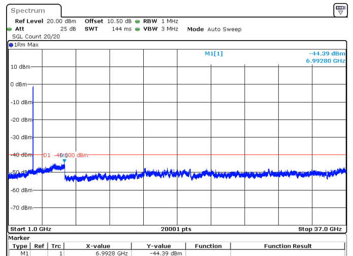
15MHz_15kHz_3625MHz_DFT-s-OFDM QPSK_RB75@0 -44.39 dBm
