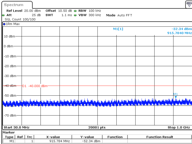
10MHz_15kHz_3625MHz_DFT-s-OFDM QPSK_RB50@0 -52.34 dBm
