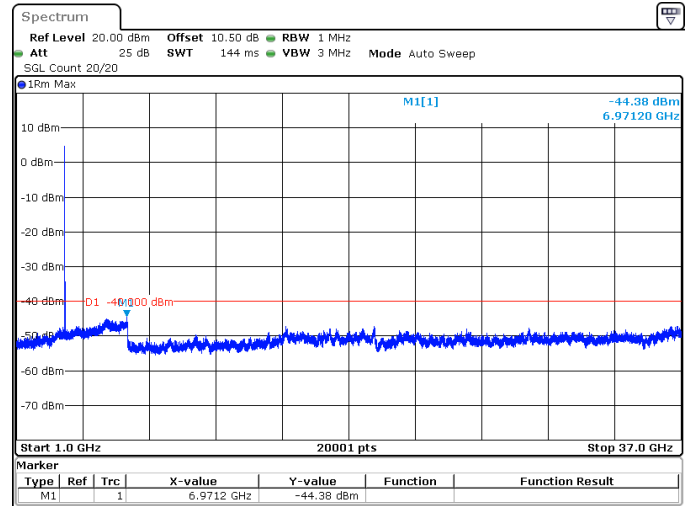
80MHz_30kHz_3625MHz_DFT-s-OFDM QPSK_RB1@0 -44.38 dBm
