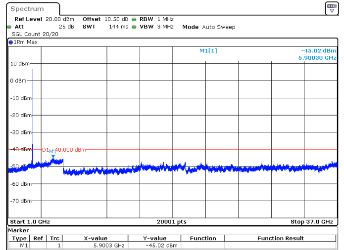
80MHz_30kHz_3660MHz_DFT-s-OFDM QPSK_RB1@216 -45.02 dBm
