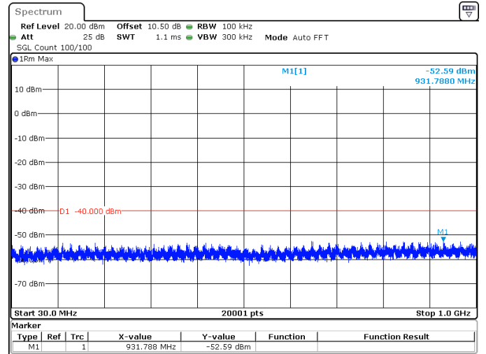
80MHz_30kHz_3660MHz_DFT-s-OFDM QPSK_RB1@0 -52.59 dBm
