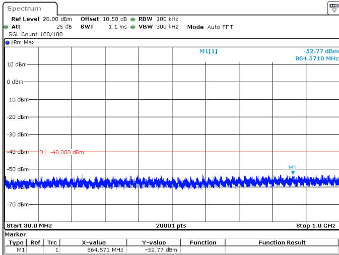
80MHz_30kHz_3590MHz_DFT-s-OFDM QPSK_RB216@0 -52.77 dBm
