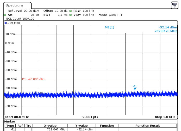
10MHz_30kHz_3695MHz_DFT-s-OFDM QPSK_RB1@23 -52.14 dBm
