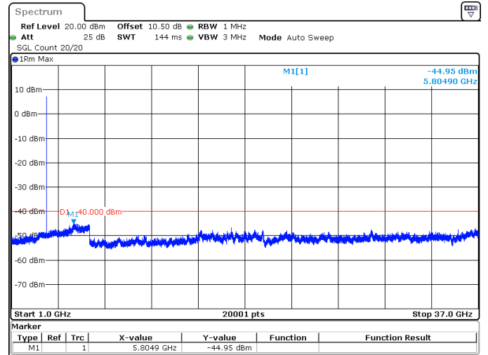
15MHz_30kHz_3692.5MHz_DFT-s-OFDM QPSK_RB1@0 -44.95 dBm
