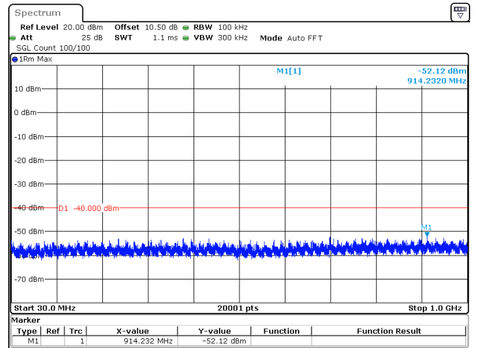
10MHz_30kHz_3625MHz_DFT-s-OFDM QPSK_RB1@0 -52.12 dBm
