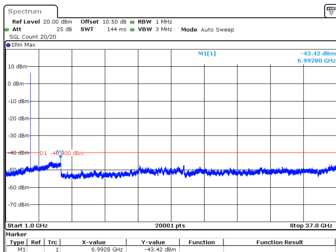
10MHz_30kHz_3695MHz_DFT-s-OFDM QPSK_RB1@23 -43.42 dBm
