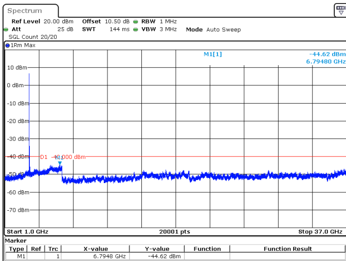
100MHz_30kHz_3600MHz_DFT-s-OFDM QPSK_RB1@0 -44.62 dBm
