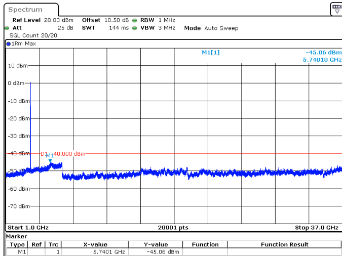
10MHz_30kHz_3625MHz_DFT-s-OFDM QPSK_RB24@0 -45.06 dBm
