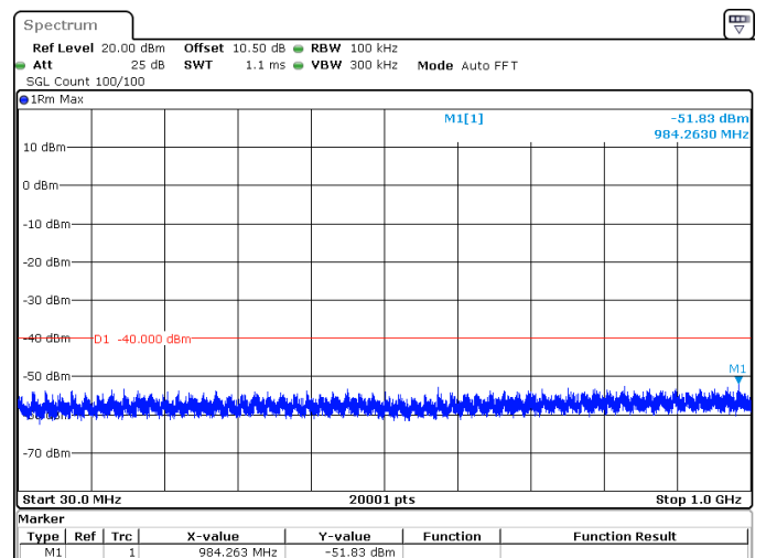
10MHz_30kHz_3625MHz_DFT-s-OFDM QPSK_RB24@0 -51.83 dBm
