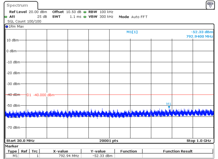
15MHz_15kHz_3625MHz_DFT-s-OFDM QPSK_RB1@0 -52.33 dBm
