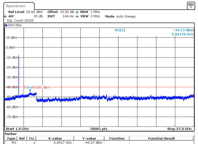
80MHz_30kHz_3660MHz_DFT-s-OFDM QPSK_RB216@0 -44.27 dBm
