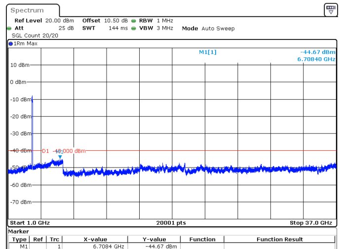
90MHz_30kHz_3625MHz_DFT-s-OFDM QPSK_RB243@0 -44.67 dBm
