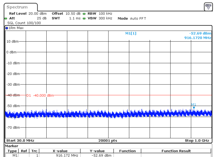
30MHz_30kHz_3565MHz_DFT-s-OFDM QPSK_RB75@0 -52.69 dBm
