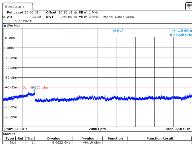
10MHz_30kHz_3625MHz_DFT-s-OFDM QPSK_RB1@23 -44.19 dBm
