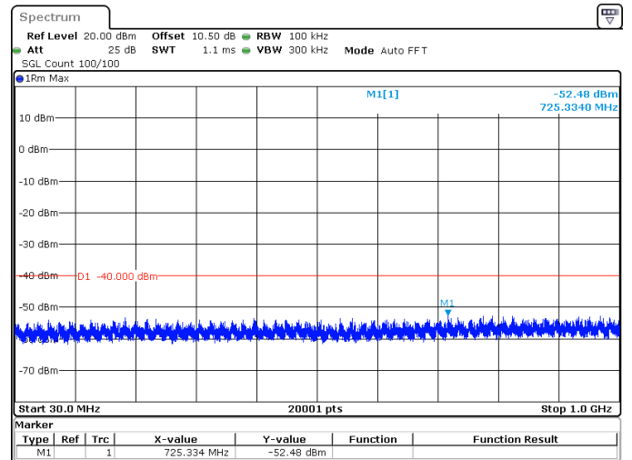
10MHz_30kHz_3695MHz_DFT-s-OFDM QPSK_RB1@0 -52.48 dBm
