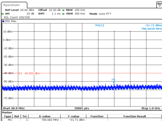
80MHz_30kHz_3660MHz_DFT-s-OFDM QPSK_RB1@216 -51.71 dBm
