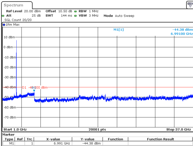
80MHz_30kHz_3660MHz_DFT-s-OFDM QPSK_RB1@0 -44.38 dBm
