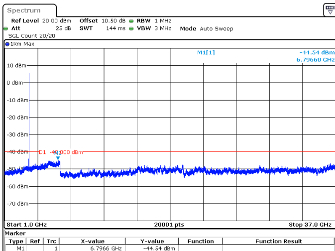
25MHz_30kHz_3625MHz_DFT-s-OFDM QPSK_RB1@64 -44.54 dBm
