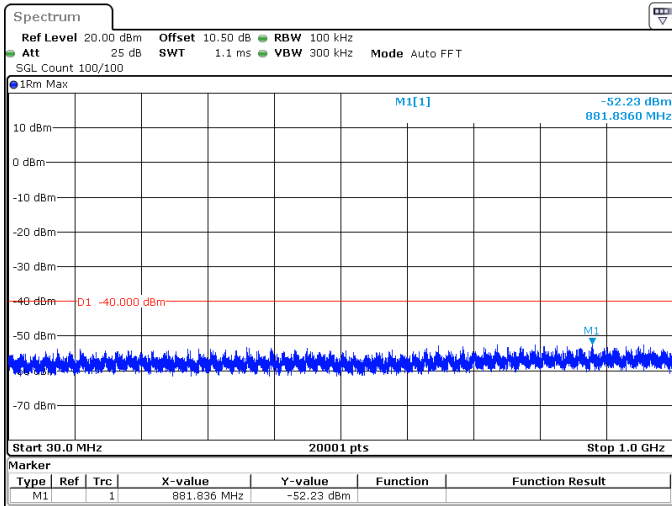
90MHz_30kHz_3595MHz_DFT-s-OFDM QPSK_RB243@0 -52.23 dBm
