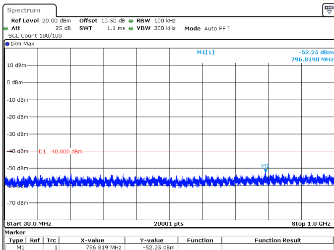
10MHz_15kHz_3695MHz_DFT-s-OFDM QPSK_RB1@51 -52.25 dBm
