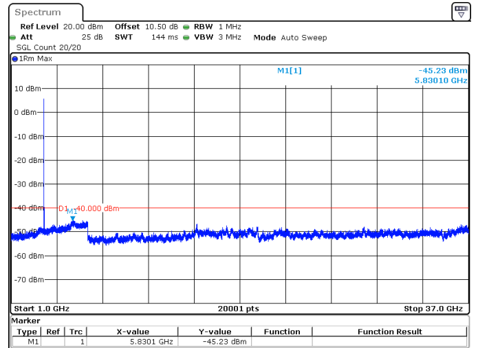
10MHz_30kHz_3555MHz_DFT-s-OFDM QPSK_RB1@23 -45.23 dBm
