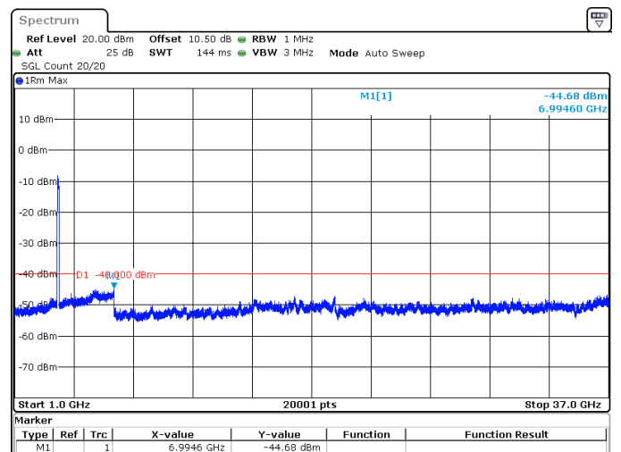
100MHz_30kHz_3625MHz_DFT-s-OFDM QPSK_RB270@0 -44.68 dBm
