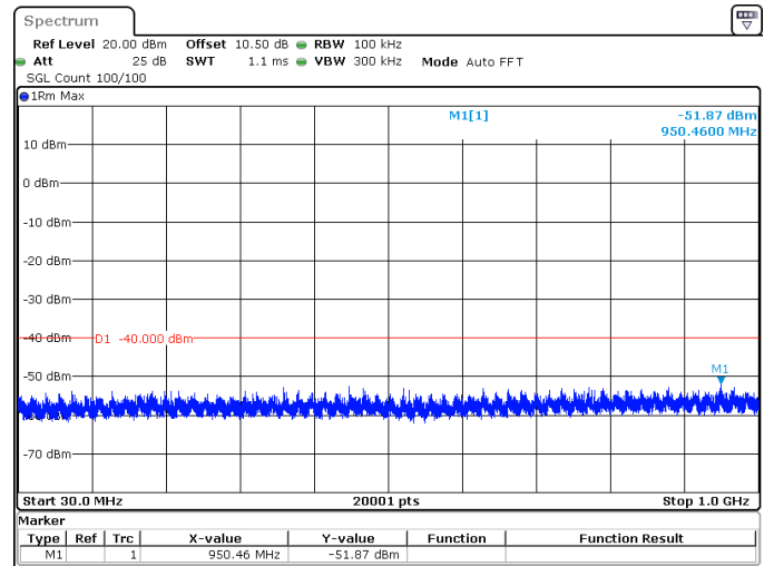
15MHz_15kHz_3692.5MHz_DFT-s-OFDM QPSK_RB1@0 -51.87 dBm
