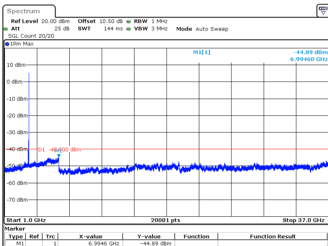
100MHz_30kHz_3650MHz_DFT-s-OFDM QPSK_RB1@272 -44.89 dBm
