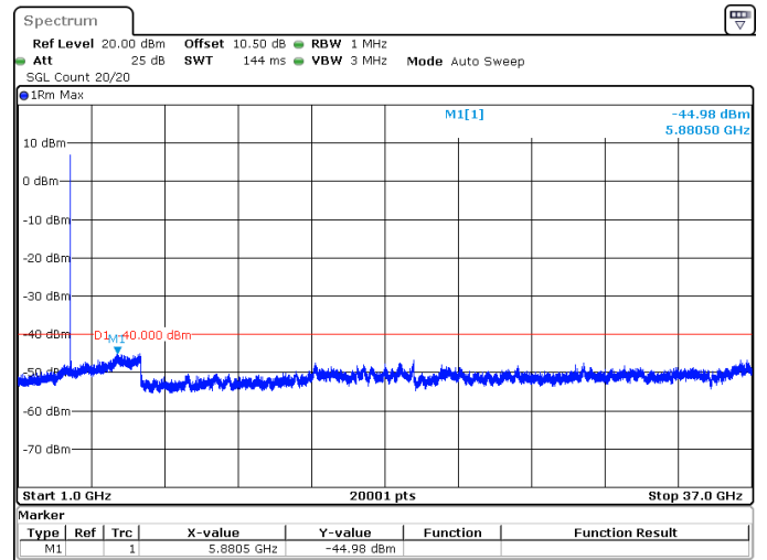
30MHz_30kHz_3565MHz_DFT-s-OFDM QPSK_RB1@0 -44.98 dBm
