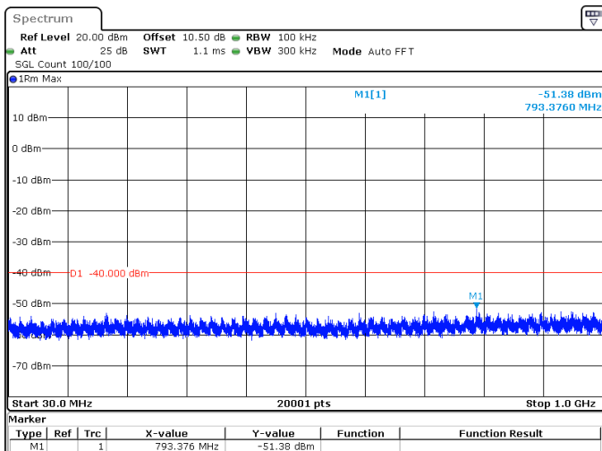
10MHz_30kHz_3555MHz_DFT-s-OFDM QPSK_RB1@23 -51.38 dBm
