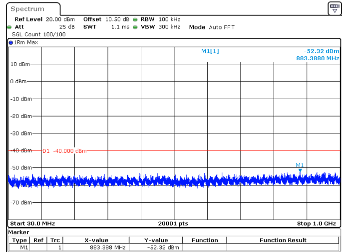
25MHz_30kHz_3625MHz_DFT-s-OFDM QPSK_RB1@64 -52.32 dBm
