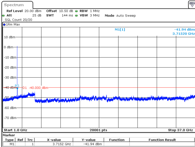
10MHz_15kHz_3695MHz_DFT-s-OFDM QPSK_RB50@0 -41.94 dBm
