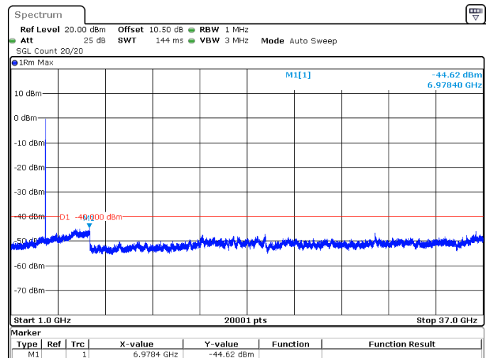
10MHz_15kHz_3625MHz_DFT-s-OFDM QPSK_RB50@0 -44.62 dBm
