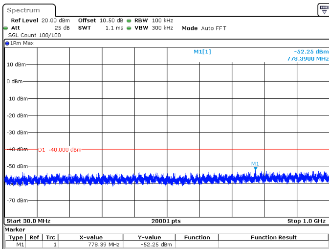
100MHz_30kHz_3650MHz_DFT-s-OFDM QPSK_RB1@0 -52.25 dBm
