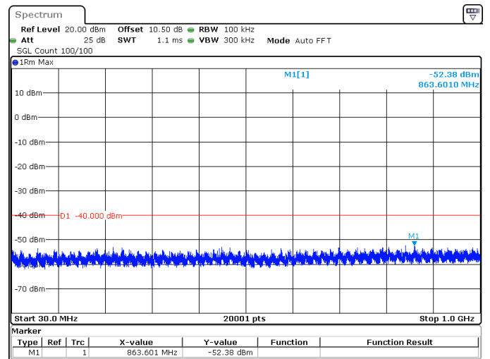
10MHz_30kHz_3625MHz_DFT-s-OFDM QPSK_RB1@23 -52.38 dBm
