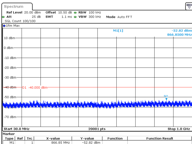
100MHz_30kHz_3600MHz_DFT-s-OFDM QPSK_RB1@272 -52.82 dBm
