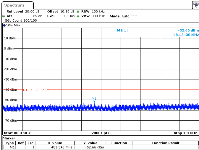
10MHz_30kHz_3555MHz_DFT-s-OFDM QPSK_RB1@0 -52.66 dBm
