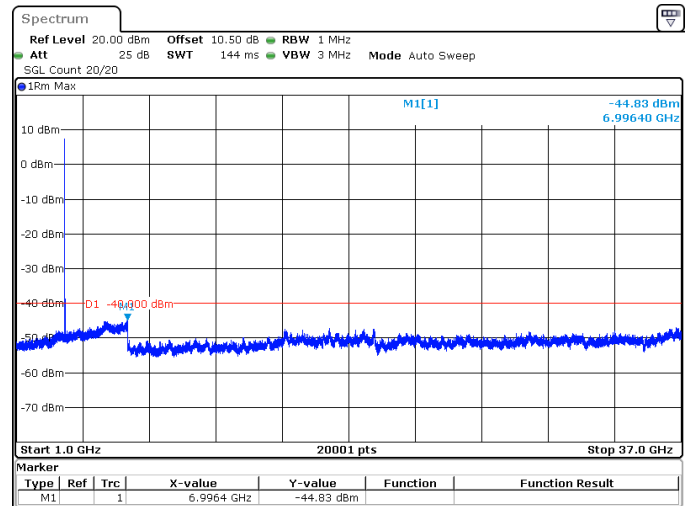
30MHz_15kHz_3625MHz_DFT-s-OFDM QPSK_RB1@0 -44.83 dBm
