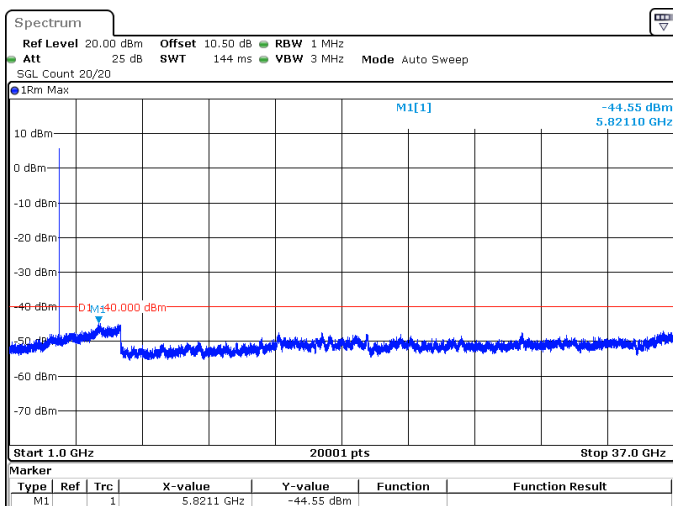
25MHz_30kHz_3687.5MHz_DFT-s-OFDM QPSK_RB1@64 -44.55 dBm
