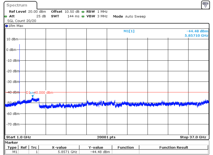
10MHz_30kHz_3555MHz_DFT-s-OFDM QPSK_RB1@0 -44.48 dBm
