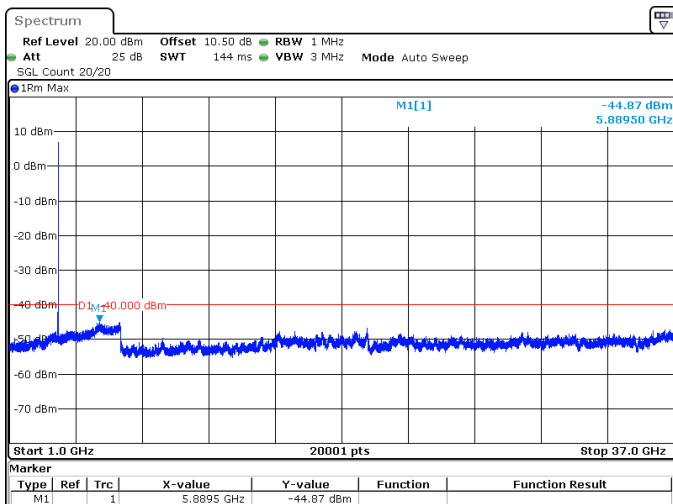
10MHz_15kHz_3625MHz_DFT-s-OFDM QPSK_RB1@51 -44.87 dBm
