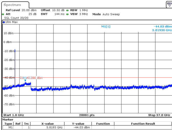
90MHz_30kHz_3655MHz_DFT-s-OFDM QPSK_RB243@0 -44.03 dBm
