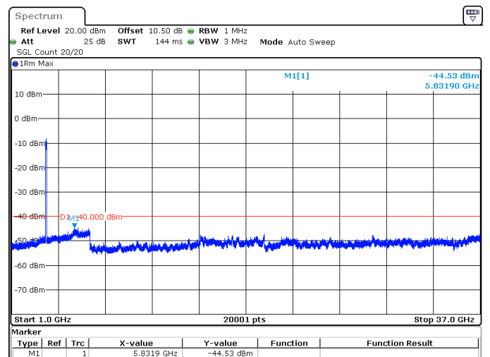
100MHz_30kHz_3650MHz_DFT-s-OFDM QPSK_RB270@0 -44.53 dBm
