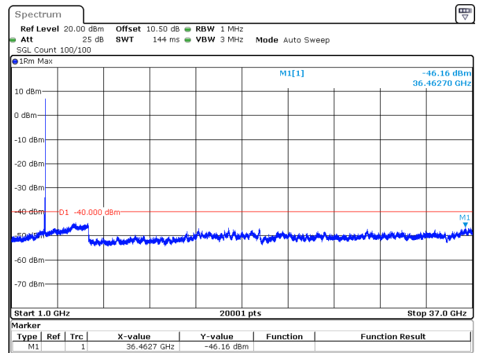
100MHz_30kHz_3600MHz_DFT-s-OFDM QPSK_RB1@272 -46.16 dBm
