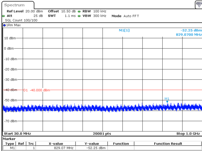
10MHz_15kHz_3555MHz_DFT-s-OFDM QPSK_RB50@0 -52.25 dBm
