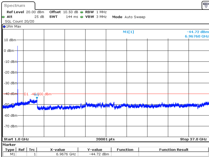
90MHz_30kHz_3625MHz_DFT-s-OFDM QPSK_RB1@0 -44.72 dBm
