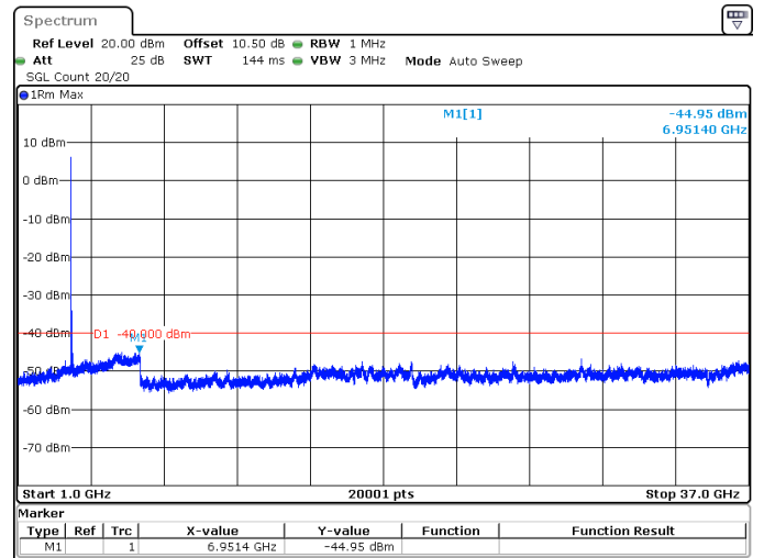
100MHz_30kHz_3650MHz_DFT-s-OFDM QPSK_RB1@0 -44.95 dBm
