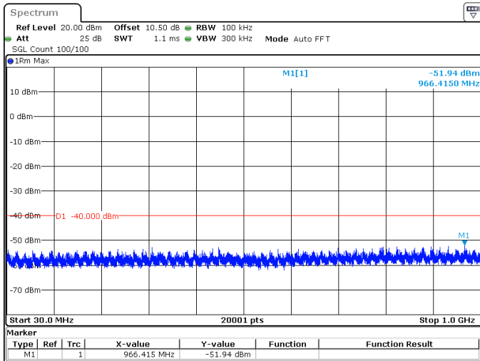
80MHz_30kHz_3625MHz_DFT-s-OFDM QPSK_RB1@0 -51.94 dBm
