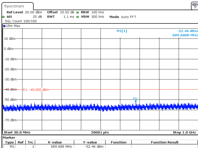
80MHz_30kHz_3625MHz_DFT-s-OFDM QPSK_RB1@216 -52.46 dBm
