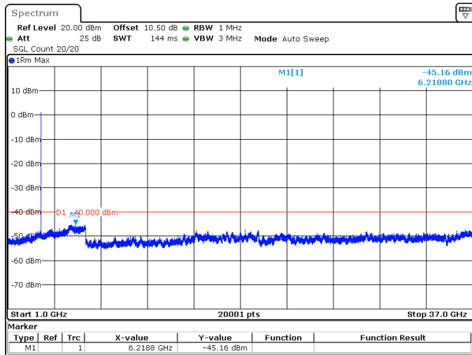
10MHz_30kHz_3555MHz_DFT-s-OFDM QPSK_RB24@0 -45.16 dBm
