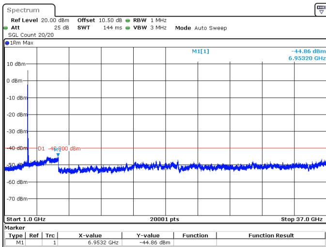
100MHz_30kHz_3625MHz_DFT-s-OFDM QPSK_RB1@0 -44.86 dBm
