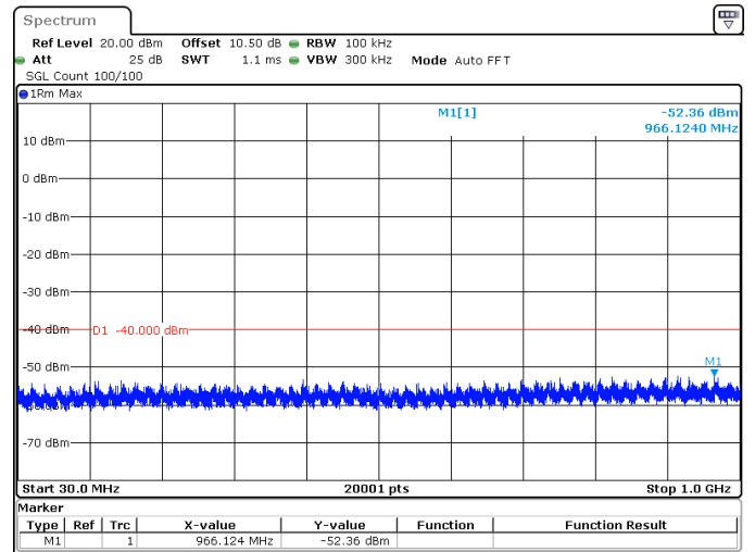
100MHz_30kHz_3600MHz_DFT-s-OFDM QPSK_RB1@0 -52.36 dBm
