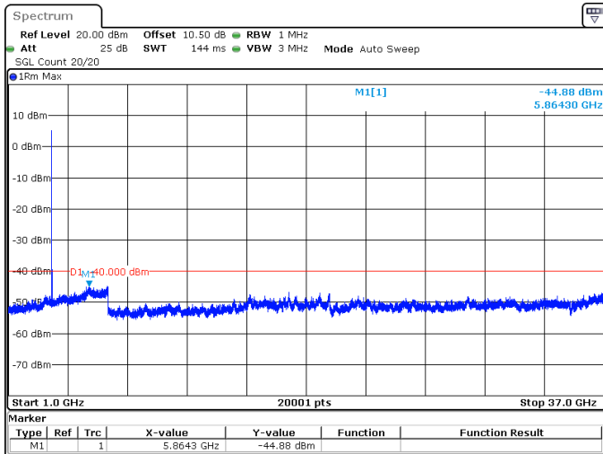
15MHz_30kHz_3625MHz_DFT-s-OFDM QPSK_RB1@0 -44.88 dBm
