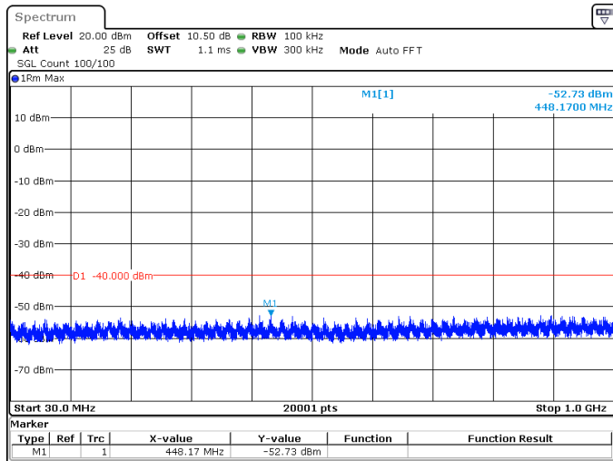
15MHz_15kHz_3625MHz_DFT-s-OFDM QPSK_RB75@0 -52.73 dBm
