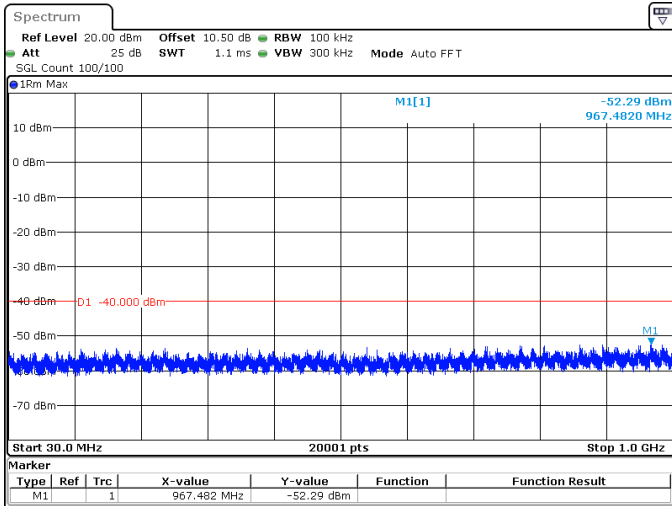
80MHz_30kHz_3625MHz_DFT-s-OFDM QPSK_RB216@0 -52.29 dBm
