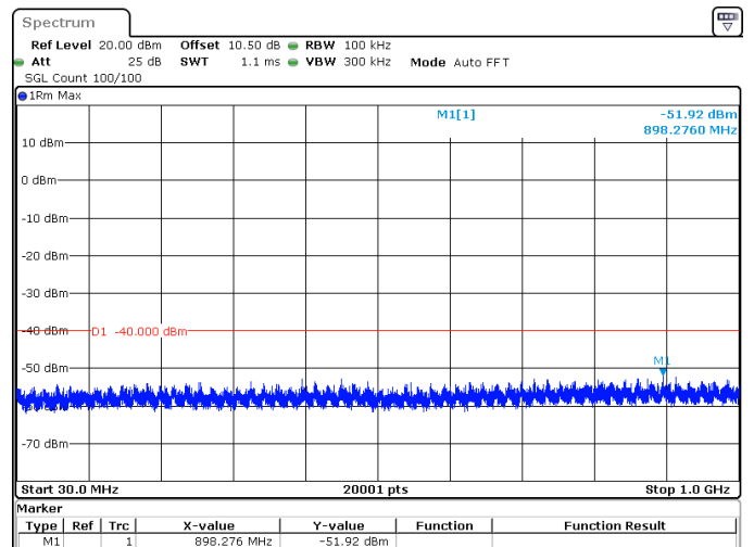
10MHz_15kHz_3695MHz_DFT-s-OFDM QPSK_RB50@0 -51.92 dBm
