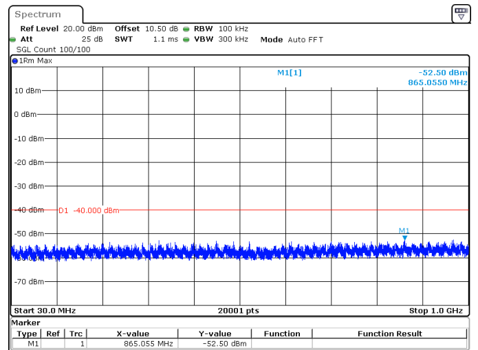
100MHz_30kHz_3650MHz_DFT-s-OFDM QPSK_RB1@272 -52.50 dBm
