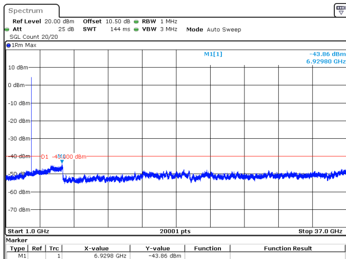
10MHz_30kHz_3695MHz_DFT-s-OFDM QPSK_RB1@0 -43.86 dBm
