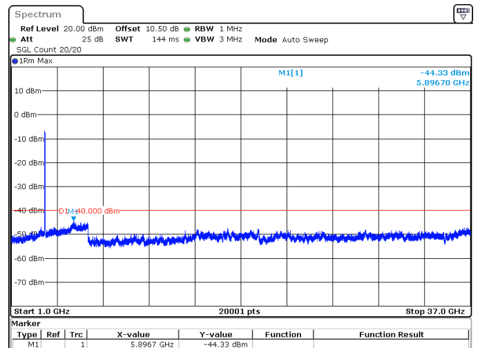
80MHz_30kHz_3625MHz_DFT-s-OFDM QPSK_RB216@0 -44.33 dBm
