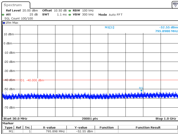
25MHz_30kHz_3625MHz_DFT-s-OFDM QPSK_RB64@0 -52.55 dBm
