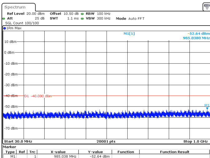
100MHz_30kHz_3625MHz_DFT-s-OFDM QPSK_RB1@272 -52.64 dBm
