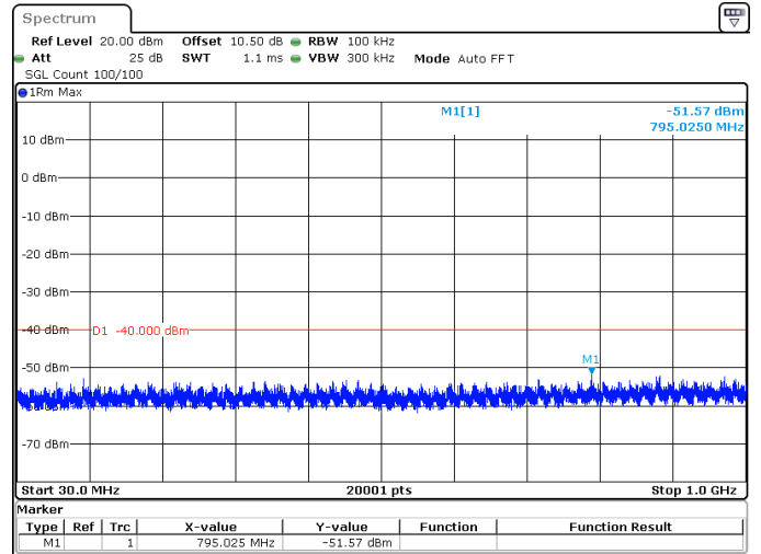
10MHz_15kHz_3695MHz_DFT-s-OFDM QPSK_RB1@0 -51.57 dBm
