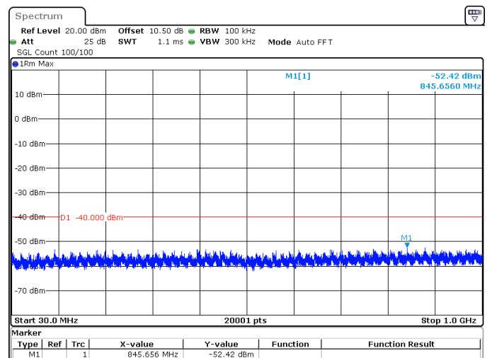
10MHz_30kHz_3695MHz_DFT-s-OFDM QPSK_RB24@0 -52.42 dBm
