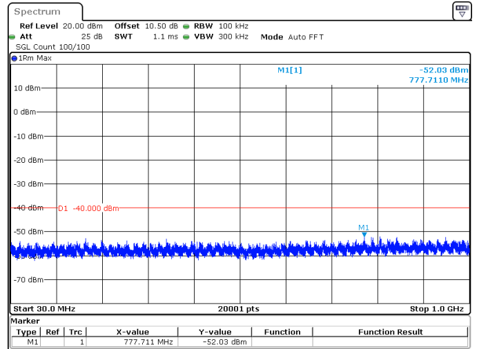
10MHz_15kHz_3625MHz_DFT-s-OFDM QPSK_RB1@0 -52.03 dBm
