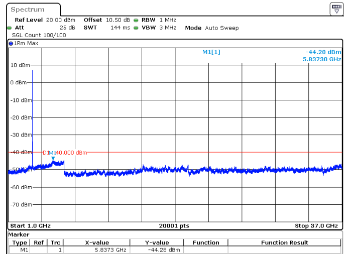
70MHz_30kHz_3625MHz_DFT-s-OFDM QPSK_RB1@0 -44.28 dBm
