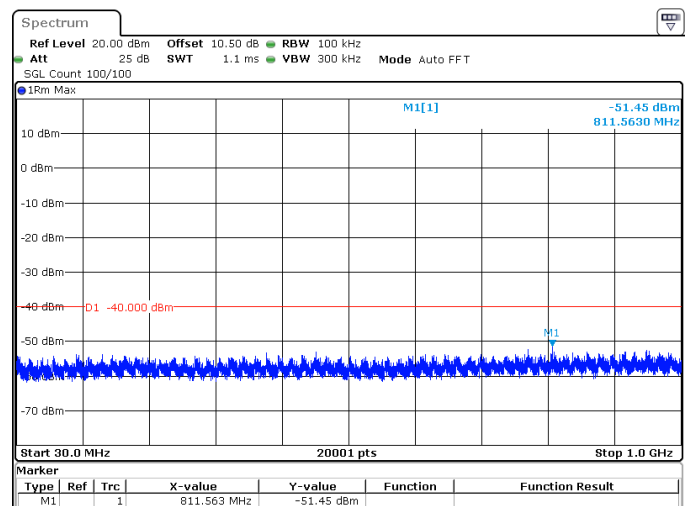
40MHz_30kHz_3625MHz_DFT-s-OFDM QPSK_RB100@0 -51.45 dBm
