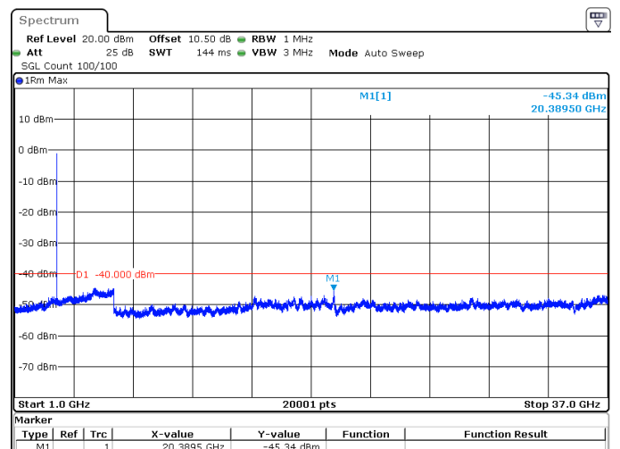
20MHz_30kHz_3560MHz_DFT-s-OFDM QPSK_RB50@0 -45.34 dBm
