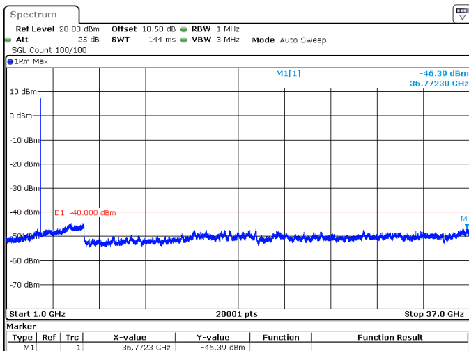
20MHz_30kHz_3625MHz_DFT-s-OFDM QPSK_RB1@50 -46.39 dBm
