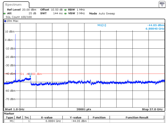
80MHz_30kHz_3590MHz_DFT-s-OFDM QPSK_RB1@0 -44.05 dBm
