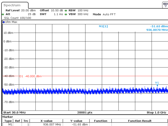
70MHz_30kHz_3625MHz_DFT-s-OFDM QPSK_RB1@0 -51.65 dBm
