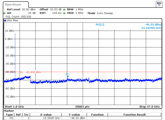
20MHz_30kHz_3560MHz_DFT-s-OFDM QPSK_RB1@0 -46.55 dBm
