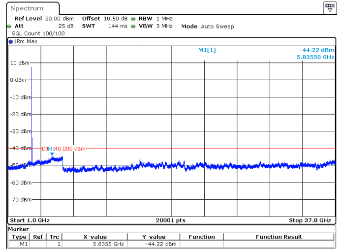
60MHz_30kHz_3625MHz_DFT-s-OFDM QPSK_RB1@0 -44.22 dBm
