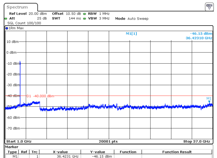
80MHz_30kHz_3590MHz_DFT-s-OFDM QPSK_RB216@0 -46.15 dBm
