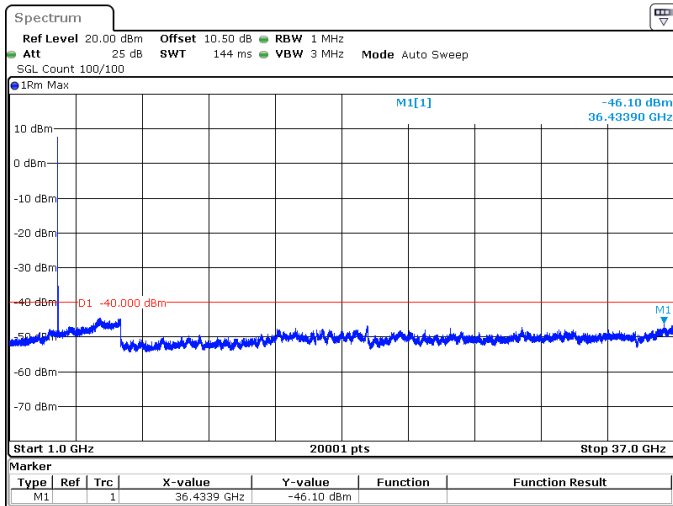
20MHz_30kHz_3625MHz_DFT-s-OFDM QPSK_RB1@0 -46.10 dBm
