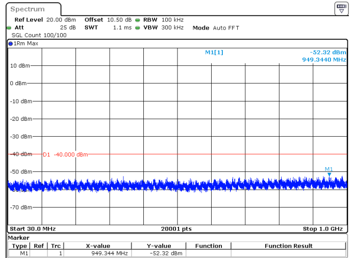
20MHz_30kHz_3625MHz_DFT-s-OFDM QPSK_RB1@50 -52.32 dBm
