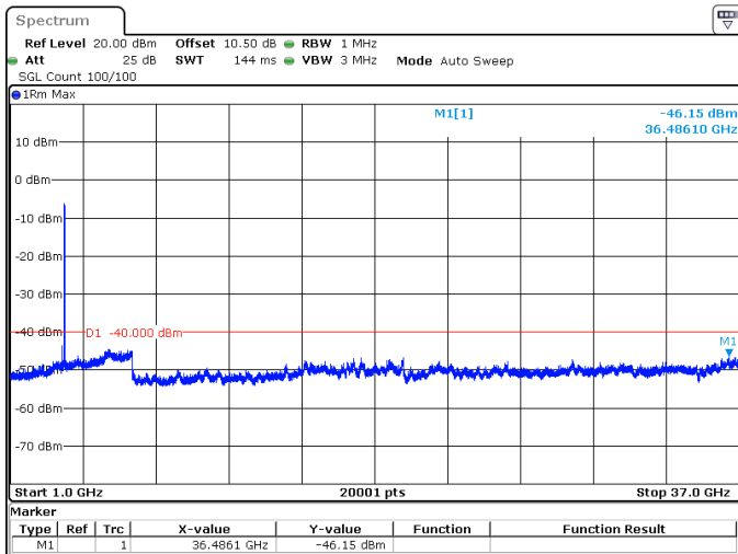
70MHz_30kHz_3665MHz_DFT-s-OFDM QPSK_RB180@0 -46.15 dBm
