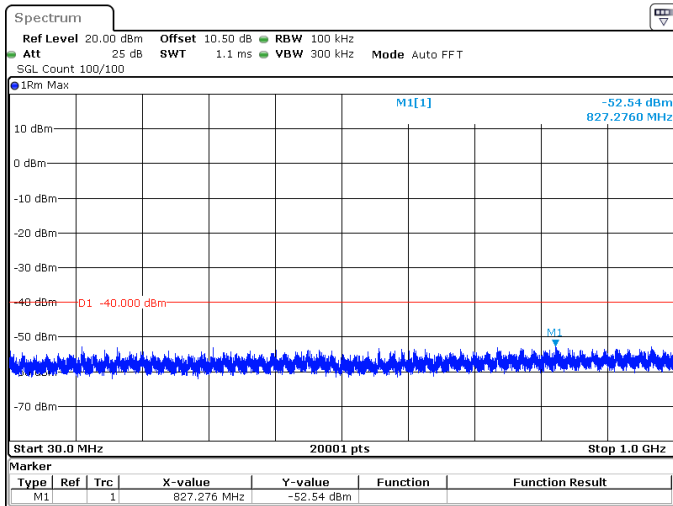
60MHz_30kHz_3625MHz_DFT-s-OFDM QPSK_RB1@0 -52.54 dBm
