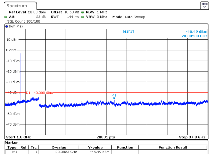
30MHz_15kHz_3685MHz_DFT-s-OFDM QPSK_RB160@0 -46.49 dBm
