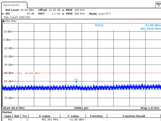
40MHz_30kHz_3625MHz_DFT-s-OFDM QPSK_RB1@0 -51.88 dBm
