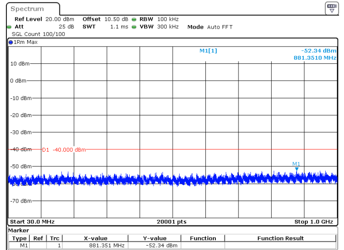
60MHz_30kHz_3625MHz_DFT-s-OFDM QPSK_RB1@161 -52.34 dBm
