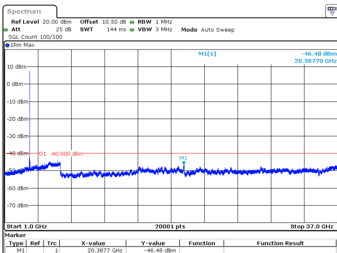
60MHz_30kHz_3670MHz_DFT-s-OFDM QPSK_RB1@161 -46.48 dBm
