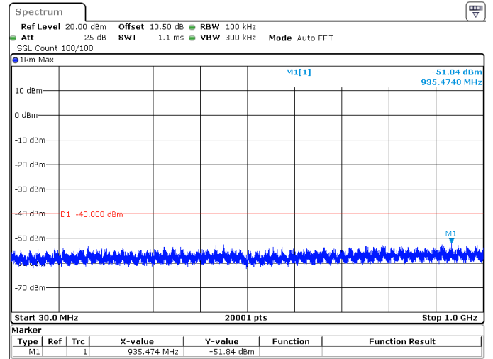
30MHz_15kHz_3685MHz_DFT-s-OFDM QPSK_RB1@0 -51.84 dBm
