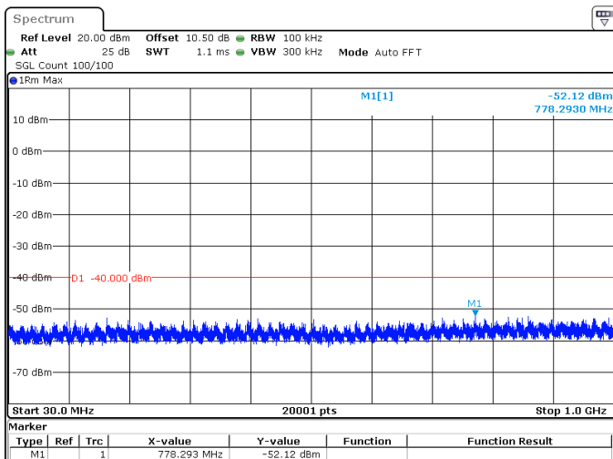
20MHz_15kHz_3560MHz_DFT-s-OFDM QPSK_RB1@105 -52.12 dBm
