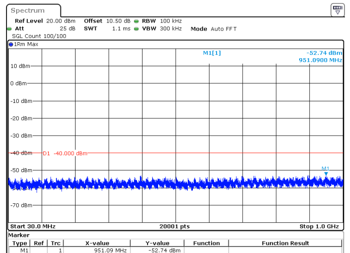
70MHz_30kHz_3585MHz_DFT-s-OFDM QPSK_RB180@0 -52.74 dBm
