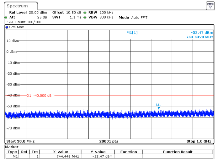
50MHz_15kHz_3675MHz_DFT-s-OFDM QPSK_RB1@0 -52.47 dBm
