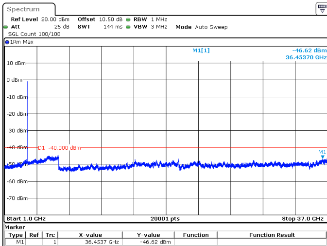
20MHz_15kHz_3560MHz_DFT-s-OFDM QPSK_RB100@0 -46.62 dBm
