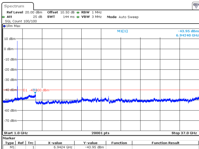
50MHz_15kHz_3675MHz_DFT-s-OFDM QPSK_RB1@0 -43.95 dBm
