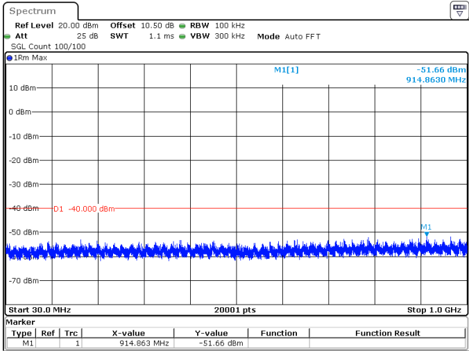
50MHz_30kHz_3625MHz_DFT-s-OFDM QPSK_RB1@0 -51.66 dBm
