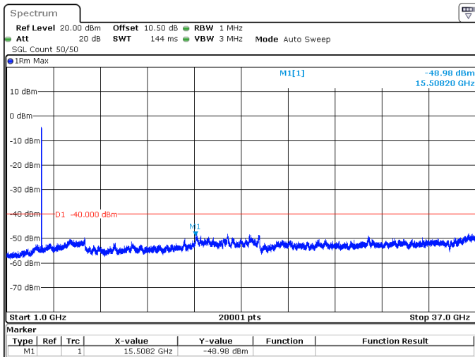
40MHz_15kHz_3680MHz_DFT-s-OFDM QPSK_RB216@0 -48.98 dBm
