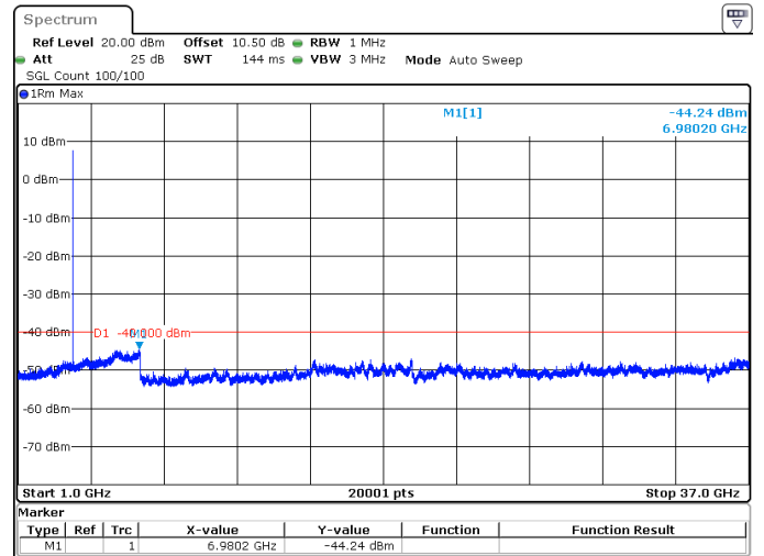
15MHz_30kHz_3692.5MHz_DFT-s-OFDM QPSK_RB1@37 -44.24 dBm
