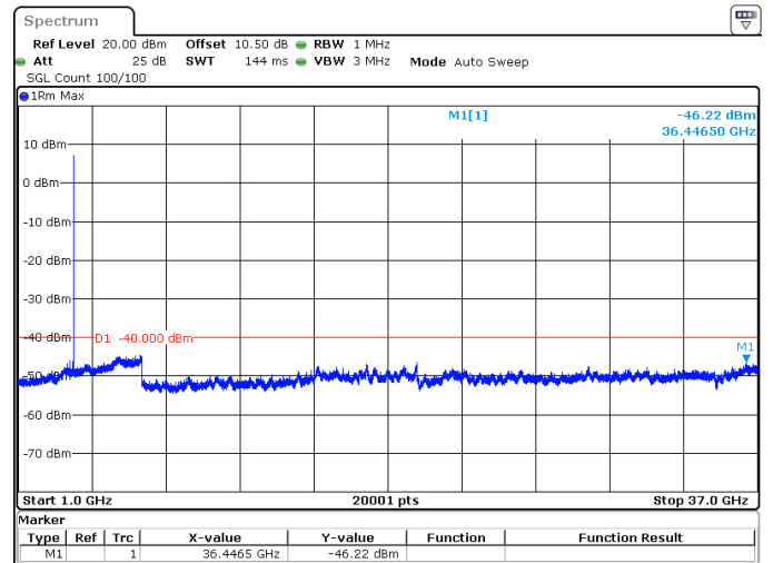
20MHz_30kHz_3690MHz_DFT-s-OFDM QPSK_RB1@0 -46.22 dBm
