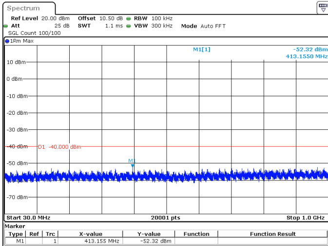
15MHz_30kHz_3692.5MHz_DFT-s-OFDM QPSK_RB36@0 -52.32 dBm
