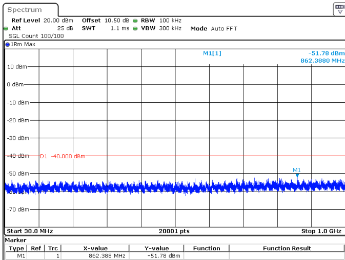
70MHz_30kHz_3625MHz_DFT-s-OFDM QPSK_RB180@0 -51.78 dBm
