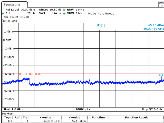
70MHz_30kHz_3585MHz_DFT-s-OFDM QPSK_RB180@0 -45.13 dBm
