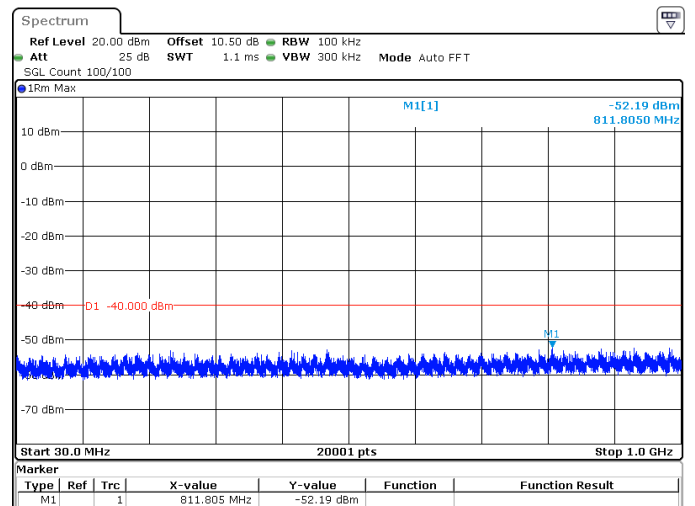
60MHz_30kHz_3670MHz_DFT-s-OFDM QPSK_RB1@161 -52.19 dBm
