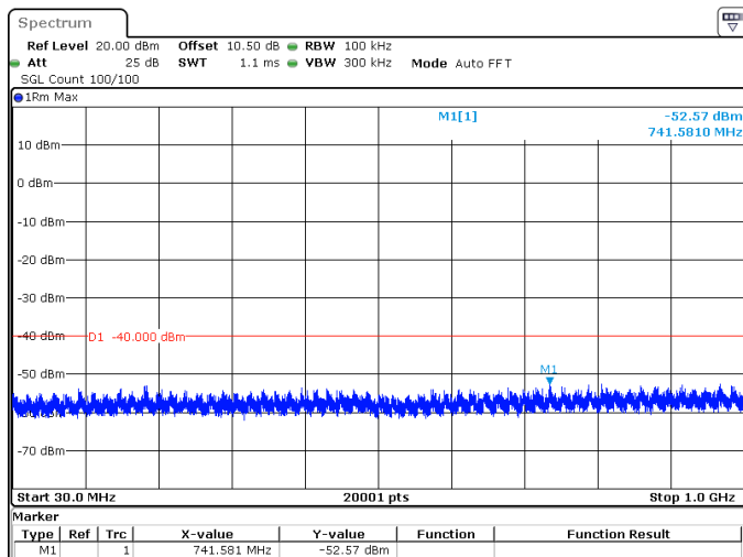
20MHz_30kHz_3690MHz_DFT-s-OFDM QPSK_RB1@0 -52.57 dBm
