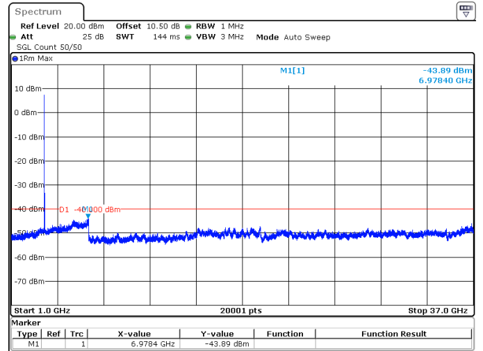
70MHz_30kHz_3585MHz_DFT-s-OFDM QPSK_RB1@0 -43.89 dBm
