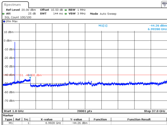
20MHz_30kHz_3625MHz_DFT-s-OFDM QPSK_RB50@0 -44.26 dBm
