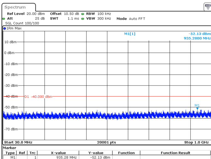
80MHz_30kHz_3590MHz_DFT-s-OFDM QPSK_RB1@216 -52.13 dBm
