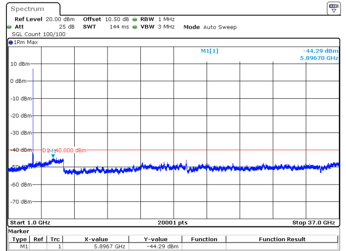
40MHz_15kHz_3680MHz_DFT-s-OFDM QPSK_RB1@215 -44.29 dBm
