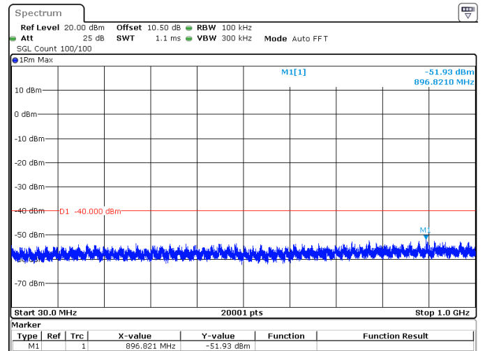
20MHz_15kHz_3690MHz_DFT-s-OFDM QPSK_RB100@0 -51.93 dBm
