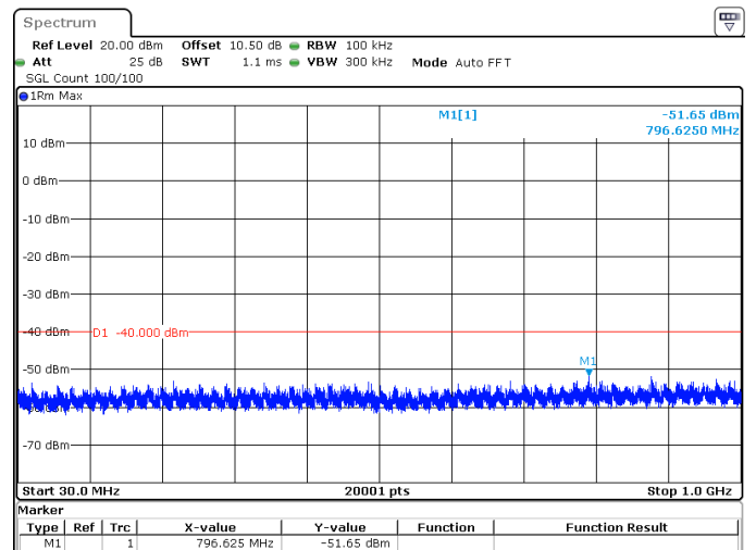
20MHz_15kHz_3625MHz_DFT-s-OFDM QPSK_RB1@105 -51.65 dBm
