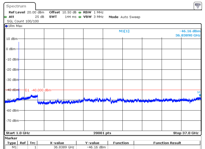
20MHz_30kHz_3560MHz_DFT-s-OFDM QPSK_RB1@50 -46.16 dBm
