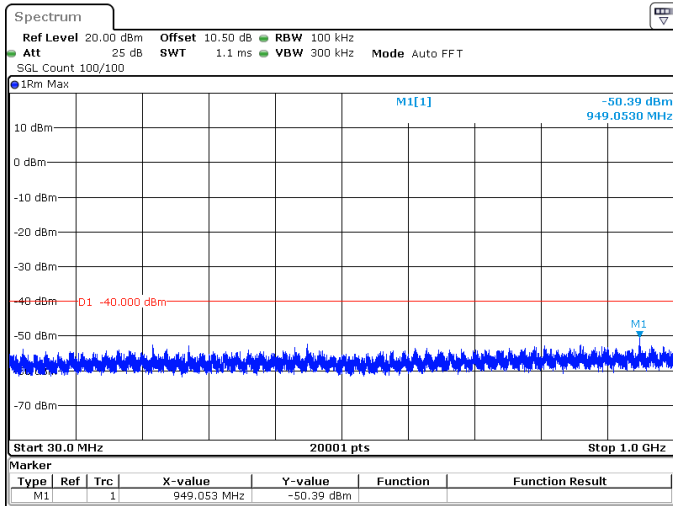
20MHz_30kHz_3560MHz_DFT-s-OFDM QPSK_RB50@0 -50.39 dBm
