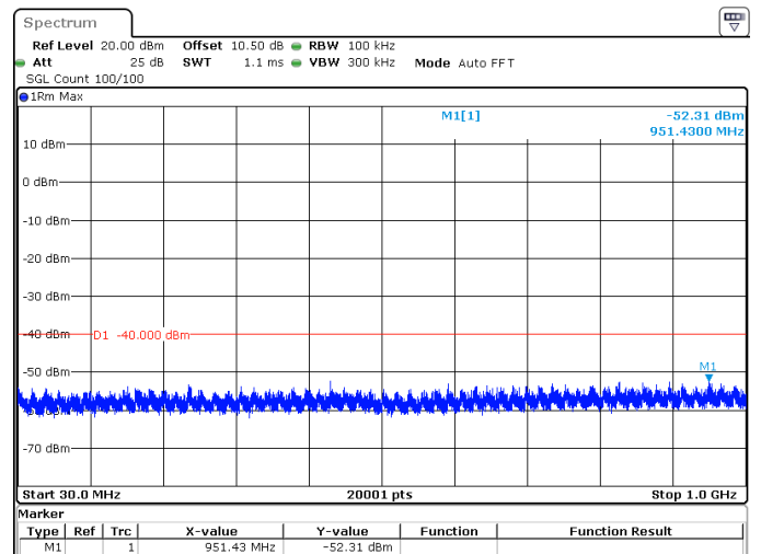
40MHz_30kHz_3625MHz_DFT-s-OFDM QPSK_RB1@105 -52.31 dBm
