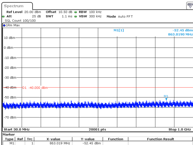
60MHz_30kHz_3580MHz_DFT-s-OFDM QPSK_RB1@0 -52.45 dBm
