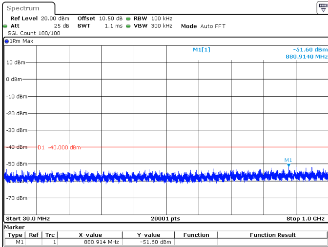
60MHz_30kHz_3670MHz_DFT-s-OFDM QPSK_RB162@0 -51.60 dBm
