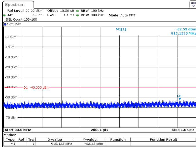
40MHz_30kHz_3680MHz_DFT-s-OFDM QPSK_RB1@105 -52.53 dBm
