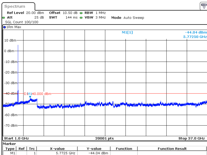
50MHz_30kHz_3675MHz_DFT-s-OFDM QPSK_RB1@0 -44.04 dBm
