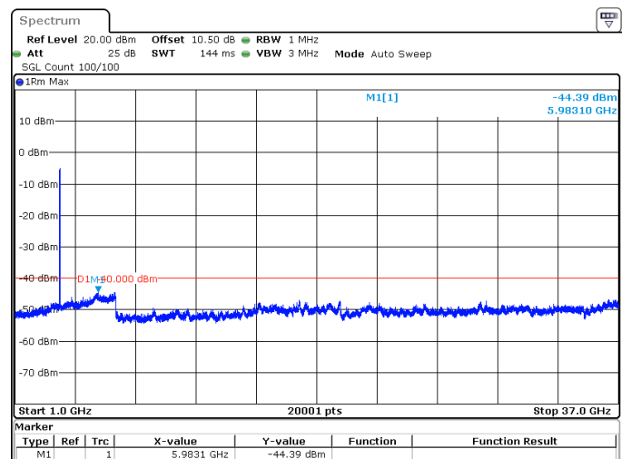
50MHz_15kHz_3675MHz_DFT-s-OFDM QPSK_RB270@0 -44.39 dBm
