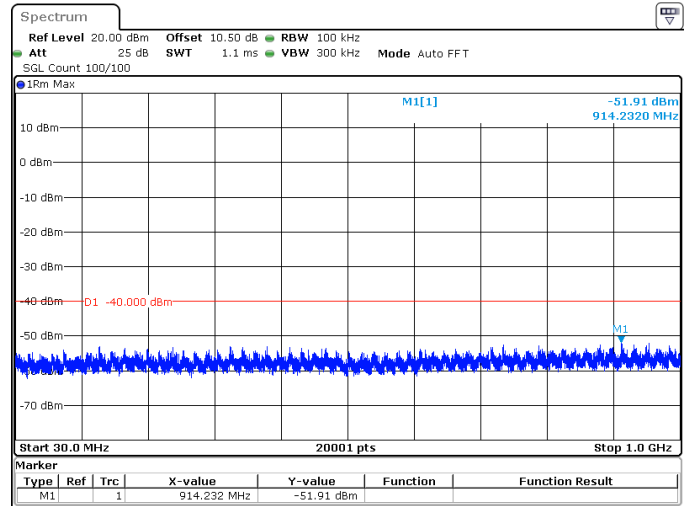
20MHz_30kHz_3625MHz_DFT-s-OFDM QPSK_RB1@0 -51.91 dBm
