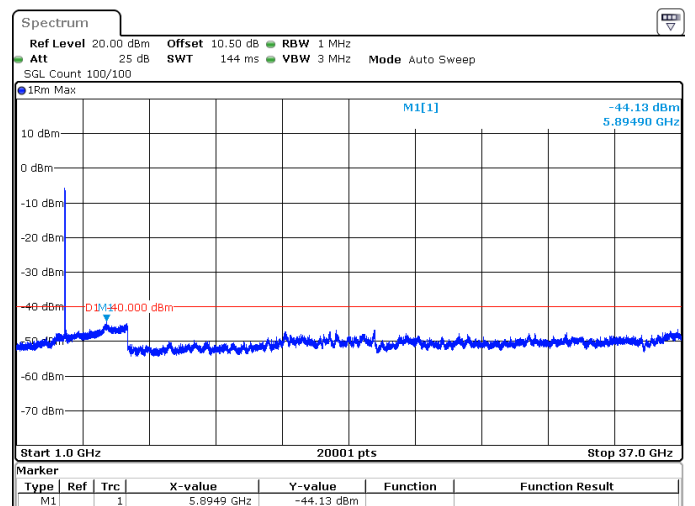
70MHz_30kHz_3625MHz_DFT-s-OFDM QPSK_RB180@0 -44.13 dBm
