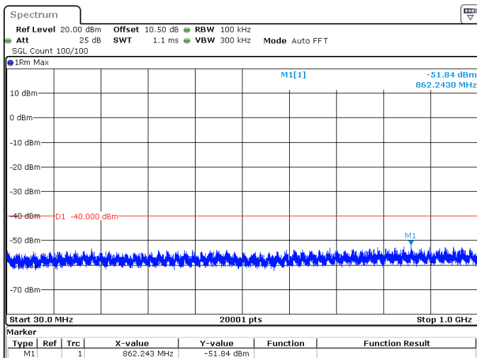
60MHz_30kHz_3670MHz_DFT-s-OFDM QPSK_RB1@0 -51.84 dBm
