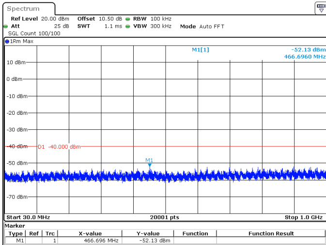
15MHz_30kHz_3692.5MHz_DFT-s-OFDM QPSK_RB1@0 -52.13 dBm
