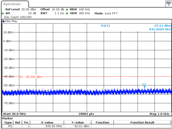
40MHz_30kHz_3680MHz_DFT-s-OFDM QPSK_RB1@0 -52.61 dBm
