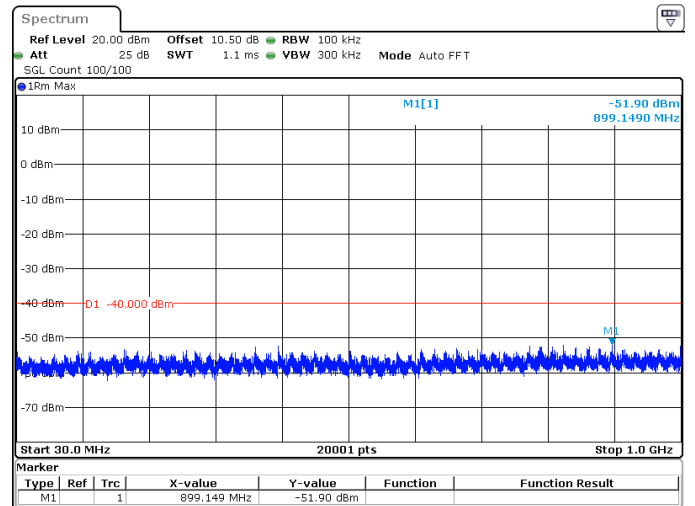
70MHz_30kHz_3665MHz_DFT-s-OFDM QPSK_RB1@0 -51.90 dBm
