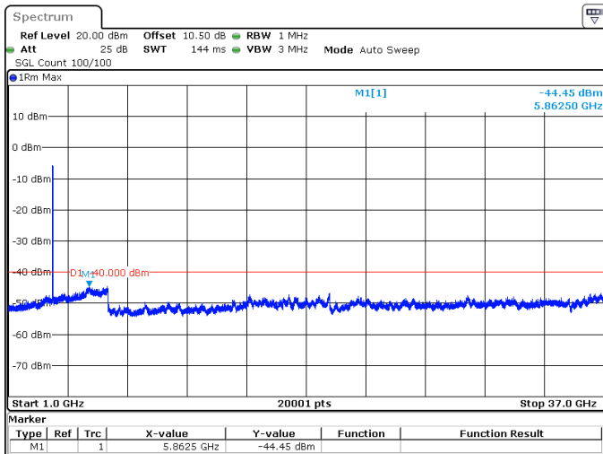
50MHz_30kHz_3675MHz_DFT-s-OFDM QPSK_RB128@0 -44.45 dBm
