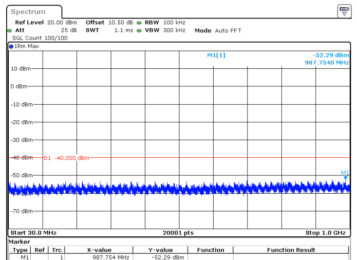
70MHz_30kHz_3665MHz_DFT-s-OFDM QPSK_RB180@0 -52.29 dBm
