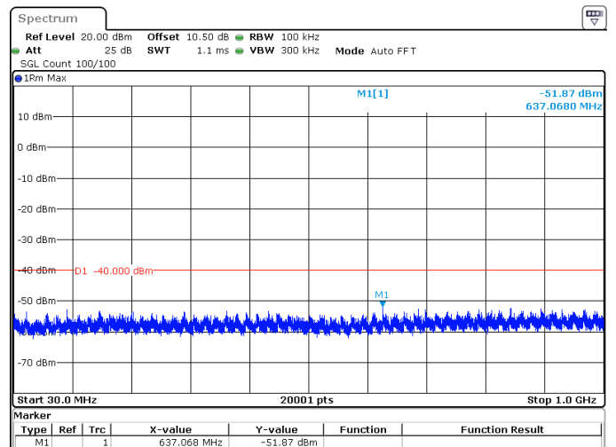
20MHz_30kHz_3625MHz_DFT-s-OFDM QPSK_RB50@0 -51.87 dBm
