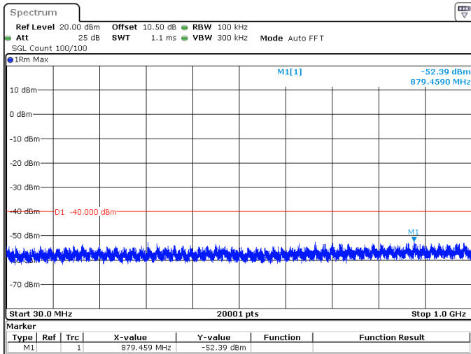
40MHz_15kHz_3625MHz_DFT-s-OFDM QPSK_RB1@0 -52.39 dBm
