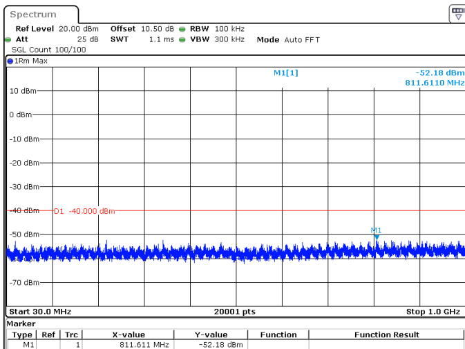
80MHz_30kHz_3590MHz_DFT-s-OFDM QPSK_RB1@0 -52.18 dBm
