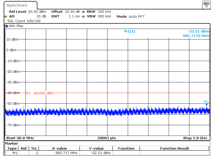
20MHz_15kHz_3690MHz_DFT-s-OFDM QPSK_RB1@0 -52.21 dBm
