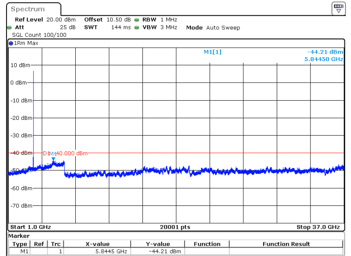
20MHz_15kHz_3690MHz_DFT-s-OFDM QPSK_RB1@105 -44.21 dBm
