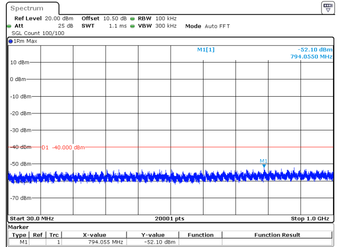
20MHz_15kHz_3560MHz_DFT-s-OFDM QPSK_RB1@0 -52.10 dBm
