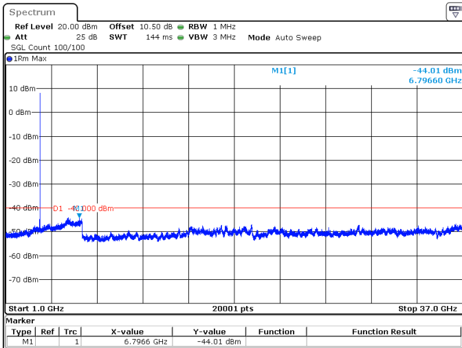
20MHz_15kHz_3690MHz_DFT-s-OFDM QPSK_RB1@0 -44.01 dBm
