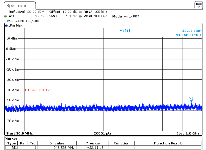
20MHz_15kHz_3625MHz_DFT-s-OFDM QPSK_RB1@0 -52.11 dBm
