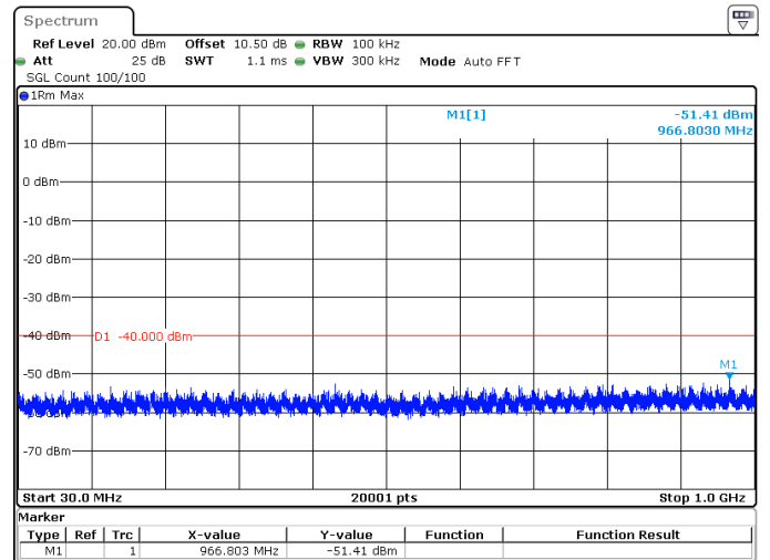
50MHz_30kHz_3675MHz_DFT-s-OFDM QPSK_RB1@0 -51.41 dBm
