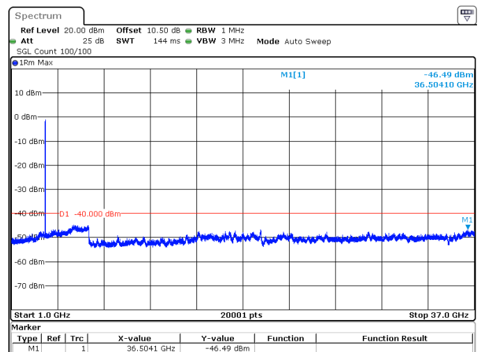
20MHz_15kHz_3625MHz_DFT-s-OFDM QPSK_RB100@0 -46.49 dBm
