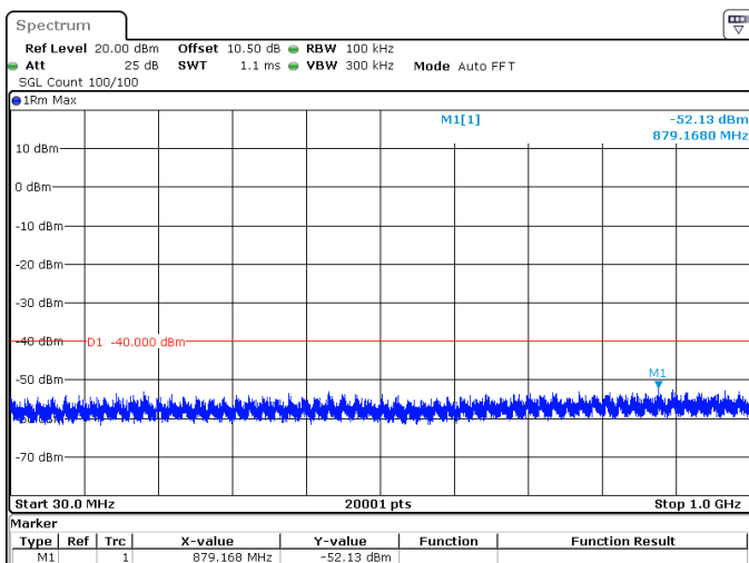
70MHz_30kHz_3665MHz_DFT-s-OFDM QPSK_RB1@188 -52.13 dBm
