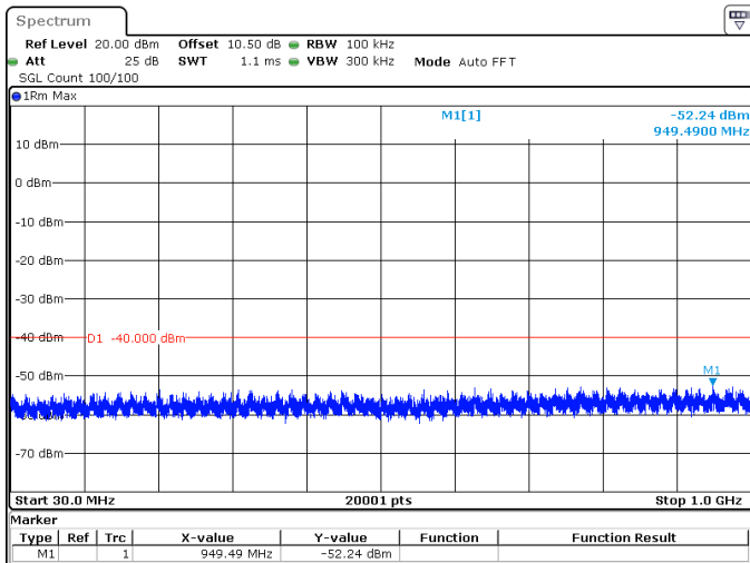
50MHz_15kHz_3625MHz_DFT-s-OFDM QPSK_RB270@0 -52.24 dBm
