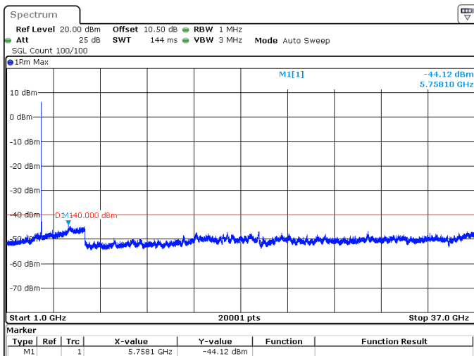
70MHz_30kHz_3665MHz_DFT-s-OFDM QPSK_RB1@0 -44.12 dBm
