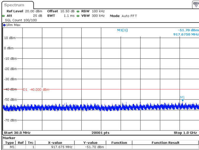
60MHz_30kHz_3580MHz_DFT-s-OFDM QPSK_RB162@0 -51.70 dBm
