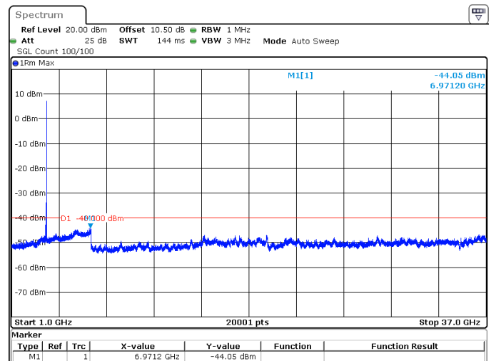
80MHz_30kHz_3590MHz_DFT-s-OFDM QPSK_RB1@216 -44.05 dBm
