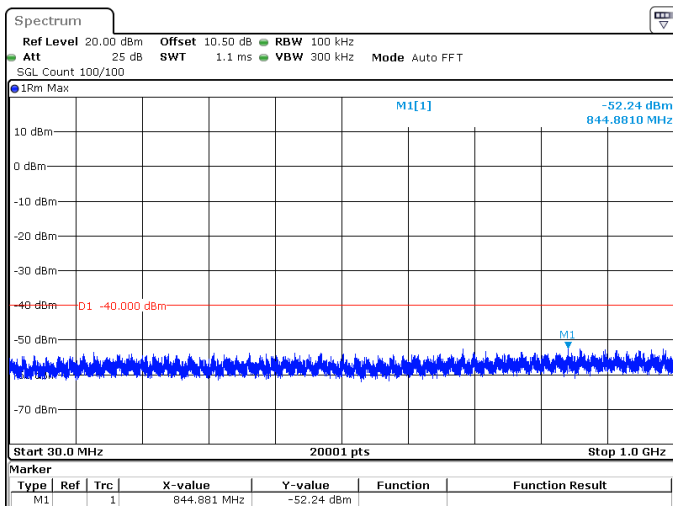
20MHz_30kHz_3560MHz_DFT-s-OFDM QPSK_RB1@0 -52.24 dBm
