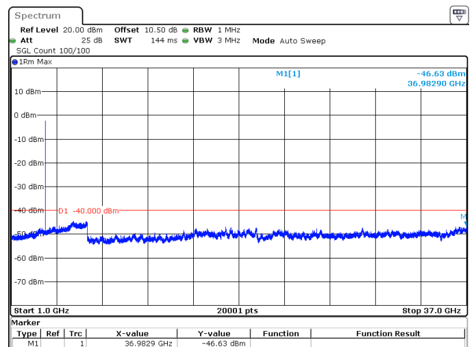
20MHz_30kHz_3690MHz_DFT-s-OFDM QPSK_RB50@0 -46.63 dBm
