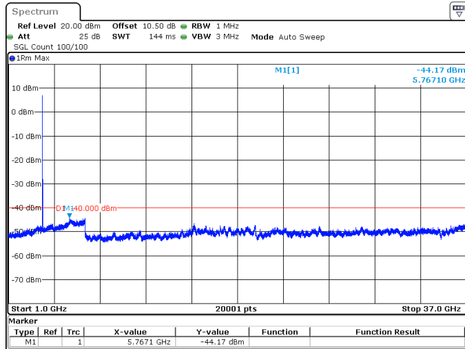
40MHz_30kHz_3680MHz_DFT-s-OFDM QPSK_RB1@0 -44.17 dBm
