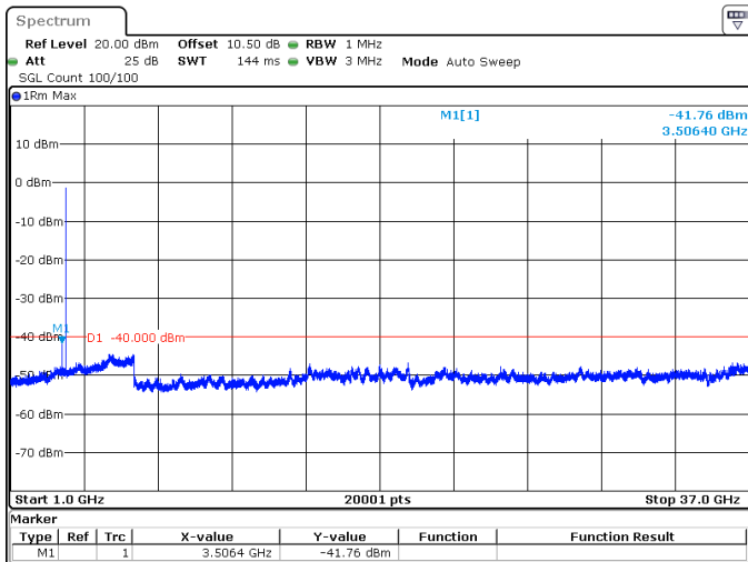
20MHz_15kHz_3690MHz_DFT-s-OFDM QPSK_RB100@0 -41.76 dBm
