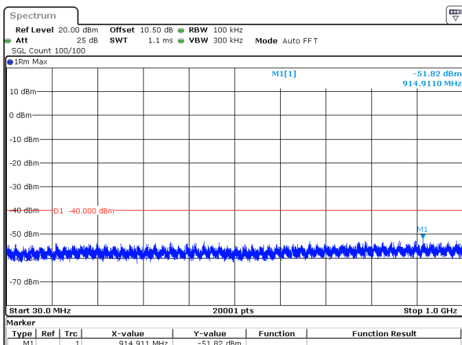
20MHz_30kHz_3560MHz_DFT-s-OFDM QPSK_RB1@50 -51.82 dBm
