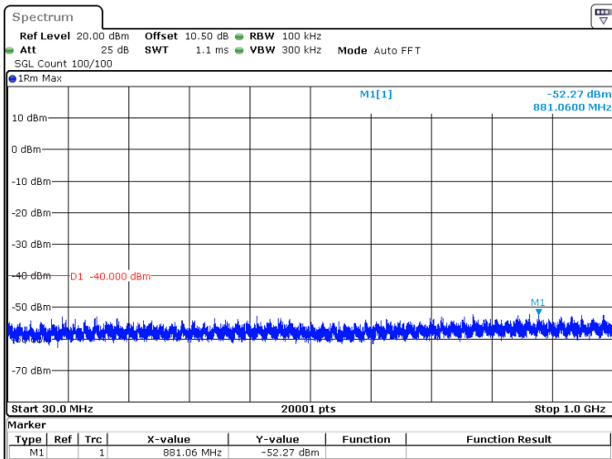
20MHz_15kHz_3690MHz_DFT-s-OFDM QPSK_RB1@105 -52.27 dBm
