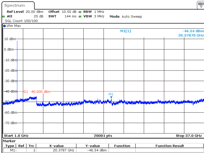
20MHz_15kHz_3560MHz_DFT-s-OFDM QPSK_RB1@0 -46.54 dBm
