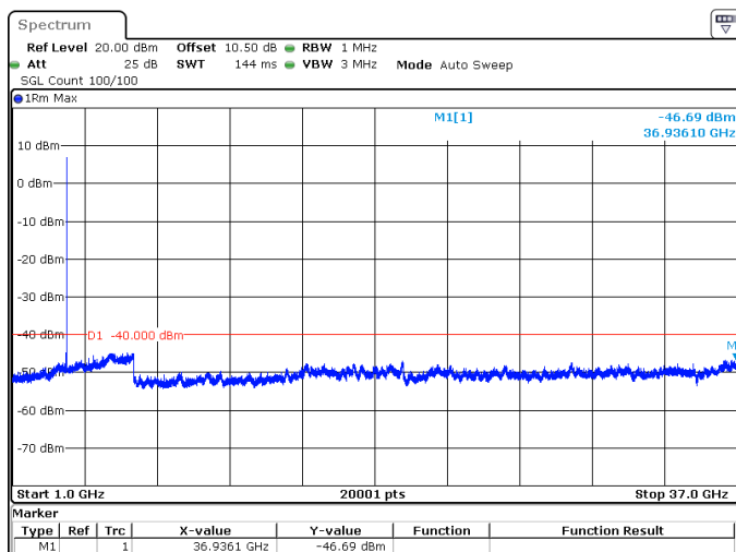
20MHz_30kHz_3690MHz_DFT-s-OFDM QPSK_RB1@50 -46.69 dBm
