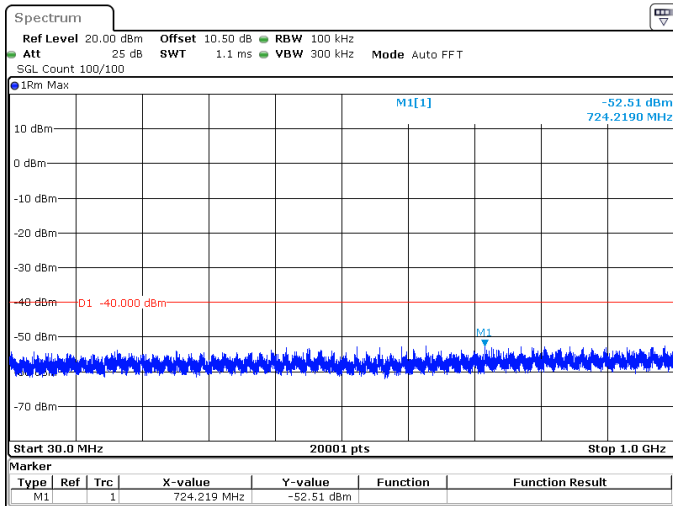
40MHz_15kHz_3680MHz_DFT-s-OFDM QPSK_RB1@0 -52.51 dBm
