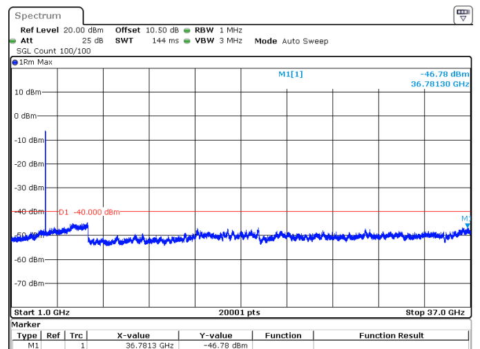
60MHz_30kHz_3670MHz_DFT-s-OFDM QPSK_RB162@0 -46.78 dBm
