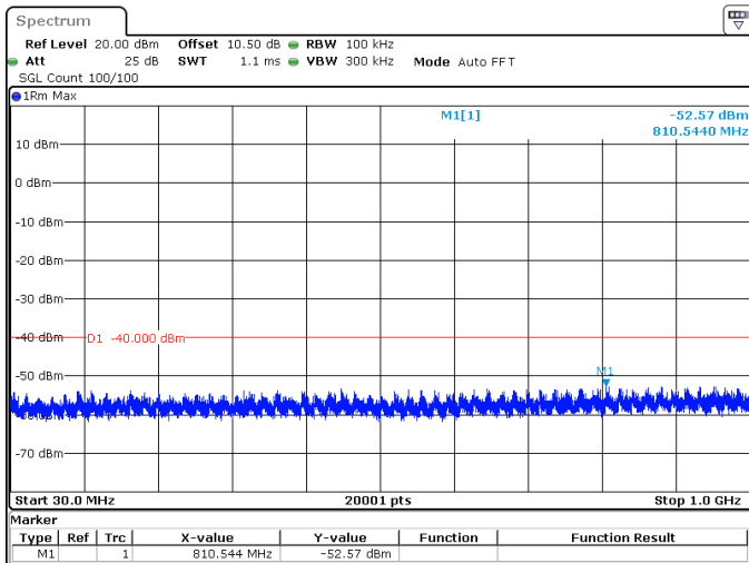
60MHz_30kHz_3625MHz_DFT-s-OFDM QPSK_RB162@0 -52.57 dBm
