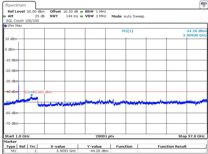
50MHz_30kHz_3625MHz_DFT-s-OFDM QPSK_RB1@0 -44.26 dBm
