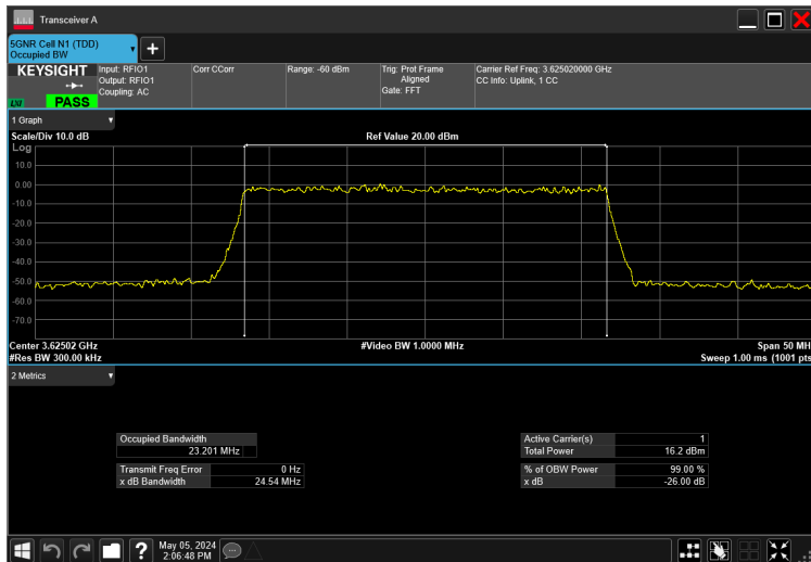
25MHz_30kHz_3625MHz_CP-OFDM QPSK_RB65@0 23.201 MHz
