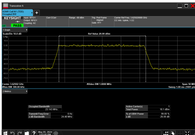
25MHz_30kHz_3625MHz_DFT-s-OFDM QPSK_RB64@0 23.143 MHz
