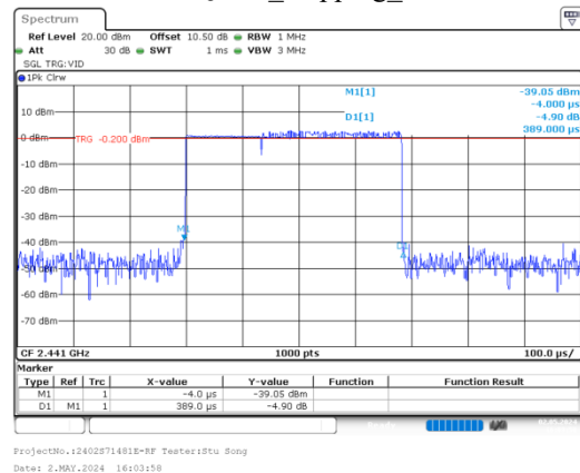
\pi/4 -DQPSK_Hopping_2DH1
