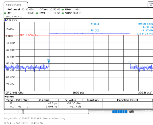
GFSK_Hopping_DH3
