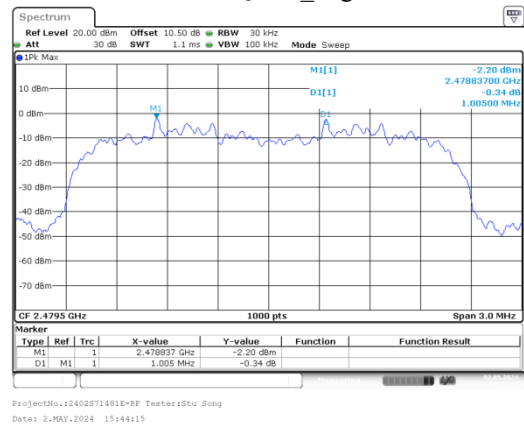
\pi/4 -DQPSK_High
