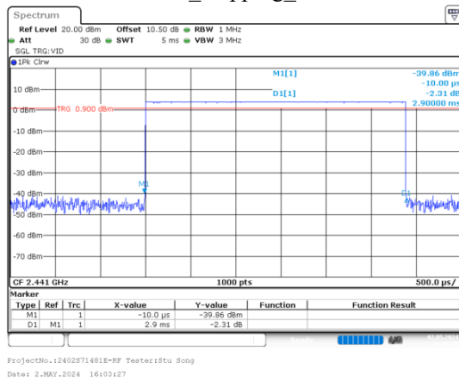
GFSK_Hopping_DH5
