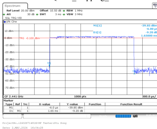
\pi/4 -DQPSK_Hopping_2DH3
