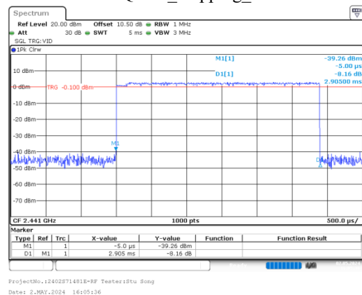
\pi/4 -DQPSK_Hopping_2DH5
