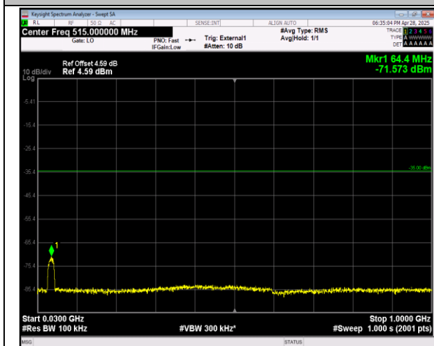
41(2555-2655)-41(2555-2655)-20MHz-20MHz-16QAM-16 QAM-40942-41140-1RB#0-0RB#0-30~1000MHz-PASS
