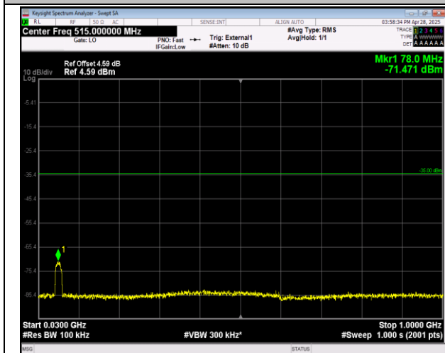
41(2555-2655)-41(2555-2655)-20MHz-5MHz-16QAM-16 QAM-41090-41207-1RB#0-0RB#0-30~1000MHz-PASS
