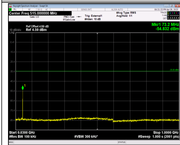
41(2555-2655)-41(2555-2655)-20MHz-20MHz-QPSK-QP SK-40942-41140-100RB#0-100RB#0-30~1000MHz-PASS
