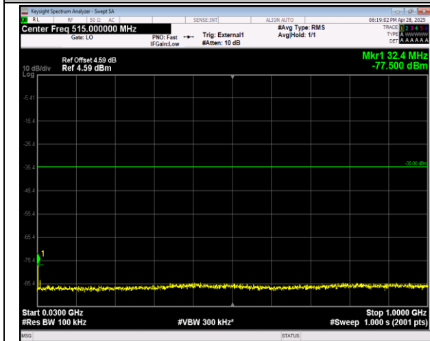
41(2555-2655)-41(2555-2655)-20MHz-20MHz-QPSK-QP SK-40340-40538-1RB#99-ORB#0-30~1000MHz-PASS
