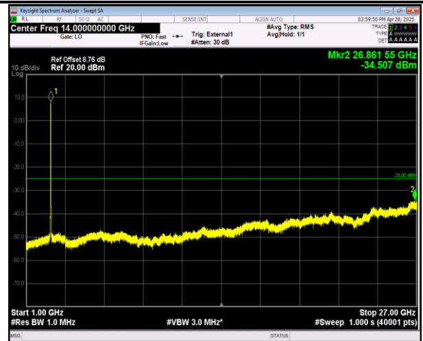
41(2555-2655)-41(2555-2655)-20MHz-20MHz-QPSK-QPS K-40340-40538-1RB#0-ORB#0-1000~27000MHz-PASS
