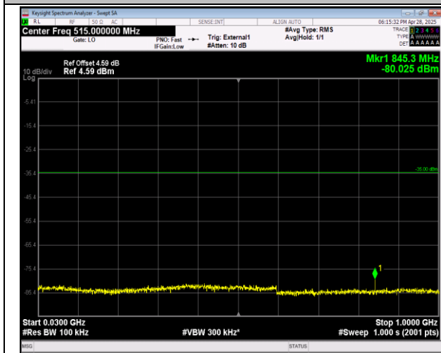
41(2555-2655)-41(2555-2655)-20MHz-20MHz-QPSK-QP SK-40340-40538-1RB#0-1RB#99-30~1000MHz-PASS
