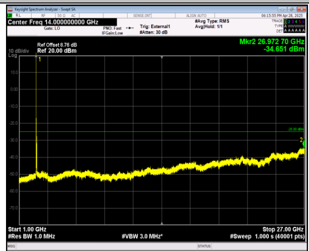
41(2555-2655)-41(2555-2655)-20MHz-20MHz-QPSK-QPS K-40340-40538-1RB#0-1RB#99-1000~27000MHz-PASS
