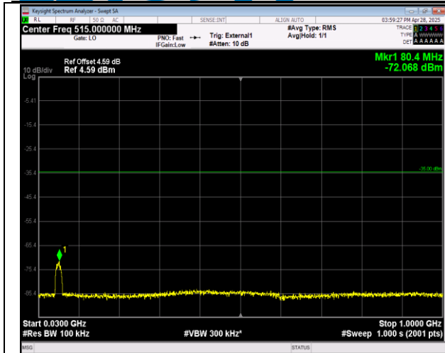
41(2555-2655)-41(2555-2655)-20MHz-20MHz-QPSK-QP SK-40340-40538-1RB#0-ORB#0-30~1000MHz-PASS
