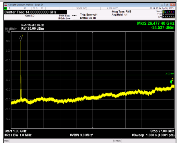
41(2555-2655)-41(2555-2655)-20MHz-20MHz-QPSK-QPS K-40340-40538-1RB#99-ORB#0-1000~27000MHz-PASS
