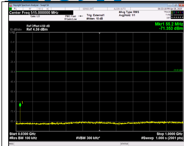
41(2555-2655)-41(2555-2655)-20MHz-20MHz-QPSK-QP SK-40942-41140-1RB#99-0RB#0-30~1000MHz-PASS
