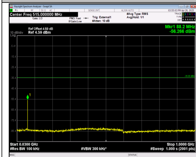
41(2555-2655)-41(2555-2655)-20MHz-5MHz-QPSK-QPS K-41090-41207-100RB#0-25RB#0-30~1000MHz-PASS
