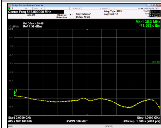
41(2555-2655)-41(2555-2655)-5MHz-20MHz-16QAM-16 QAM-40273-40390-1RB#0-0RB#0-30~1000MHz-PASS
