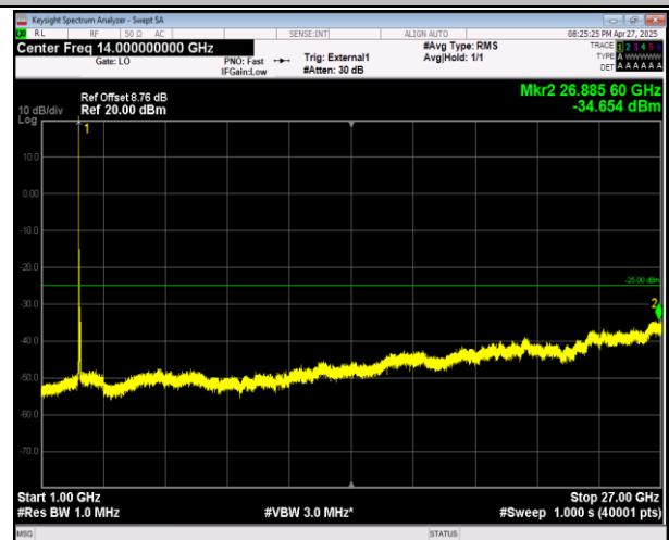
38-38-20MHz-20MHz-QPSK-QPSK-37952-38150-1RB#0-1 RB#99-1000~27000MHz-PASS
