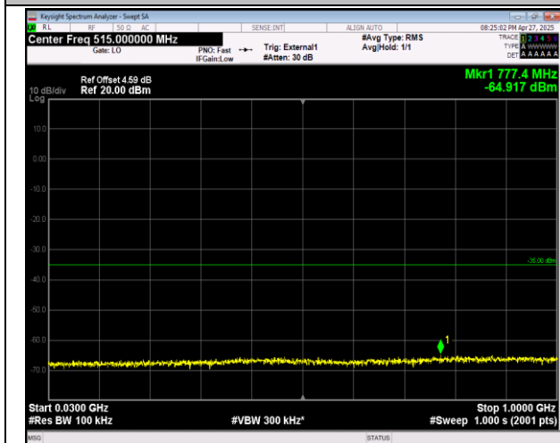
38-38-20MHz-20MHz-QPSK-QPSK-37952-38150-1RB#0- 1RB#99-30~1000MHz-PASS
