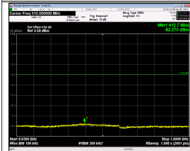
41(2555-2655)-41(2555-2655)-5MHz-20MHz-16QAM-16 QAM-40273-40390-1RB#0-1RB#99-30~1000MHz-PASS
