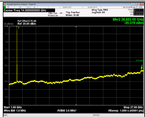
7-7-20MHz-20MHz-QPSK-QPSK-21152-21350-1RB#0-1RB #99-1000~27000MHz-PASS
