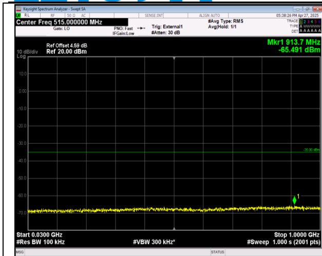
38-38-20MHz-20MHz-QPSK-QPSK-37850-38048-1RB#0-ORB#0-30~1000MHz-PASS
