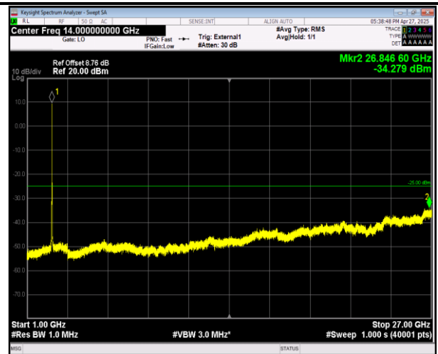
38-38-20MHz-20MHz-QPSK-QPSK-37850-38048-1RB#0-0RB#0-1000~27000MHz-PASS
