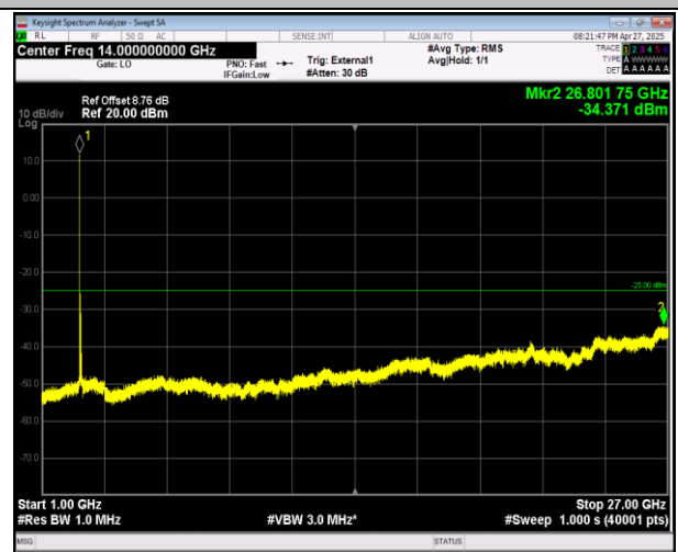
38-38-20MHz-20MHz-QPSK-QPSK-37901-38099-1RB#99-9-0RB#0-1000~27000MHz-PASS
