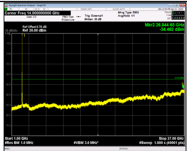
38-38-20MHz-20MHz-QPSK-QPSK-37850-38048-100RB#0 -100RB#0-1000~27000MHz-PASS
