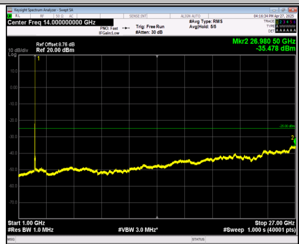
7-7-20MHz-20MHz-QPSK-QPSK-21152-21350-100RB#0-1 00RB#0-1000~27000MHz-PASS
