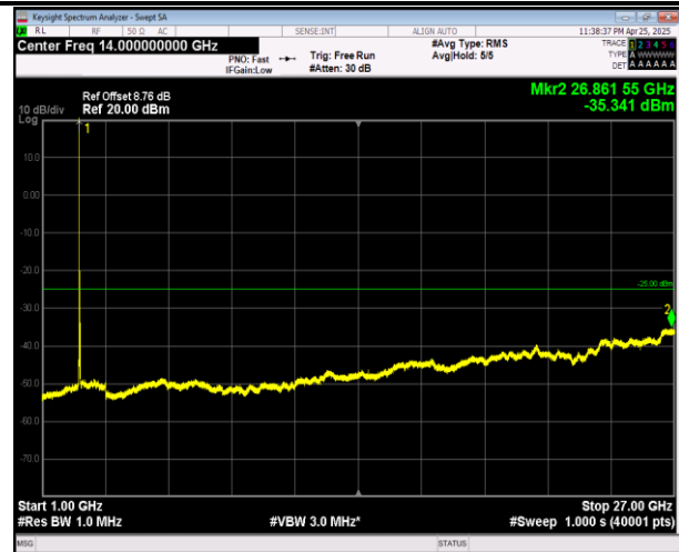
7-7-20MHz-10MHz-QPSK-QPSK-21051-21195-1RB#0-1RB #49-1000~27000MHz-PASS
