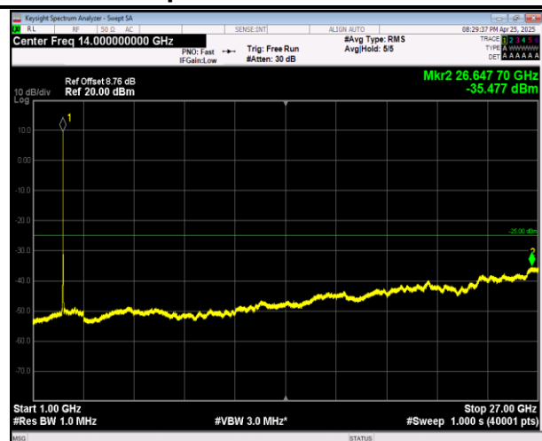
7-7-20MHz-10MHz-QPSK-QPSK-20850-20994-1RB#0-0RB #0-1000~27000MHz-PASS
