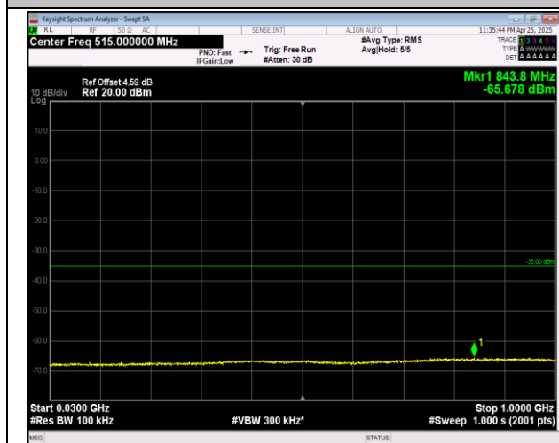
7-7-20MHz-10MHz-QPSK-QPSK-20850-20994-1RB#99-0 RB#0-30~1000MHz-PASS
