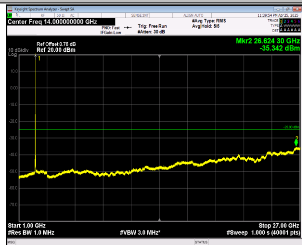
7-7-20MHz-10MHz-QPSK-QPSK-21051-21195-100RB#0-5 ORB#0-1000~27000MHz-PASS
