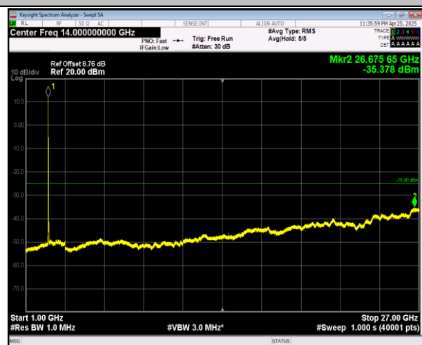
7-7-20MHz-10MHz-QPSK-QPSK-20850-20994-1RB#99-0RB B#0-1000~27000MHz-PASS
