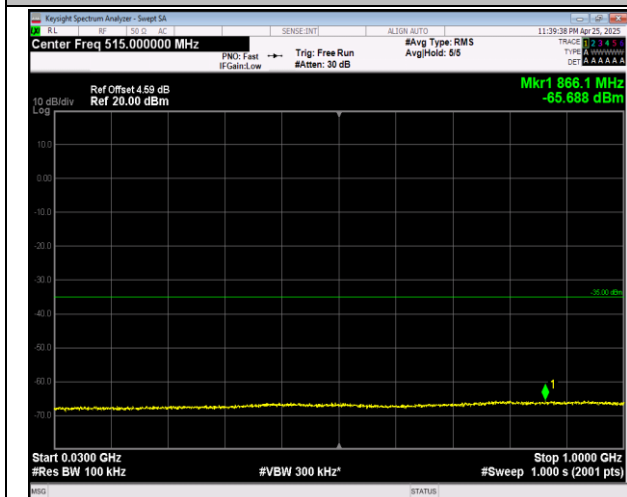
7-7-20MHz-10MHz-QPSK-QPSK-21051-21195-100RB#0- 50RB#0-30~1000MHz-PASS
