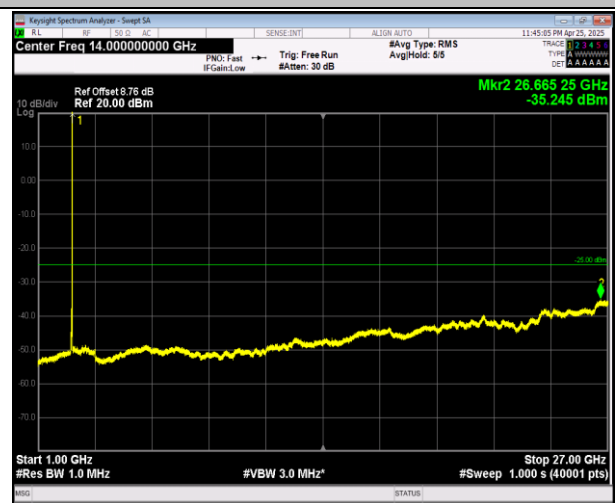
7-7-20MHz-10MHz-QPSK-QPSK-21251-21395-100RB#0-50RB#0-30~1000MHz-PASS ORB#0-1000~27000MHz-PASS
