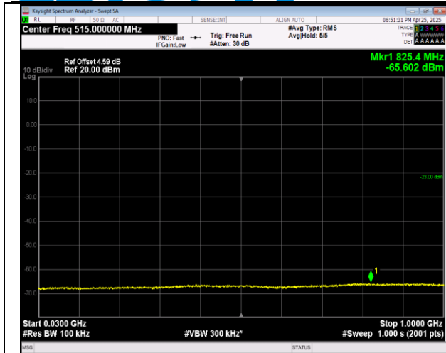
2-2-20MHz-20MHz-QPSK-QPSK-18700-18898-100RB#0-100RB#0-30~1000MHz-PASS
