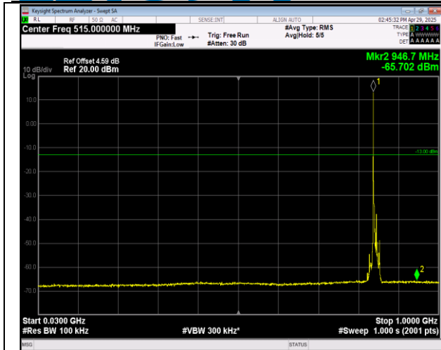
5-5-3MHz-5MHz-QPSK-QPSK-20586-20625-1RB#14-0R B#0-30~1000MHz-PASS
