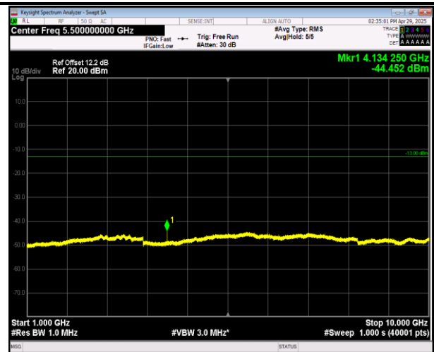
5-5-3MHz-5MHz-QPSK-QPSK-20416-20455-15RB#0-25RB #0-1000~10000MHz-PASS
