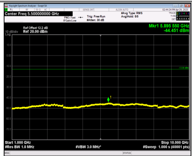
5-5-3MHz-5MHz-QPSK-QPSK-20586-20625-15RB#0-25RB #0-1000~10000MHz-PASS
