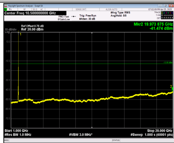
2-2-20MHz-20MHz-QPSK-QPSK-18902-19100-100RB#0-1 00RB#0-1000~20000MHz-PASS
