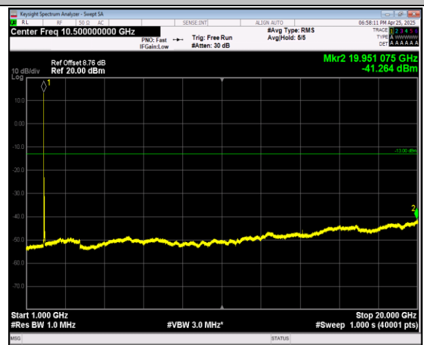
2-2-20MHz-20MHz-QPSK-QPSK-18801-18999-1RB#99-0R B#0-1000~20000MHz-PASS
