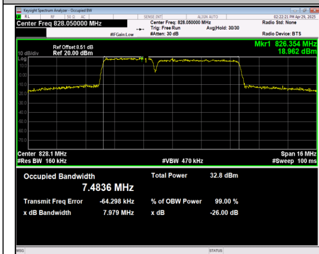
5-5-3MHz-5MHz-QPSK-QPSK-20501-20540-15RB#0-25 RB#0-PASS
