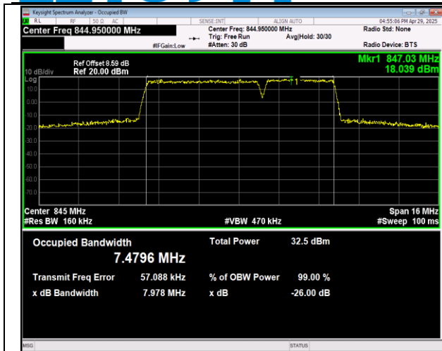
5-5-5MHz-10MHz-QPSK-QPSK-20428-20500-25RB#0-50 RB#0-PASS
