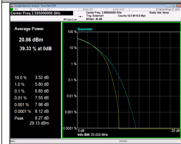
41(2555-2655)-41(2555-2655)-20MHz-20MHz-QPSK-QPS-40641-40839-100RB#0-100RB#0-PASS
