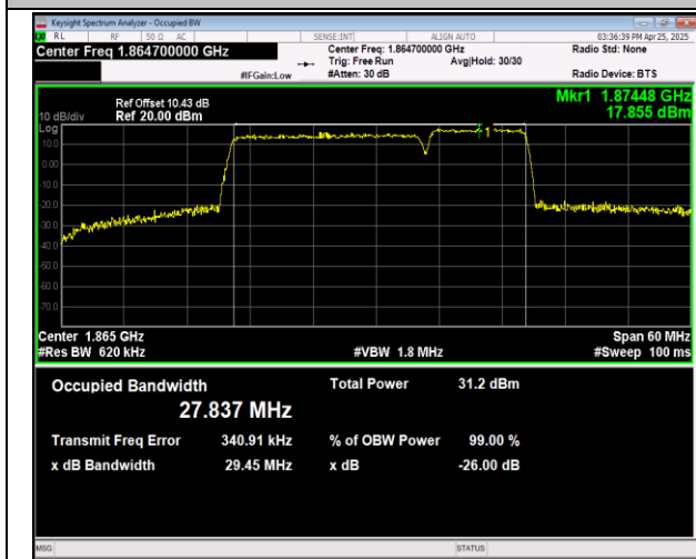
2-2-20MHz-10MHz-QPSK-QPSK-1864-1864-100RB#0-50RB#0-PASS
