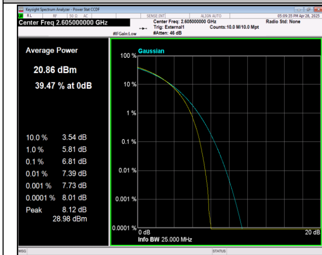
41(2555-2655)-41(2555-2655)-20MHz-20MHz-QPSK-QPS-40641-40839-100RB#0-100RB#0-PASS
