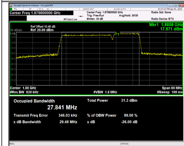
2-2-20MHz-10MHz-QPSK-QPSK-1879-1879-100RB#0-50RB#0-PASS
