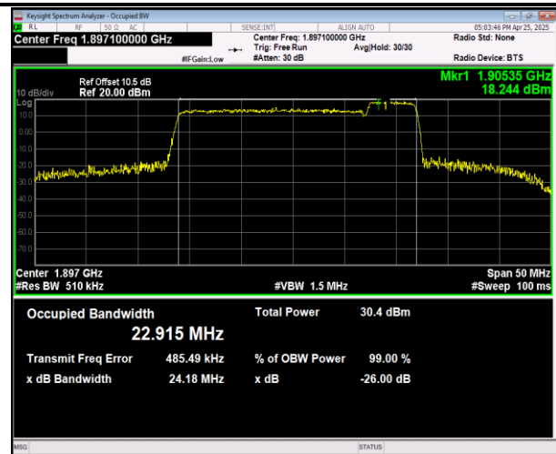
2-2-20MHz-10MHz-16QAM-16QAM-1897-1897-100RB#0-50RB#0-PASS
