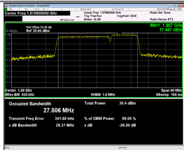
2-2-20MHz-10MHz-16QAM-16QAM-1879-1879-100RB#0-50RB#0-PASS
