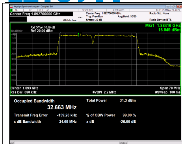
2-2-20MHz-5MHz-QPSK-QPSK-18700-18817-100RB#0-2 5RB#0-PASS
