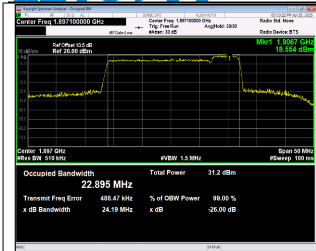
2-2-20MHz-10MHz-QPSK-QPSK-1897-1897-100RB#0-50RB#0-PASS
