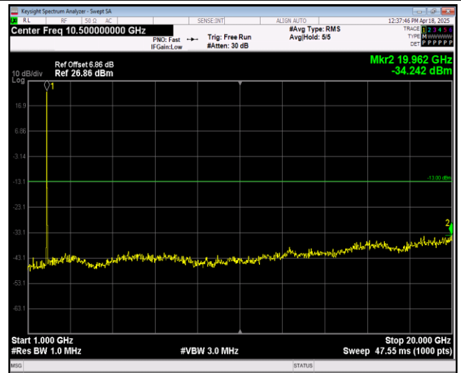
Band2-20MHz-64QAM-18900-1RB#0-Range2:1000~20000MHz
