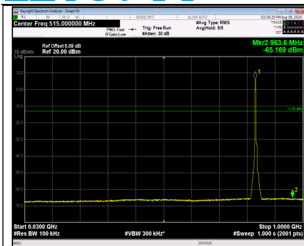
5-5-3MHz-5MHz-QPSK-QPSK-20501-20540-15RB#0-25 RB#0-30~1000MHz-PASS
