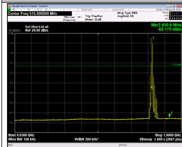
5-5-5MHz-3MHz-QPSK-QPSK-20425-20464-1RB#0-1R B#15-30~1000MHz-PASS
