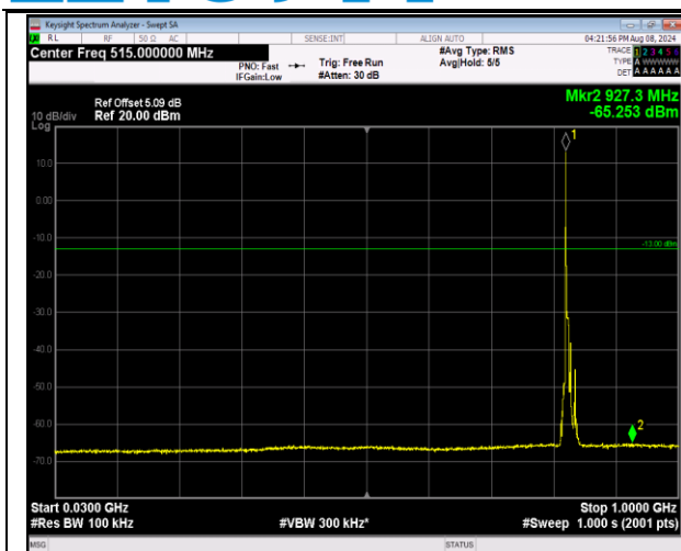
5-5-5MHz-3MHz-QPSK-QPSK-20425-20464-1RB#0-0R B#0-30~1000MHz-PASS
