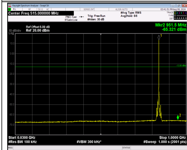
5-5-3MHz-5MHz-QPSK-QPSK-20586-20625-1RB#14-0R B#0-30~1000MHz-PASS
