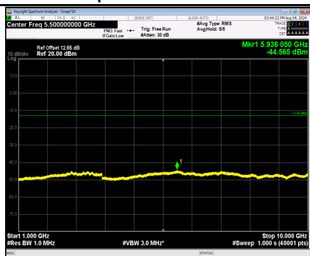
5-5-3MHz-5MHz-QPSK-QPSK-20586-20625-15RB#0-25 RB#0-1000~10000MHz-PASS
