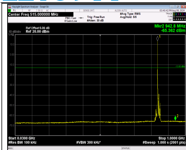
5-5-3MHz-5MHz-QPSK-QPSK-20586-20625-1RB#0-0R B#0-30~1000MHz-PASS
