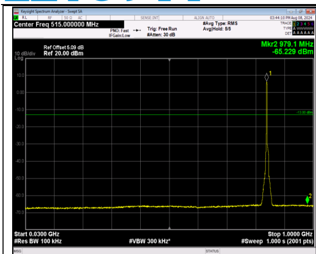
5-5-3MHz-5MHz-QPSK-QPSK-20586-20625-15RB#0-25 RB#0-30~1000MHz-PASS
