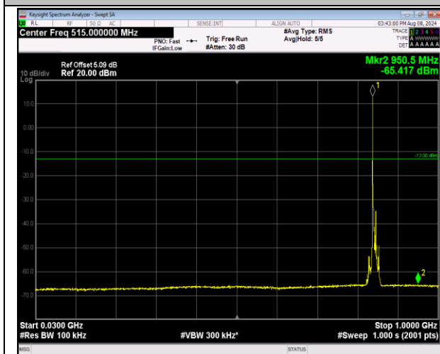
5-5-3MHz-5MHz-QPSK-QPSK-20586-20625-1RB#0-1R B#24-30~1000MHz-PASS
