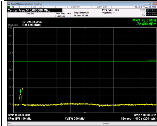
41-41-20MHz-5MHz-QPSK-QPSK-41090-41207-100RB# 0-25RB#0-30-1000MHz-PASS
