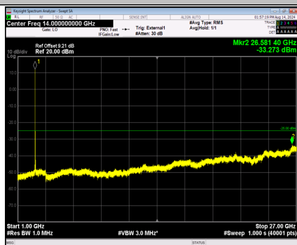
41-41-20MHz-5MHz-QPSK-QPSK-41090-41207-1RB#0-0RB#24-1000~27000MHz-PASS
