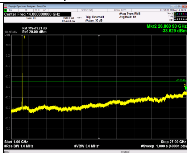
41-41-20MHz-5MHz-QPSK-QPSK-41090-41207-1RB#0-0RB#0-1000~27000MHz-PASS
