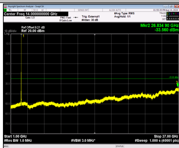
41-41-20MHz-5MHz-QPSK-QPSK-41090-41207-1RB#99-0RB#0-1000~27000MHz-PASS
