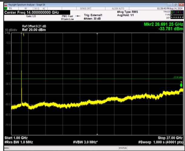
41-41-20MHz-5MHz-QPSK-QPSK-40340-40457-1RB#0-0RB#0-1000~27000MHz-PASS
