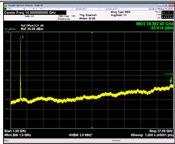
41-41-20MHz-20MHz-QPSK-QPSK-40340-40538-1RB#0-1 RB#99-1000~27000MHz-PASS
