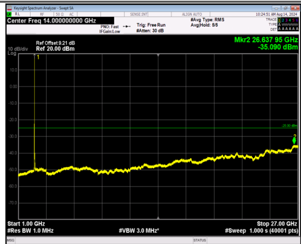
7-7-20MHz-10MHz-QPSK-QPSK-20850-20994-1RB#99-0R B#0-1000~27000MHz-PASS
