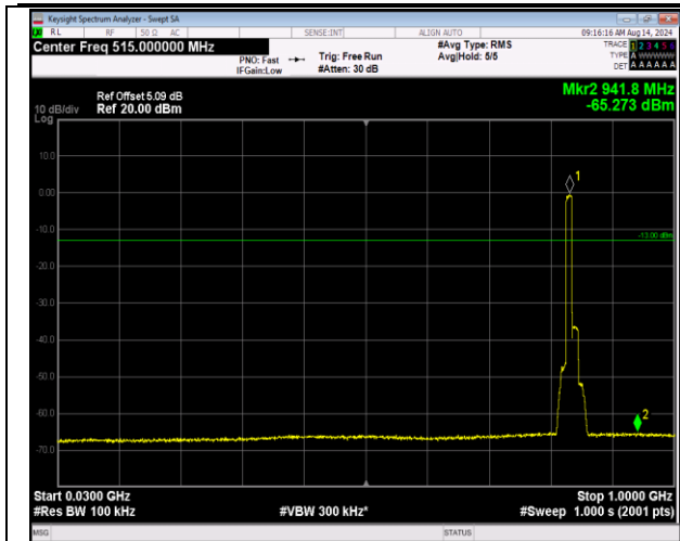
5-5-10MHz-10MHz-QPSK-QPSK-20501-20600-50RB#0-50RB#0-30~1000MHz-PASS
