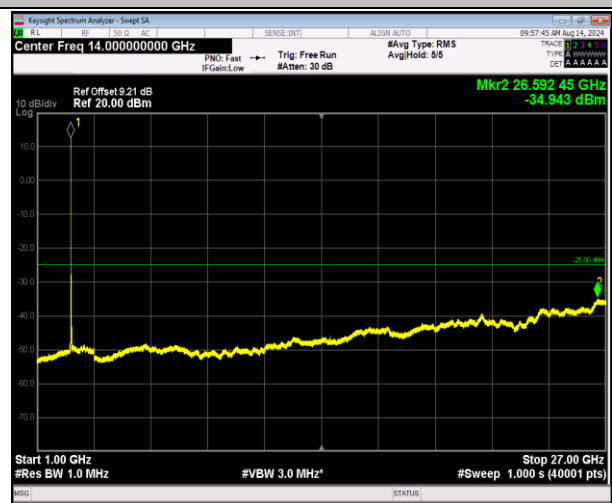
7-7-10MHz-20MHz-QPSK-QPSK-21206-21350-1RB#0-1RB #99-1000~27000MHz-PASS
