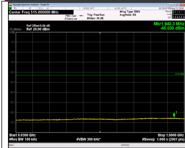
2-2-5MHz-20MHz-QPSK-QPSK-18808-18925-25RB#0-1 00RB#0-30~1000MHz-PASS
