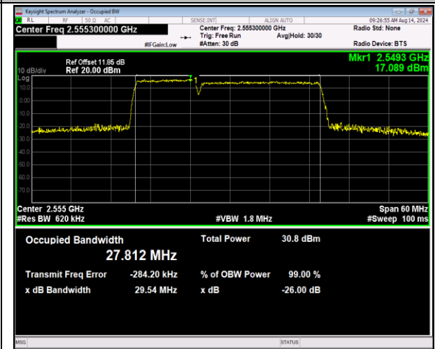
7-7-10MHz-20MHz-QPSK-QPSK-21206-21350-50RB#0- 100RB#0-PASS
