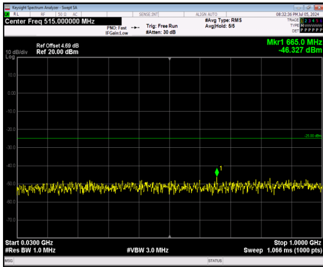
Band41-5MHz-QPSK-41215-1RB#0-Range1:30~100 OMHz
