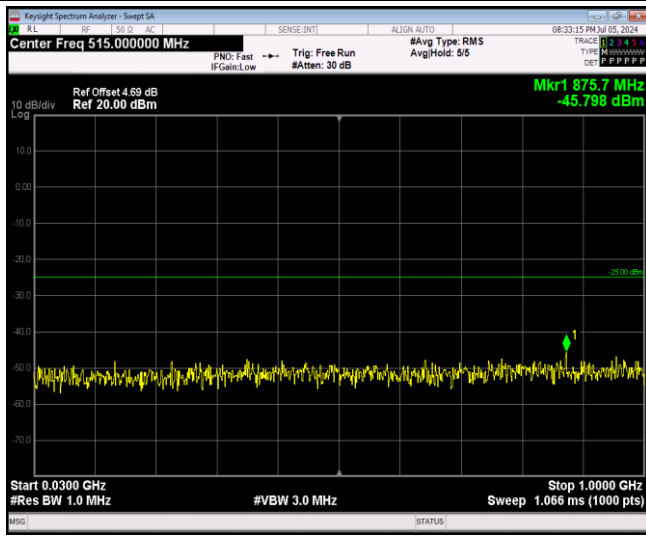
Band41-5MHz-QPSK-41215-1RB#0-Range1:30~100 OMHz
