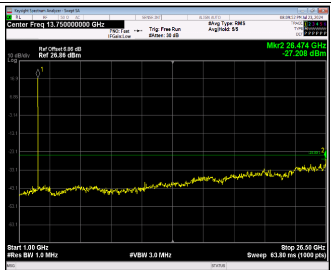
Band7-20MHz-QPSK-20850-1RB#0-Range2:1000~265 00MHz
