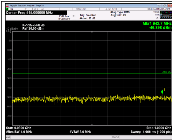
Band41-5MHz-QPSK-40640-1RB#0-Range1:30~100 OMHz
