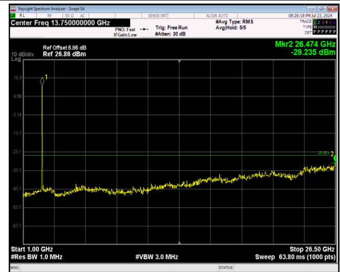
Band41-5MHz-QPSK-40065-1RB#0-Range2:1000~26500MHz
