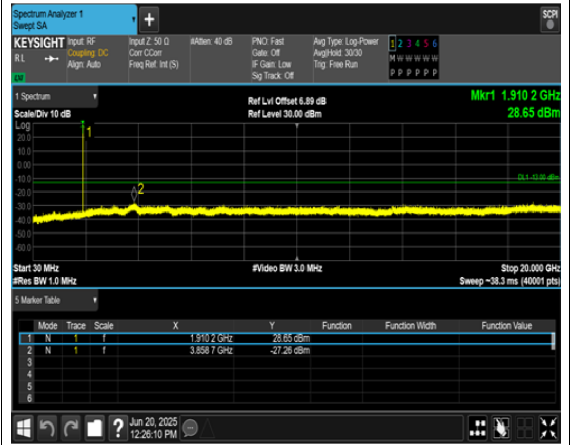
EGPRS1900 Channel=810
