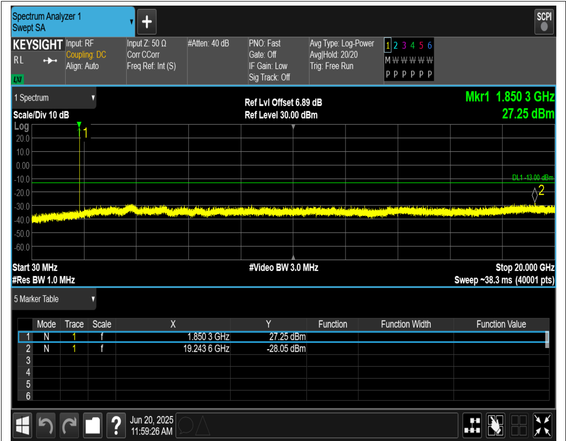
GPRS1900 Channel=512
