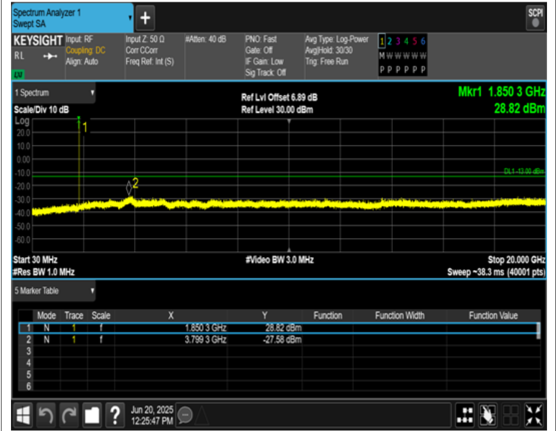
EGPRS1900 Channel=512
