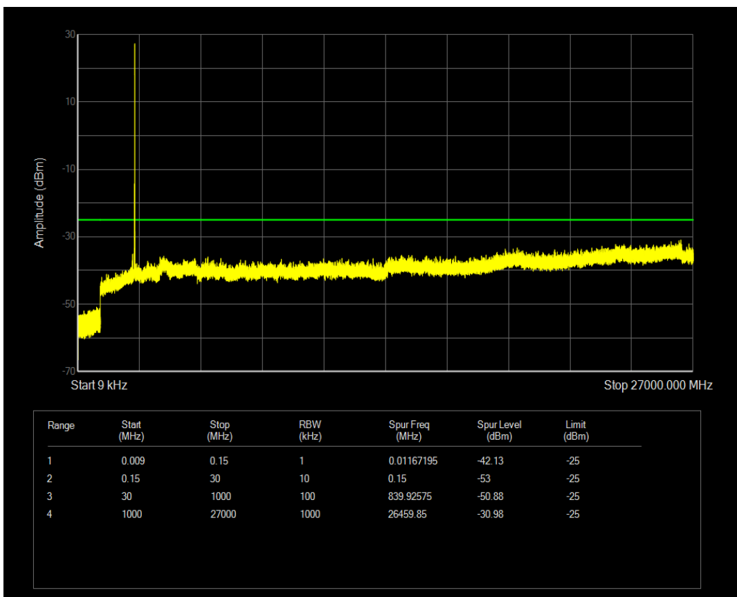
n41 SCS=30kHz CP_QPSK BW=20MHz Channel=501204 RB=51@50
