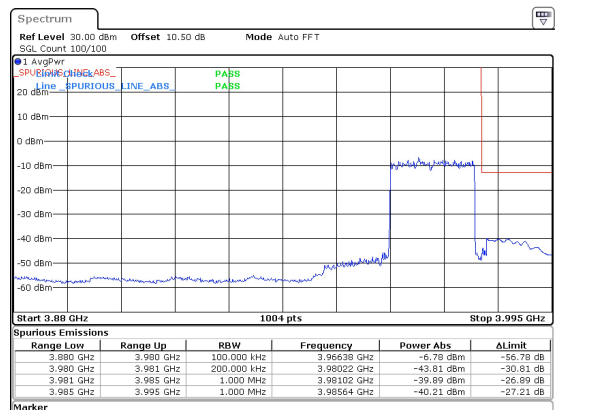
20MHz_15kHz_3970MHz_DFT-s-OFDM QPSK_RB100@0 -39.89 dBm
