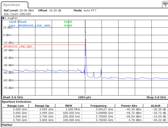
20MHz_15kHz_3710MHz_DFT-s-OFDM QPSK_RB1@0 -28.04 dBm
