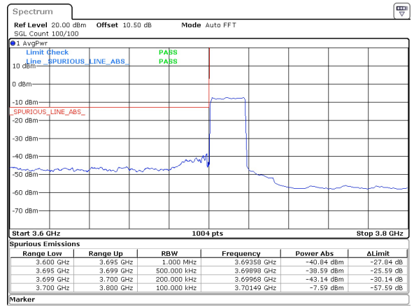
20MHz_15kHz_3710MHz_DFT-s-OFDM QPSK_RB100@0 -38.59 dBm
