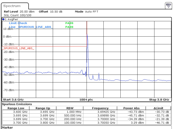
15MHz_30kHz_3707.5MHz_DFT-s-OFDM QPSK_RB1@0 -34.39 dBm
