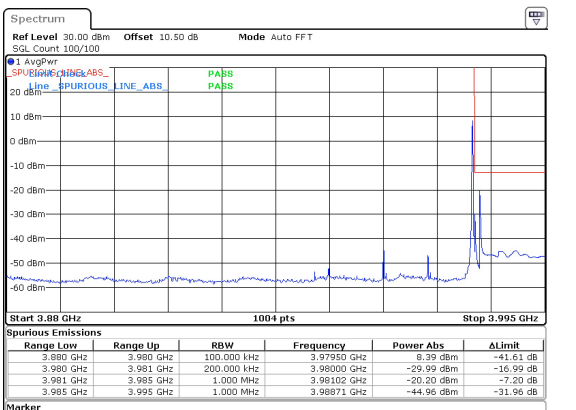
20MHz_15kHz_3970MHz_DFT-s-OFDM QPSK_RB1@105 -20.20 dBm
