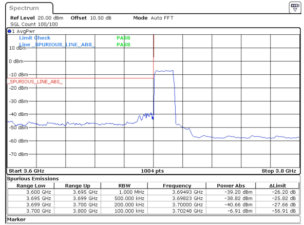
15MHz_15kHz_3707.5MHz_DFT-s-OFDM QPSK_RB75@0 -38.82 dBm
